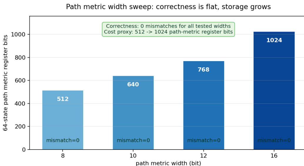
图4展示了 path metric width 对硬件代价的影响。在 depth=40 和 subtract-min normalization 条件下，当前测试集里 8/10/12/16 bit 都没有观察到 mismatch，所以图中直接在每根柱子底部标出 mismatch=0；柱高表示 64 个状态需要保存的 path metric register 总位数。位宽越大，寄存器位数从 512 增加到 1024，加法器和比较器也会变宽，资源占用和时序压力都会上升。因此，选择 12 bit 不是因为 16 bit 不正确，而是因为 12 bit 已经足够通过当前功能闭环，同时比 16 bit 更克制。
