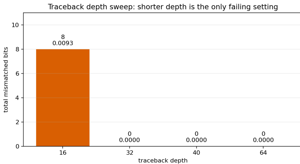
图3展示了 traceback depth 对 mismatch 数量的影响。depth=16 时，当前向量集中出现 8 个 mismatch，说明回溯深度太短时，路径还没有充分收敛，译码器可能过早做出判断。depth=32、40、64 时，当前测试向量下 mismatch 都为 0。因此，depth=40 的意义是：它已经达到当前测试条件下的 0 mismatch，同时相比 depth=64 可以减少一部分 survivor memory 需求和 traceback 等待时间。
