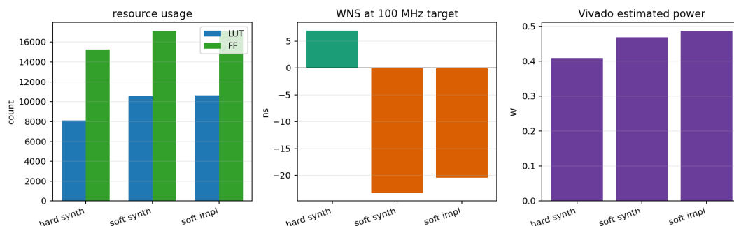
图 8：Vivado 资源、时序和功耗对比。左图比较 LUT 和 FF，中图比较 WNS，右图比较 Vivado 估算功耗。这样分开画以后可以看清楚：soft-decision 版本资源增加并不夸张，但 WNS
