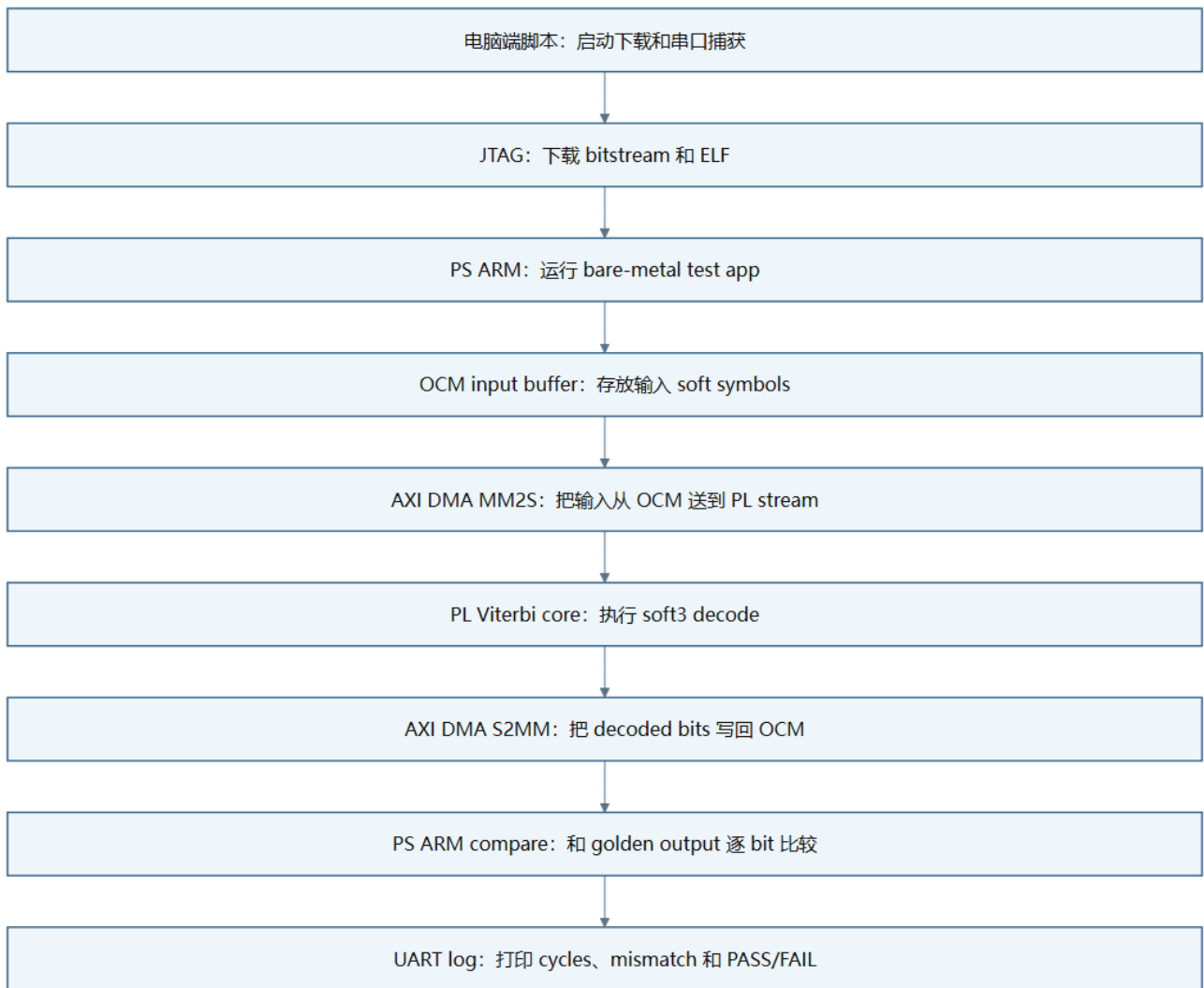
图 11：板级数据流。这张图说明一次 board validation 的完整路径：电脑启动测试，JTAG 下载，ARM 准备 OCM buffer，DMA 把输入送进 PL，Viterbi core 输出 decoded bits，DMA 写回 OCM，ARM 比对 golden output，最后 UART 打印结果。
