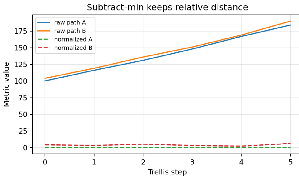
图 6 展示了 subtract-min normalization 的作用。图中每条路径的绝对 path metric 数值都被整体压低，但路径之间的相对大小没有改变。也就是说，归一化前哪条路径最优，归一化后仍然是哪条路径最优。它解决的是固定宽度硬件中的数值范围和溢出风险问题，而不是改变 Viterbi Decoder 的路径选择逻辑
