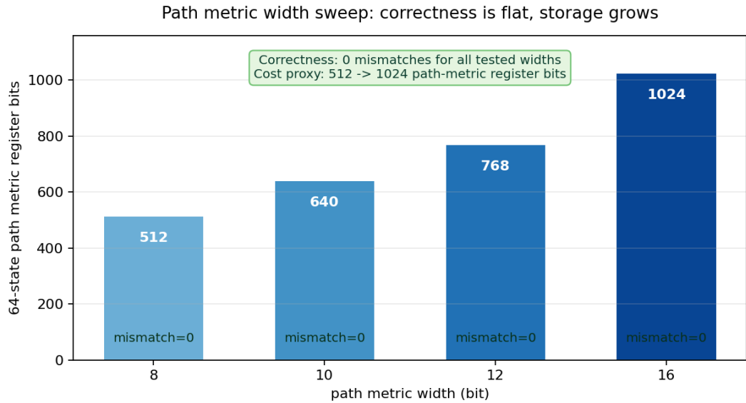
图 4 展示了 path metric width 对硬件代价的影响。在 depth=40 和 subtract-min normalization 条件下，当前测试集里 8/10/12/16 bit 都没有观察到 mismatch，所以图中直接在每根柱子底部标出 mismatch=0；柱高表示 64 个状态需要保存的 path metric register 总位数。位宽越大，寄存器位数从 512 增加到 1024，加法器和比较器也会变宽，资源占用和时序压力都会上升。因此，选择 12 bit 不是因为 16 bit 不正确，而是因为 12 bit 已经足够通过当前功能闭环，同时比 16 bit 更克制。
