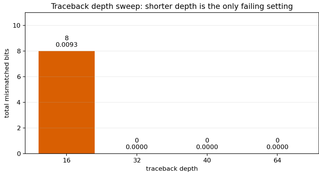
图 3 展示了 traceback depth 对 mismatch 数量的影响。depth=16 时，当前向量集中出现 8 个 mismatch，说明回溯深度太短时，路径还没有充分收敛，译码器可能过早做出判断。depth=32、40、64 时，当前测试向量下 mismatch 都为 0。因此，depth=40 的意义是：它已经达到当前测试条件下的 0 mismatch，同时相比 depth=64 可以减少一部分 survivor memory 需求和 traceback 等待时间。
