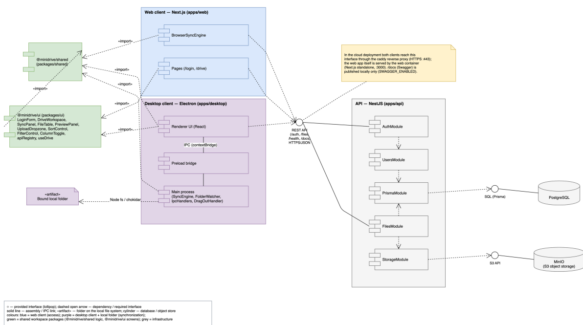
Рисунок 1. Рис. 1. Діаграма компонентів
