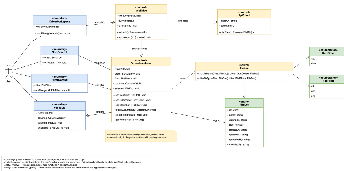
Рисунок 5. Рис. 5. VOPC для UC5 + UC6
