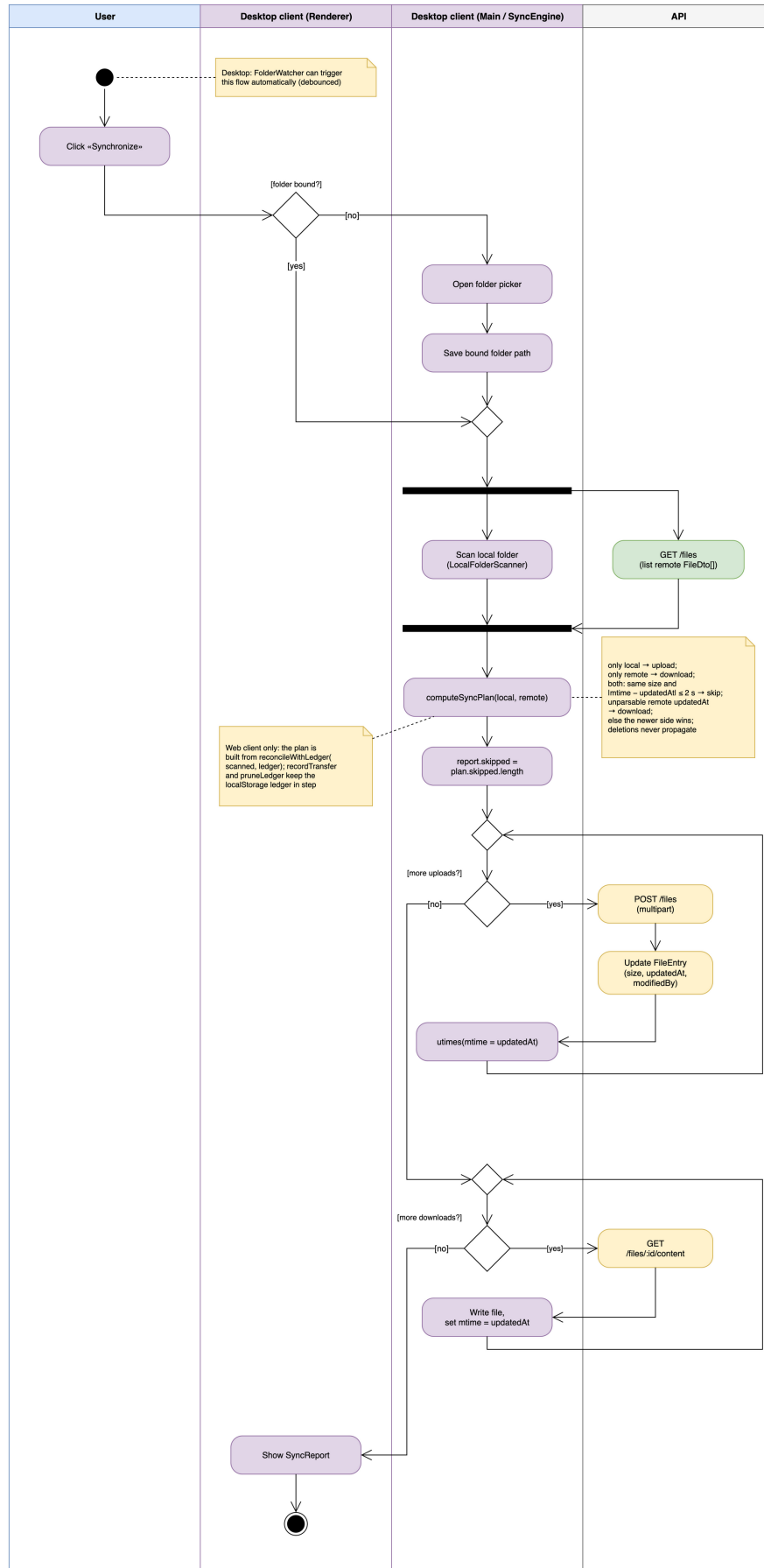
Рисунок 8. Рис. 8. Активність: синхронізація
