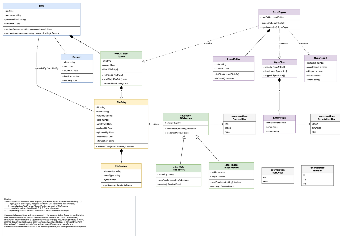
Рисунок 4. Рис. 4. Доменна модель
