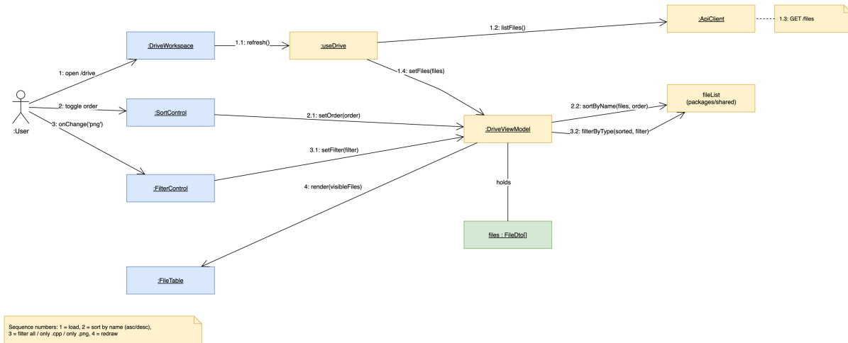
Рисунок 13. Рис. 13. Комунікація: сортування та фільтрація
