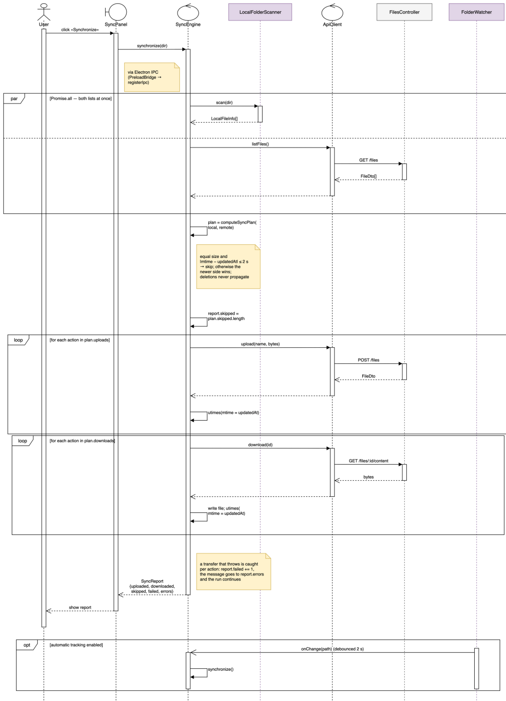
Рисунок 12. Рис. 12. Послідовність: синхронізація
