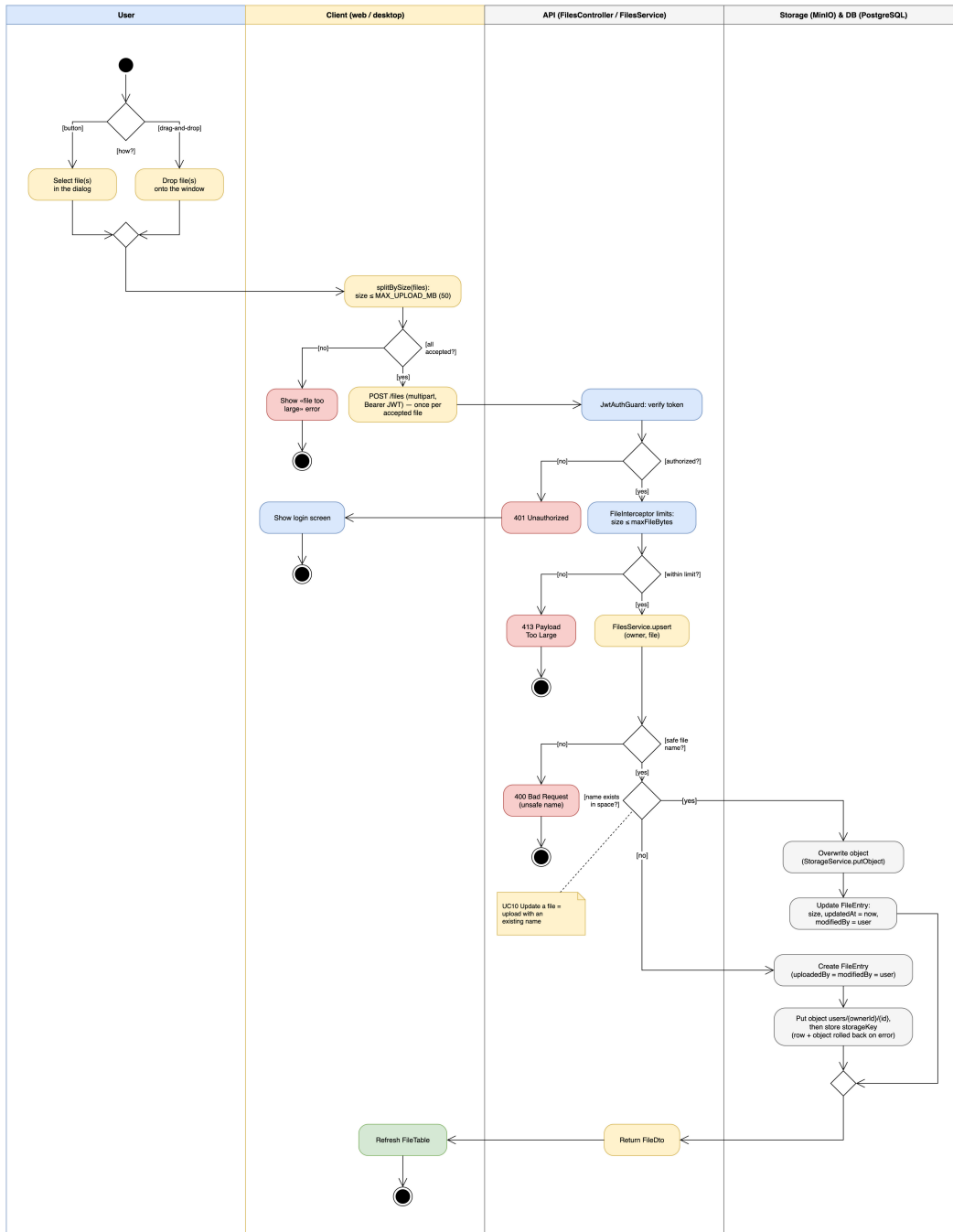
Рисунок 9. Рис. 9. Активність: завантаження
