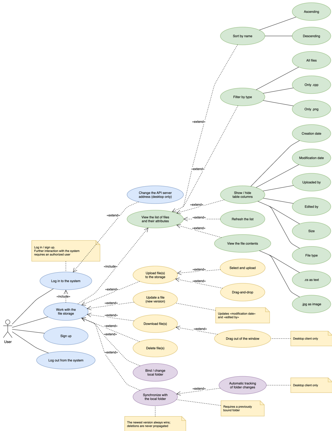
Рисунок 3. Рис. 3. Діаграма прецедентів
