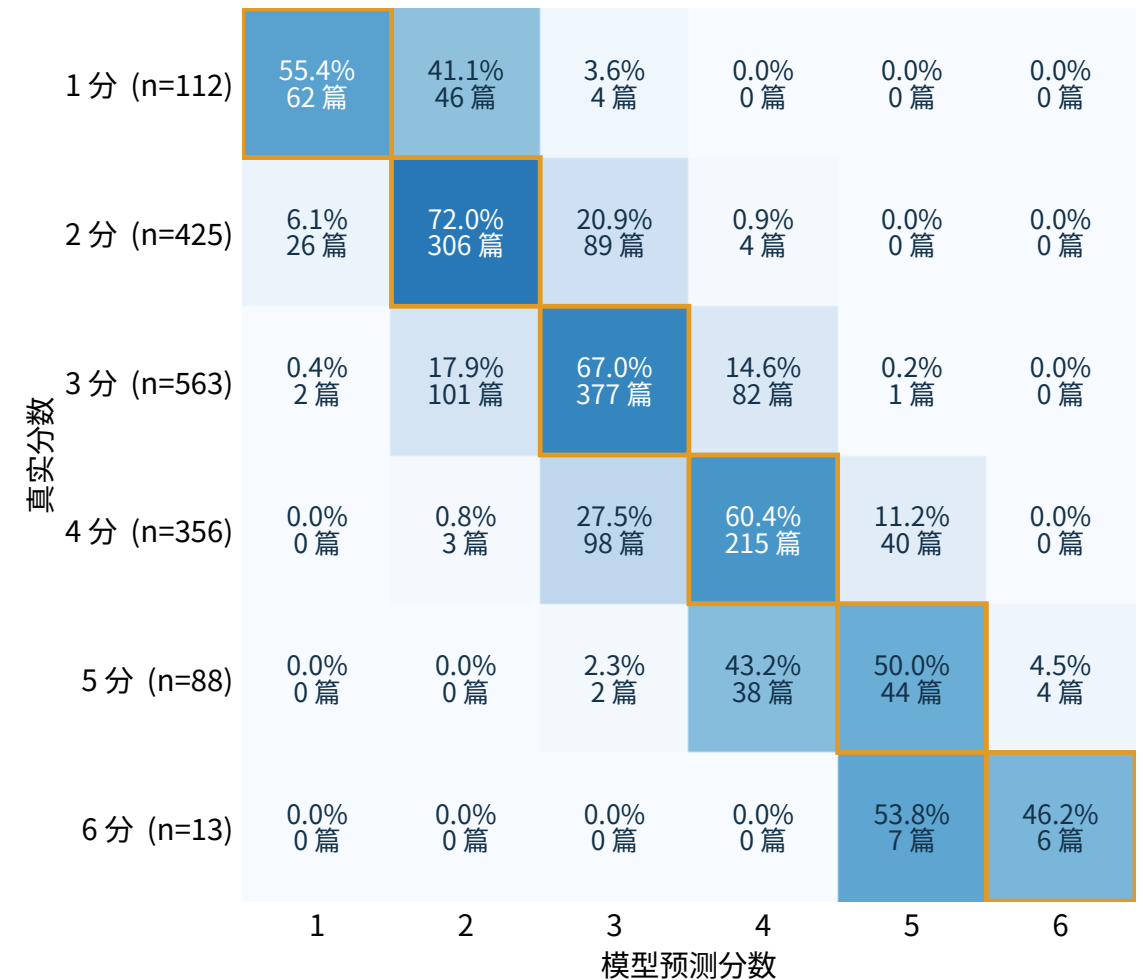
B0 · 固定半整数阈值 QWK = 0.81984
