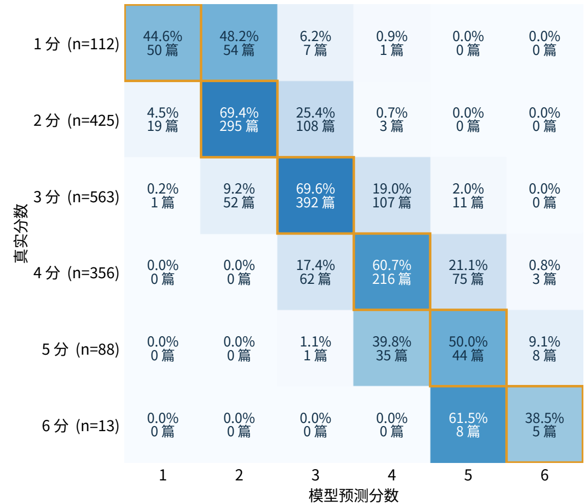
B0 · 固定半整数阈值 QWK = 0.81429
