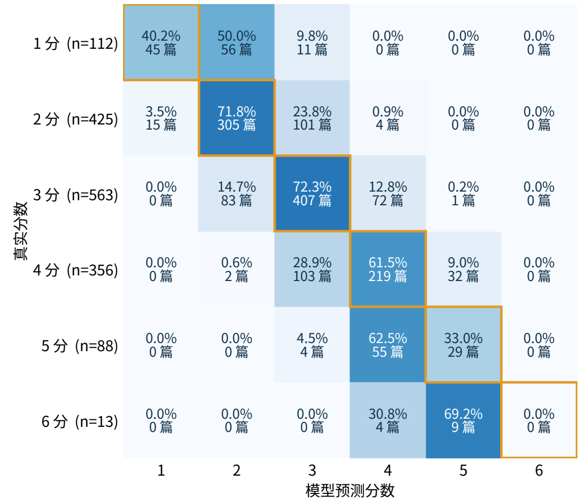
B0 · 固定半整数阈值 QWK = 0.79104
