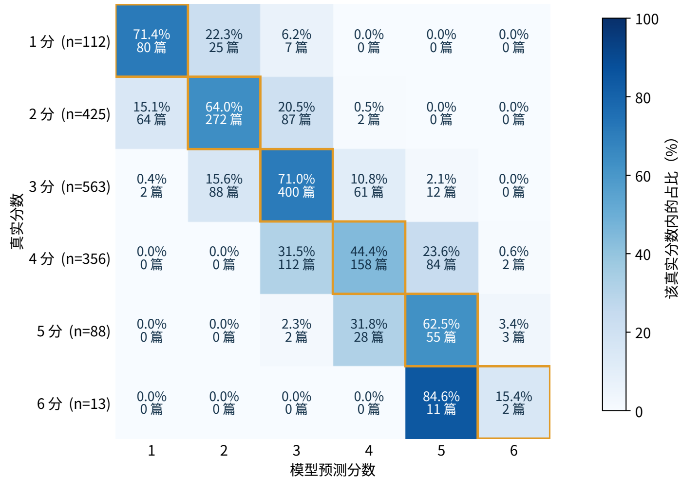
B1 · calibration 集拟合阈值 QWK = 0.81457
