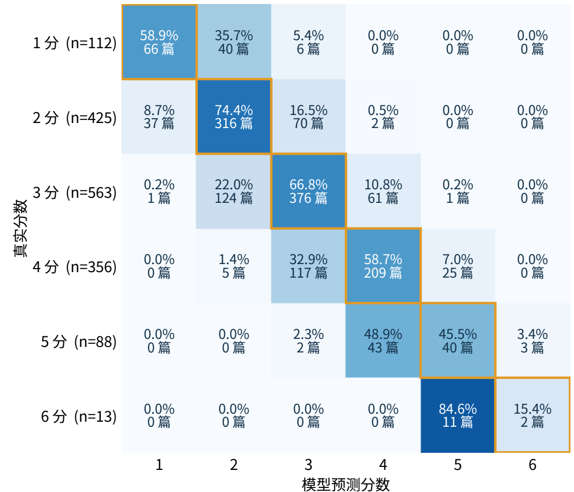
B0 · 固定半整数阈值 QWK = 0.81547
