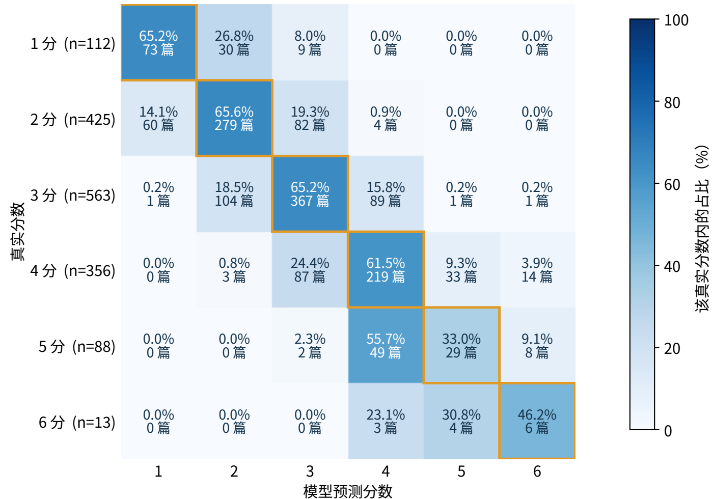
B1 · calibration 集拟合阈值 QWK = 0.80102
