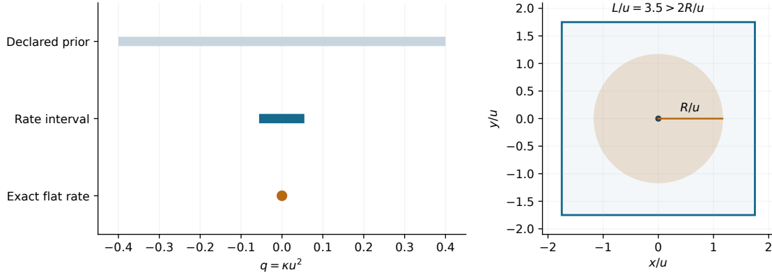
Рис. 2: Слева: синтетический исходный интервал кривизны, уточнение интервалом скорости и точная плоская скорость. Справа: двумерное сечение, иллюстрирующее инъективный шар внутри кубической фундаментальной области тора; полная конструкция трёхмерна. Подгонка космологических данных не показана.
