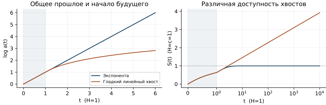
Рис. 2: Синтетический пример H = c = 1 , T_* = 1 , \delta = 1/2 . Истории и доступность совпадают до переключения; затем экспоненциальный путь стремится к единице, а путь с гладким линейным хвостом неограничен. Конечные значения графика не доказывают расходимость; её доказывает формула (10).
