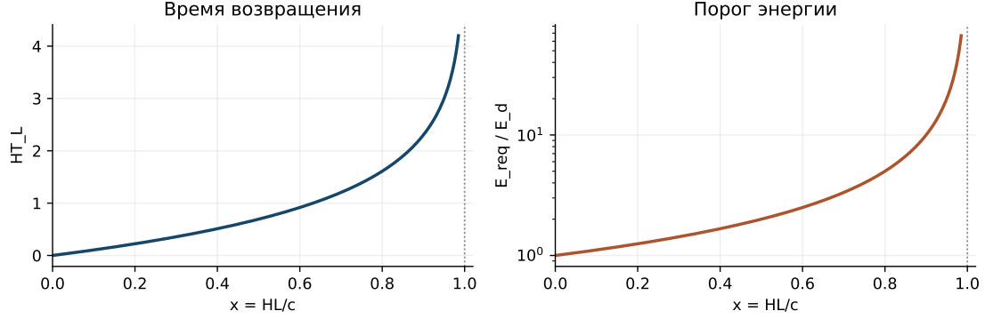
Рис. 1: Синтетическая экспоненциальная модель: нормированное время возвращения и необходимая энергия. Причинная граница x = 1 исключена; конечные ресурсные пороги могут достигаться. Подгонки космологических данных нет.
