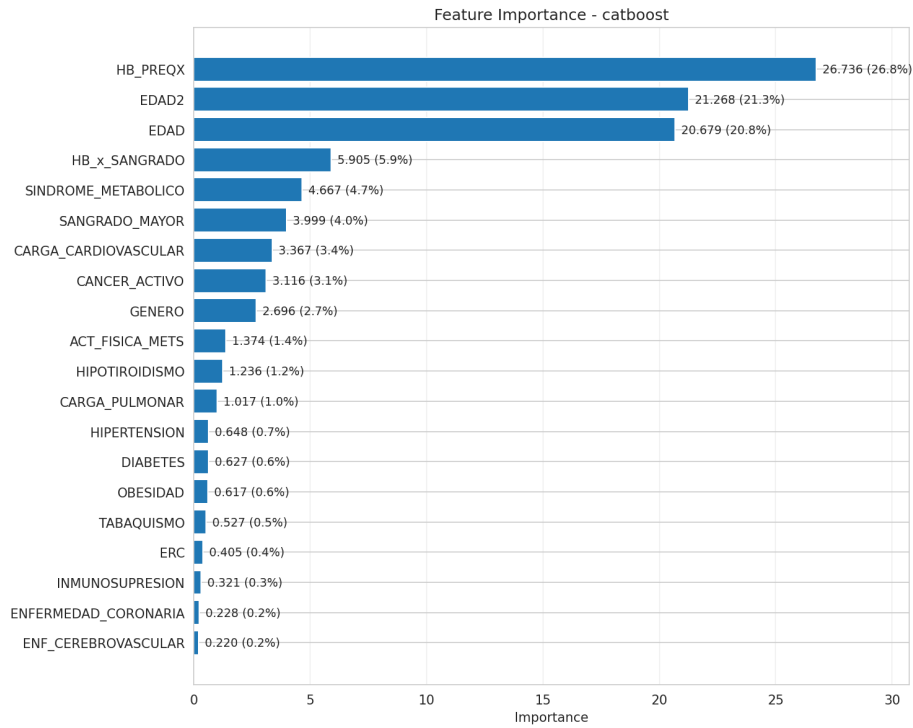
Figura 4: Importancia de variables del modelo lider (catboost) en el Experimento 2
