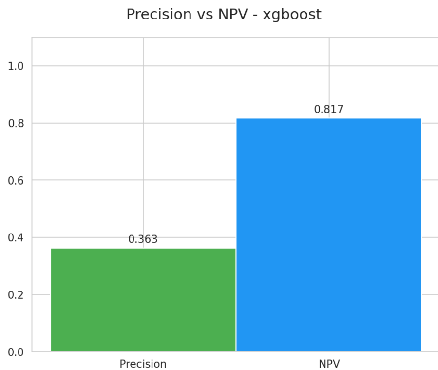
Figura 18: Comparativa precision-NPV para xgboost en el Experimento 5
