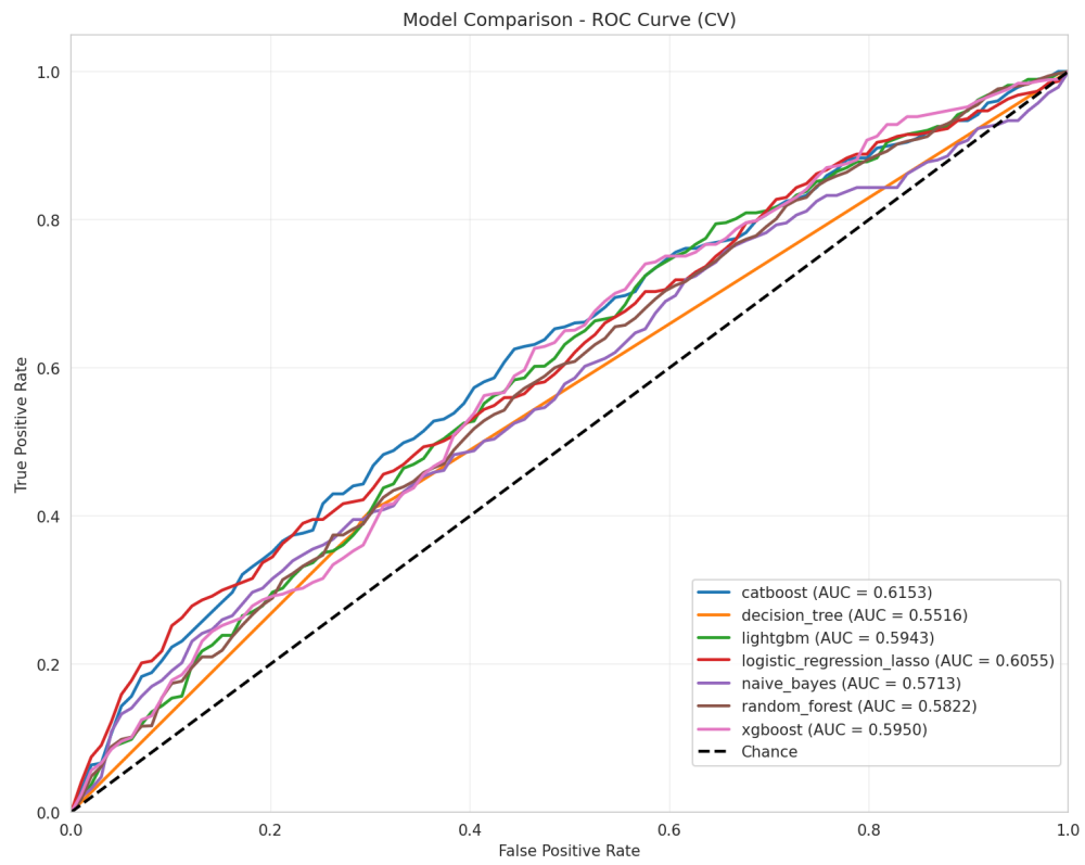
Figura 1: Comparacion ROC global del Experimento 1
