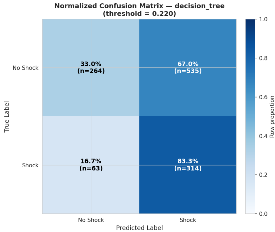
Figura 25: Matriz de confusion normalizada para decision_tree en el Experimento 5
