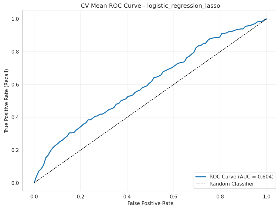
Figura 9: Curva ROC en CV para logistic_regression_lasso en el Experimento 4
