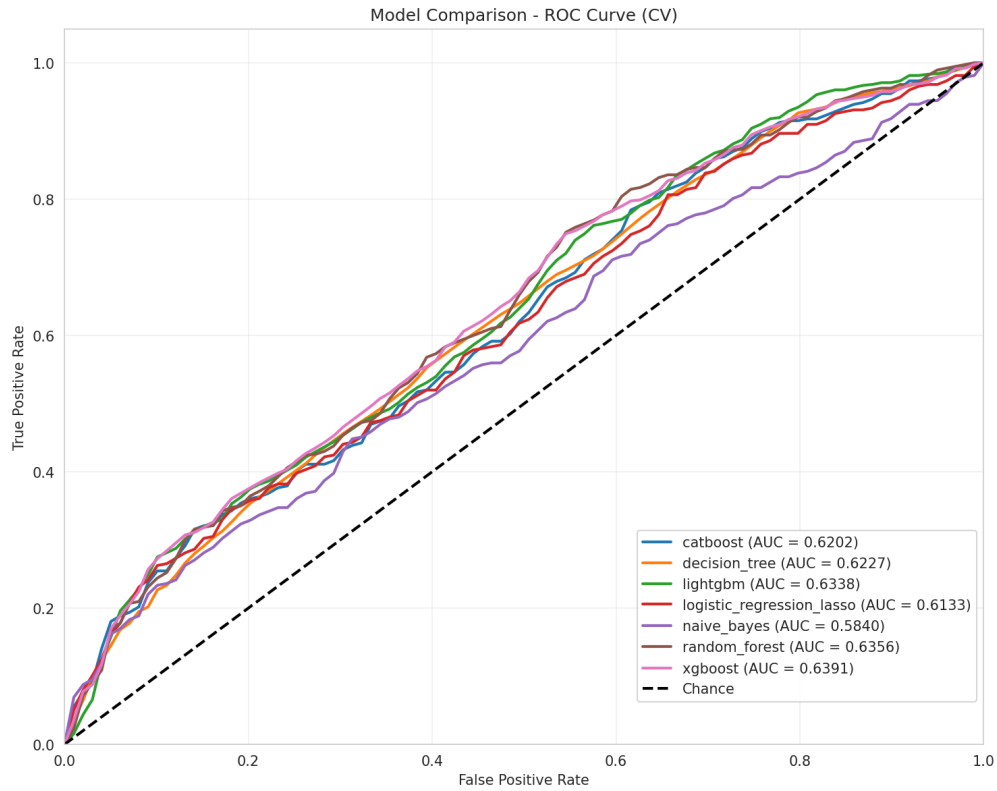
Figura 11: Comparacion ROC global del Experimento 5
