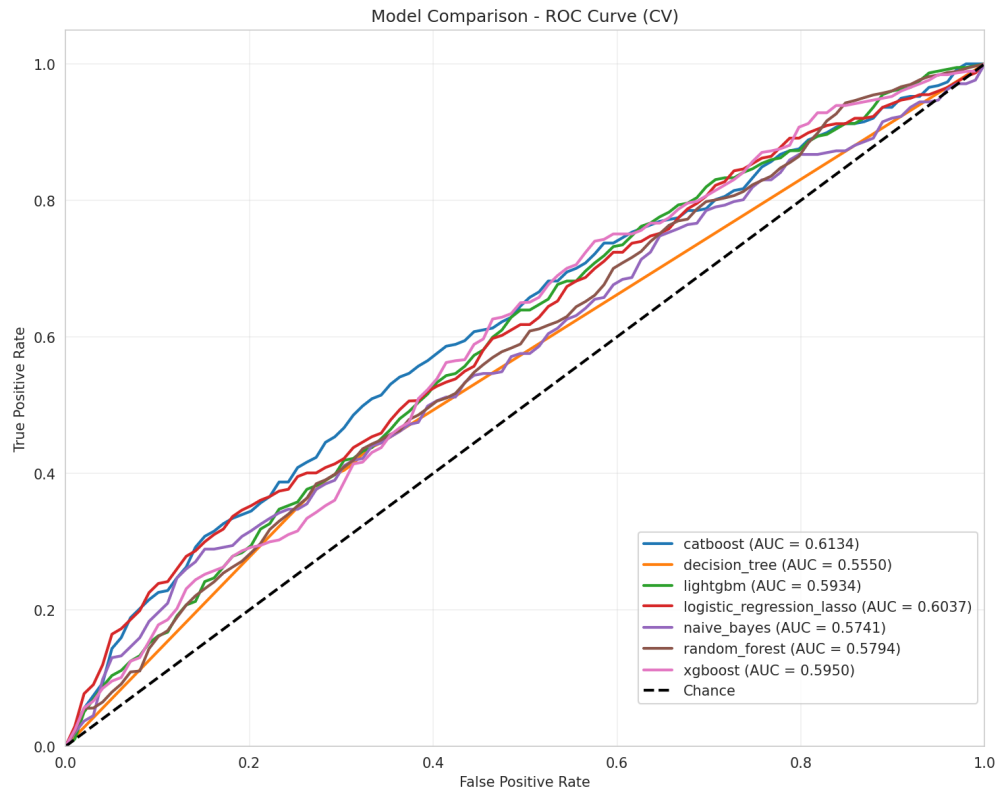
Figura 5: Comparacion ROC global del Experimento 3
