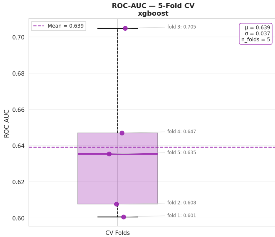
Figura 16: Boxplot de AUC-ROC por fold para xgboost en el Experimento 5
