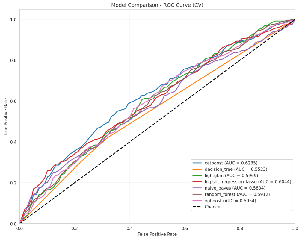
Figura 28: Comparación de curvas ROC - Experimento 2
