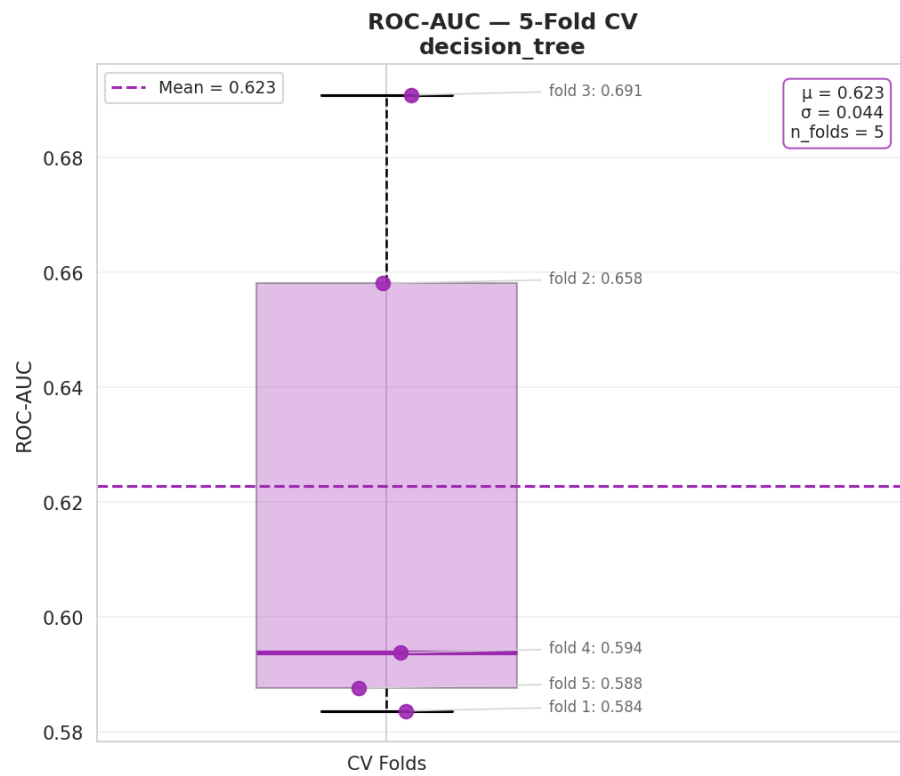
Figura 17: Boxplot de AUC-ROC por fold para decision_tree en el Experimento 5
