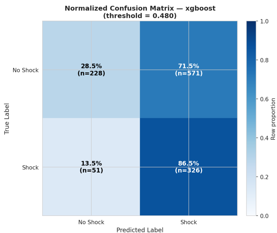
Figura 24: Matriz de confusion normalizada para xgboost en el Experimento 5
