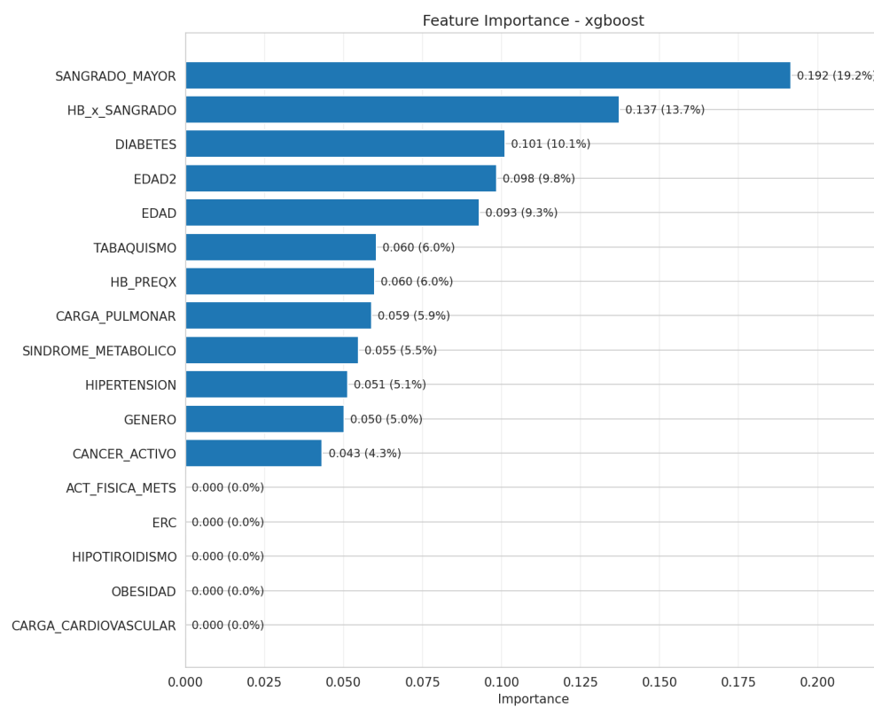
Figura 32: Importancia de características - Modelo Campeón (XGBoost)
