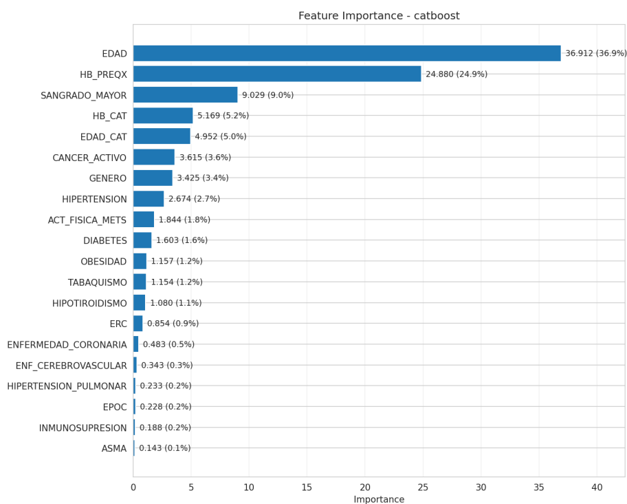
Figura 6: Importancia de variables del modelo lider (catboost) en el Experimento 3
