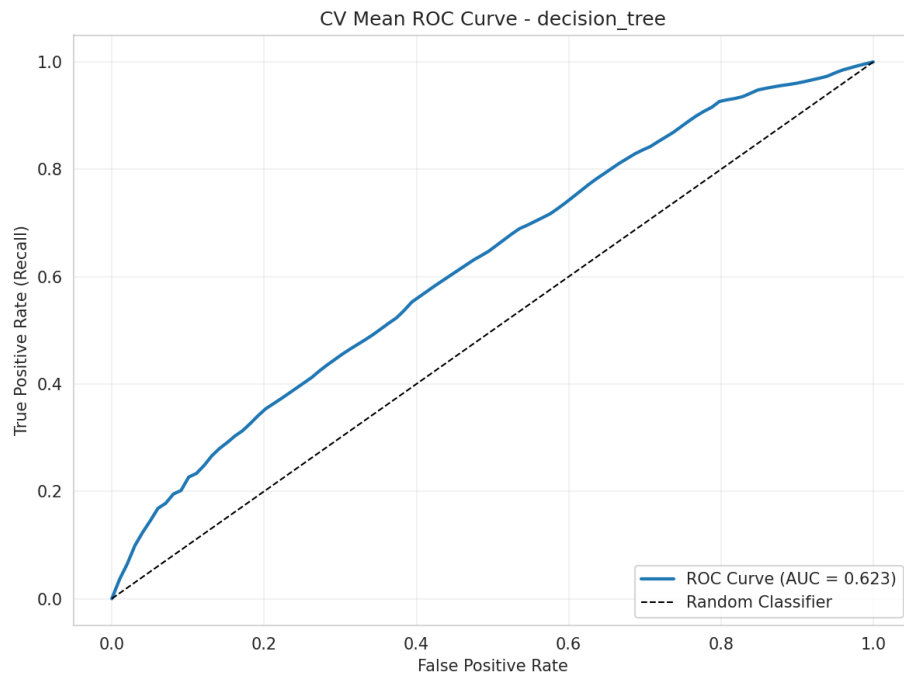
Figura 15: Curva ROC en CV para decision_tree (AUC=0.6227)
