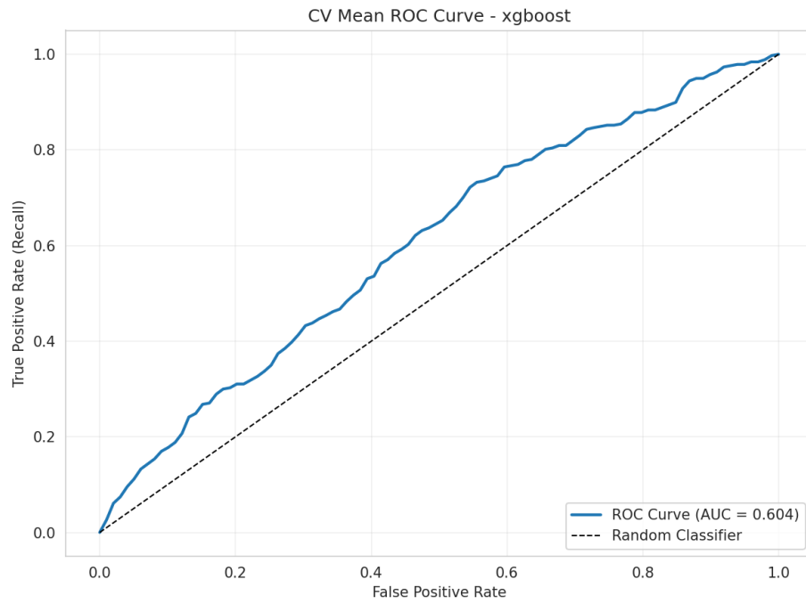
Figura 10: Curva ROC en CV para xgboost en el Experimento 4
