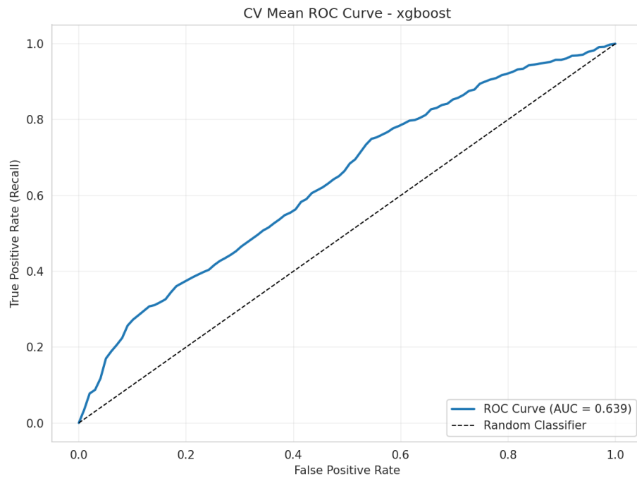
Figura 14: Curva ROC en CV para xgboost (AUC=0.6391)
