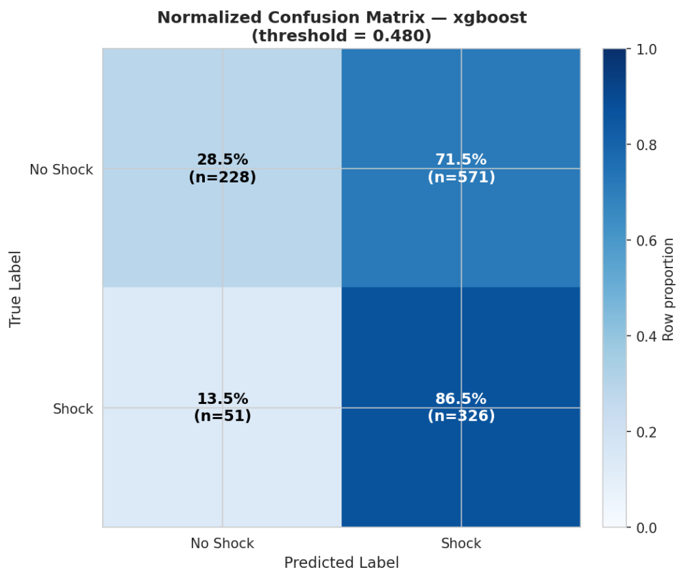
Figura 34: Matriz de confusión - Modelo Campeón (Umbral: 0.48)
