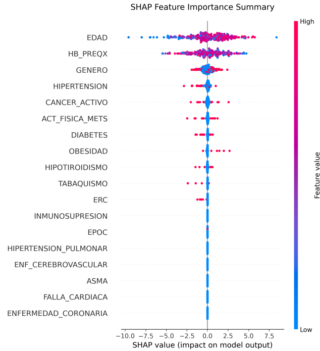
Figura 25: Gráfico de resumen SHAP para el modelo Random Forest optimizado. Cada punto representa el valor SHAP de una variable para un paciente específico. El color indica el valor normalizado de la variable (rojo: valor alto, azul: valor bajo). La posición en el eje X indica la dirección y magnitud del impacto en la predicción de riesgo de shock (valores positivos: incrementan el riesgo; valores negativos: reducen el riesgo).
