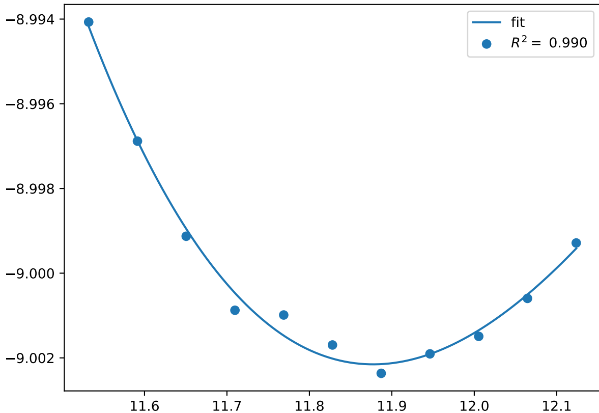
Cr_pv16Co_pv10W_sv4.sigma-BCAAB.FM
