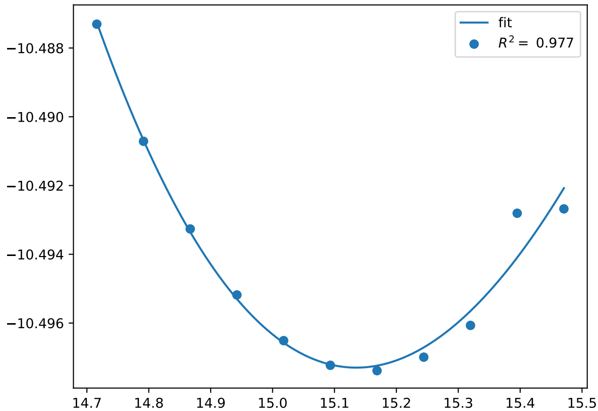
Co_pv8W_sv16.C36-BAABB.FM
