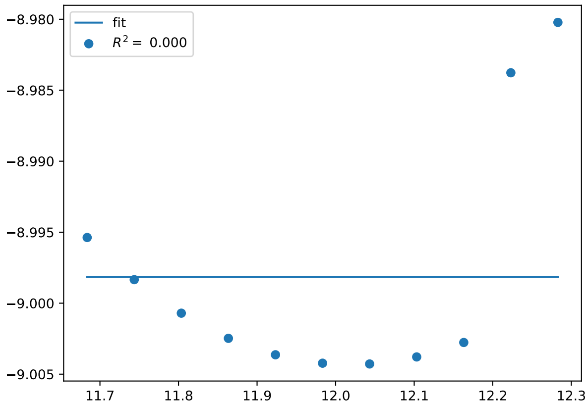
Co_pv8W_sv4.C14-BAA.FM
