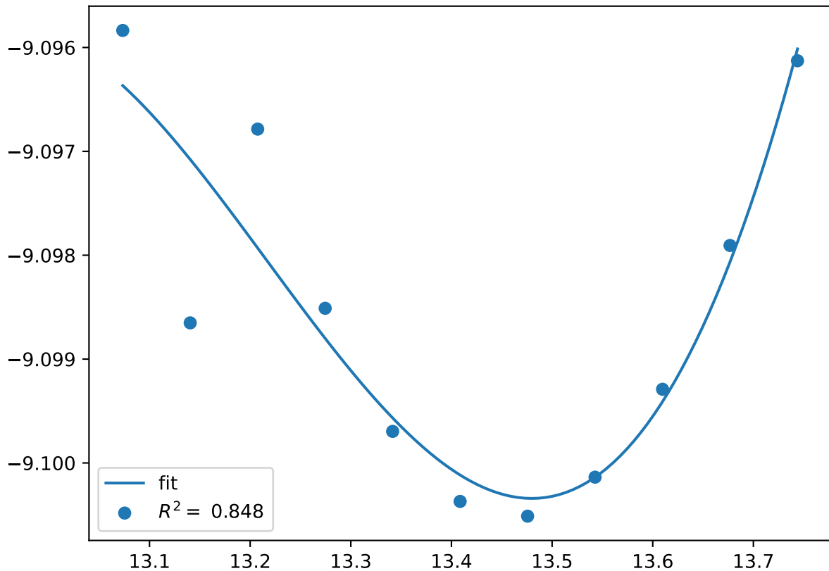
Co_pv17W_sv12.chi-AAAB.FM
