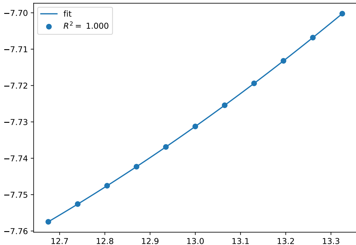
Cr_pv10Co_pv14.C36-ABBAB.FM
