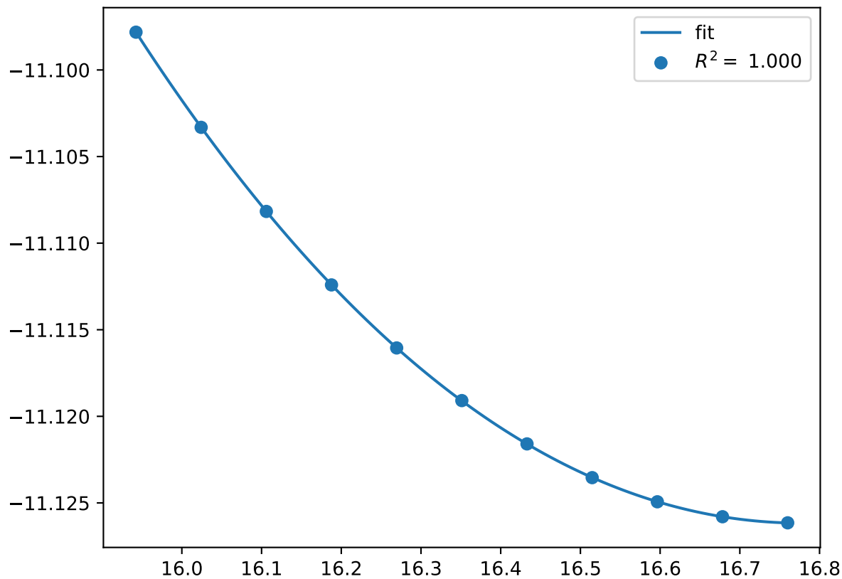
Cr_pv8W_sv16.C36-AABBB.FM
