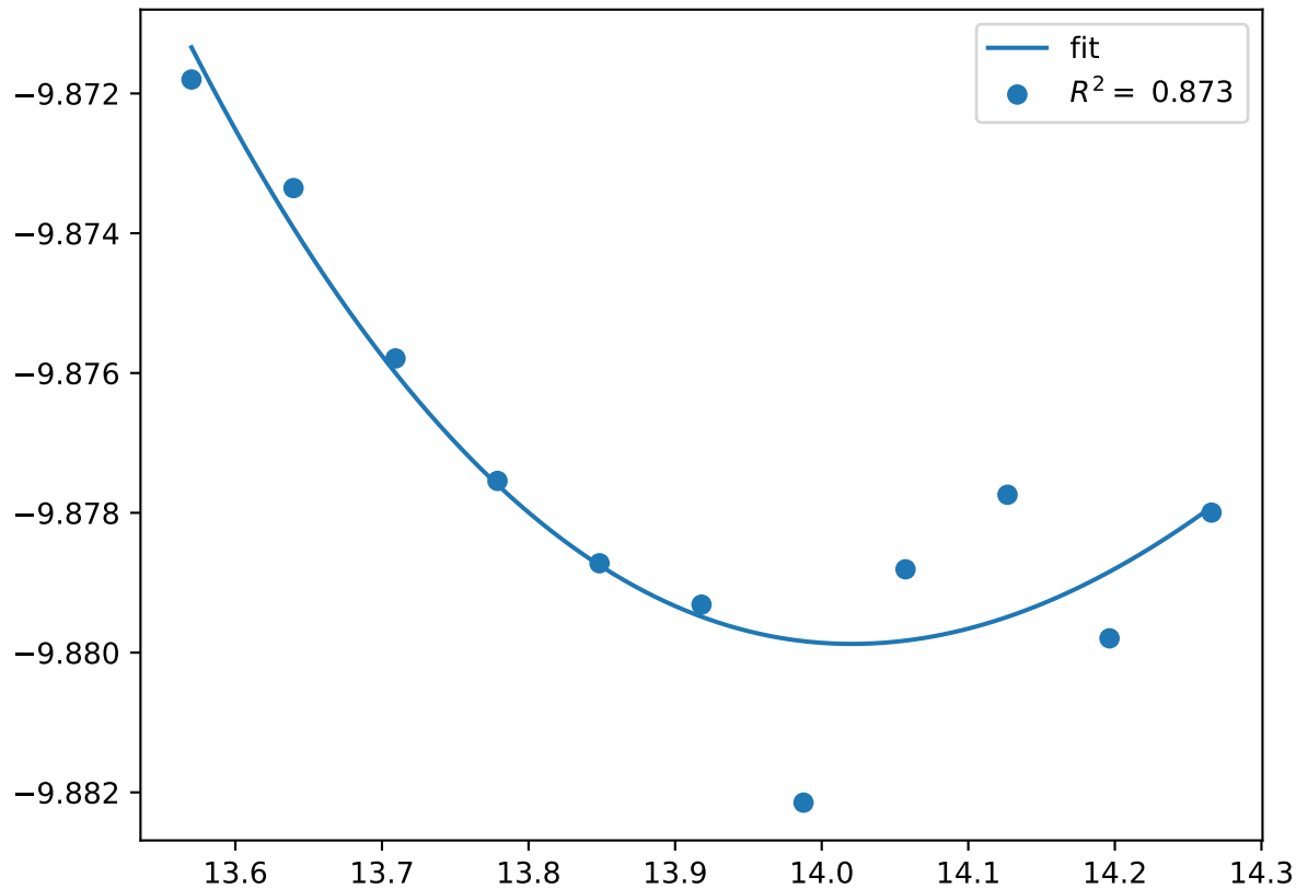
Co_pv14W_sv16.sigma-AABBA.FM
