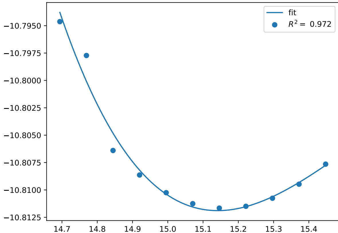
Cr_pv3Co_pv2W_sv8.mu-ACACB.FM
