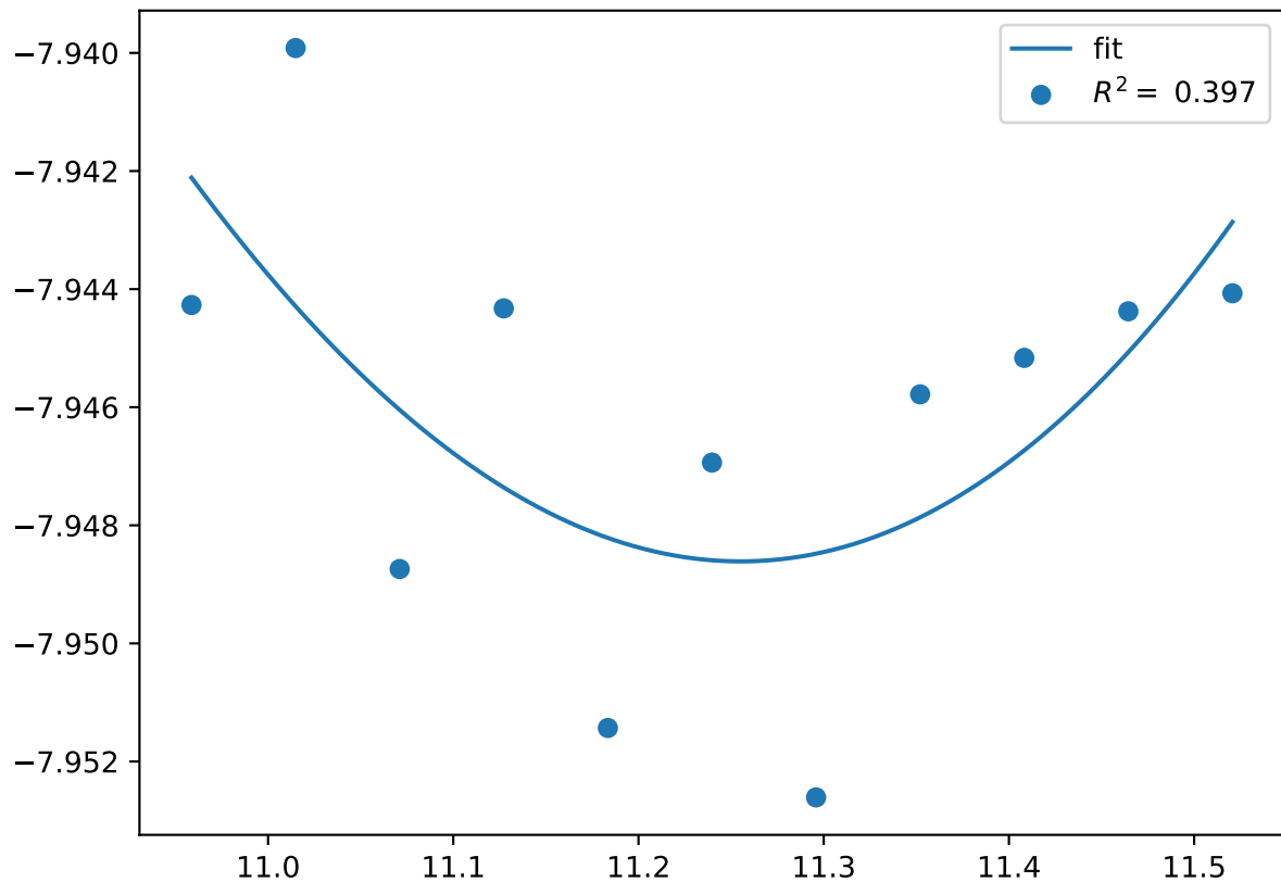
Cr_pv8Co_pv20W_sv2.sigma-CBABB.FM
