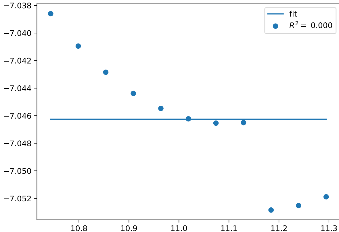
Cr_pv1Co_pv28.chi-ABBB.FM
