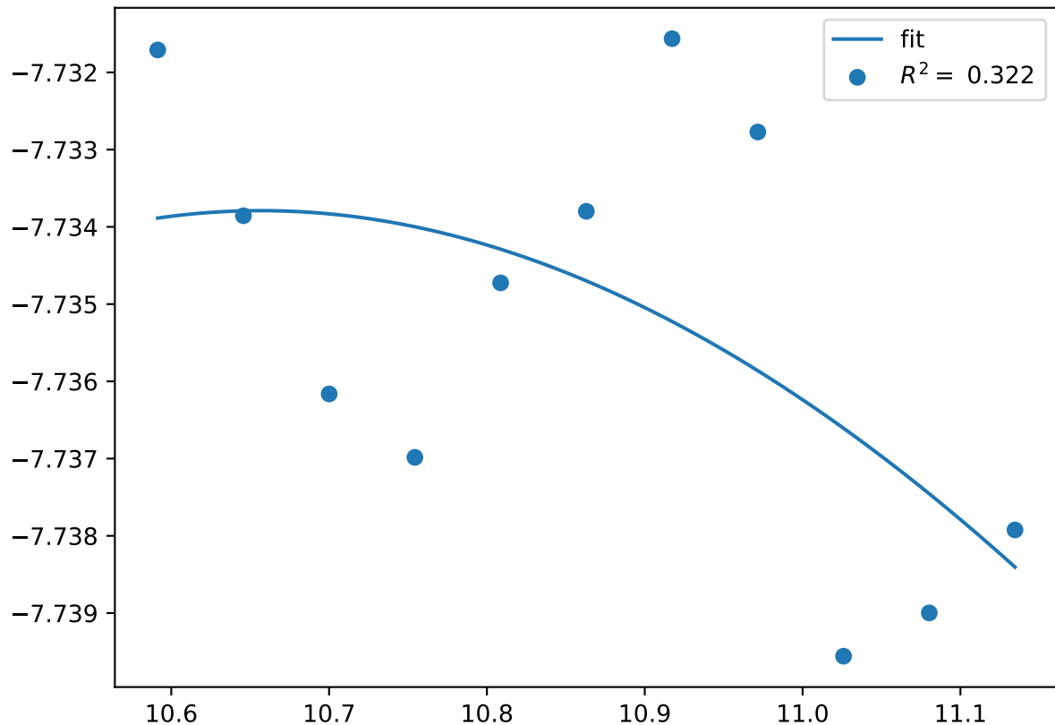
Cr_pv10Co_pv20.sigma-ABABB.FM
