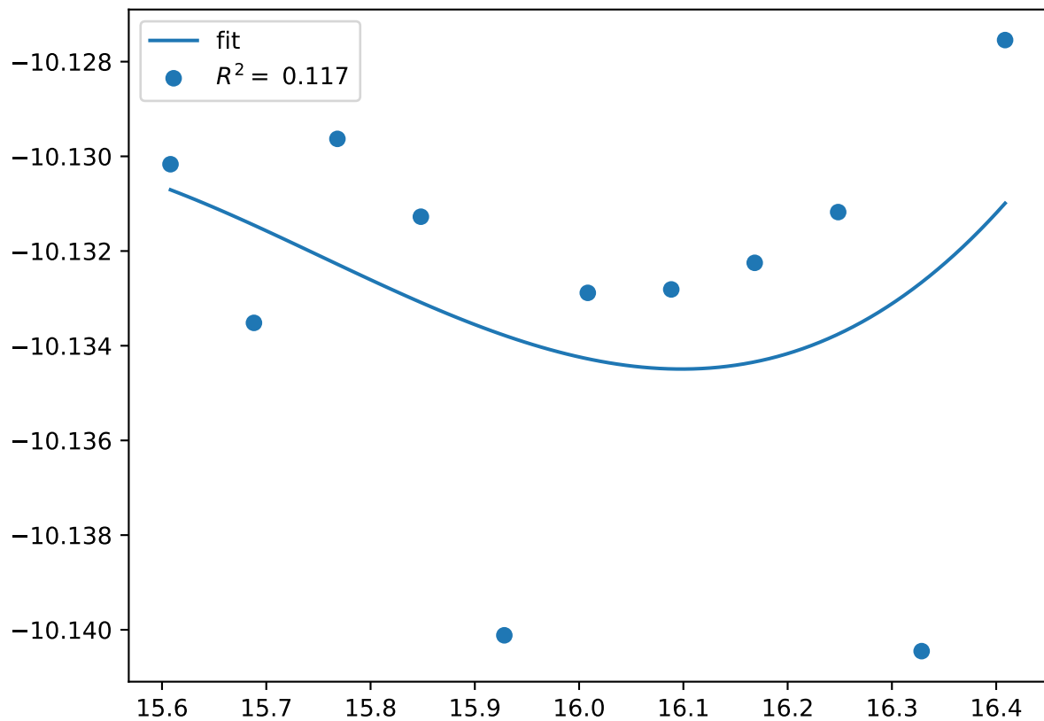
Co_pv4W_sv8.C14-ABB.FM
