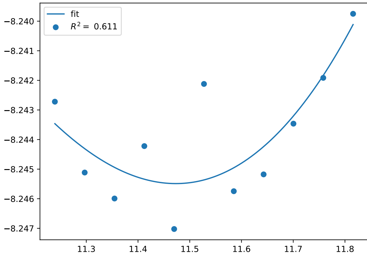
Cr_pv14Co_pv10.C36-AABAB.FM
