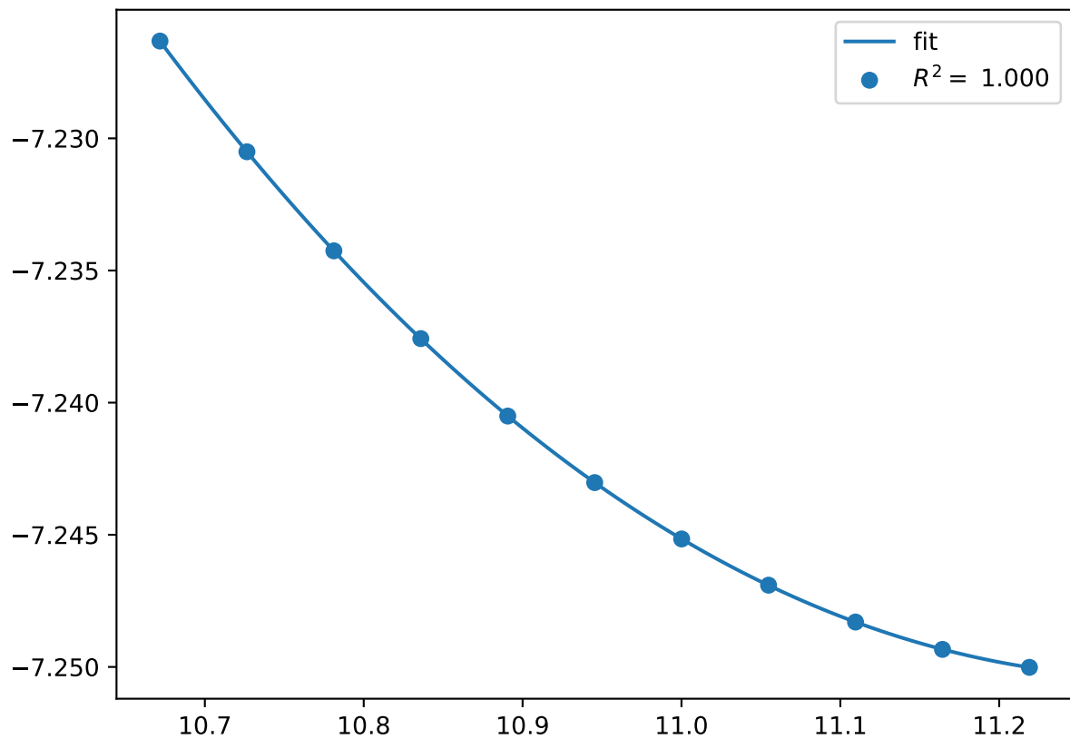
Cr_pv2Co_pv11.mu-BBBBA.FM
