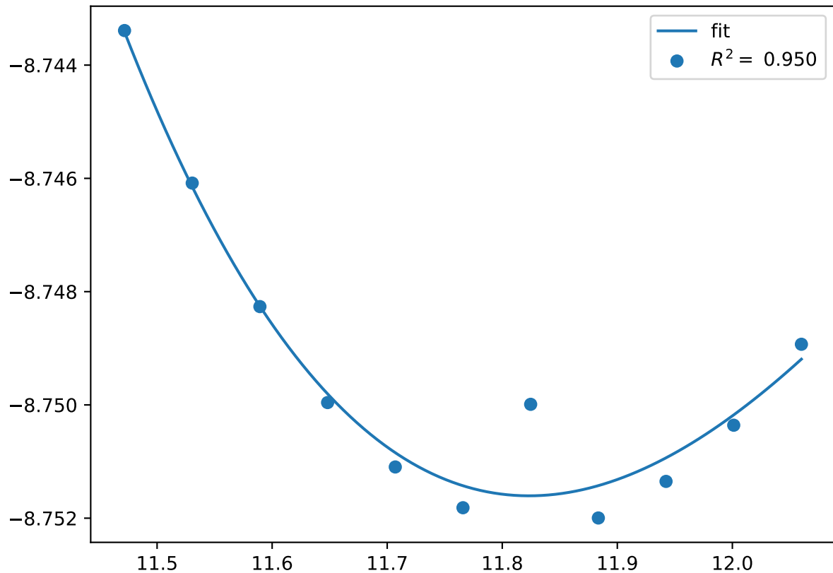
Cr_pv12Co_pv13W_sv4.chi-BCBA.FM
