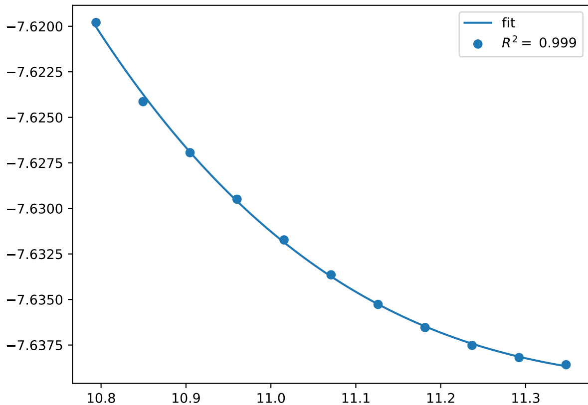
Cr_pv8Co_pv16.C36-BAABB.FM
