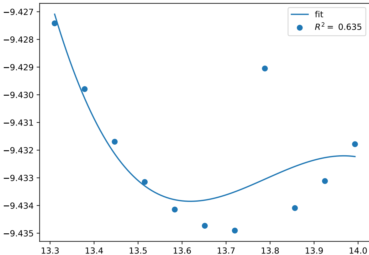
Cr_pv14Co_pv4W_sv6.C36-ABACA.FM
