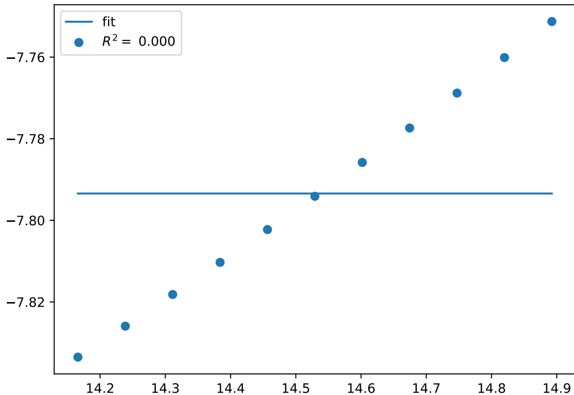
Cr_pv4Co_pv8W_sv1.mu-CBAAB.FM
