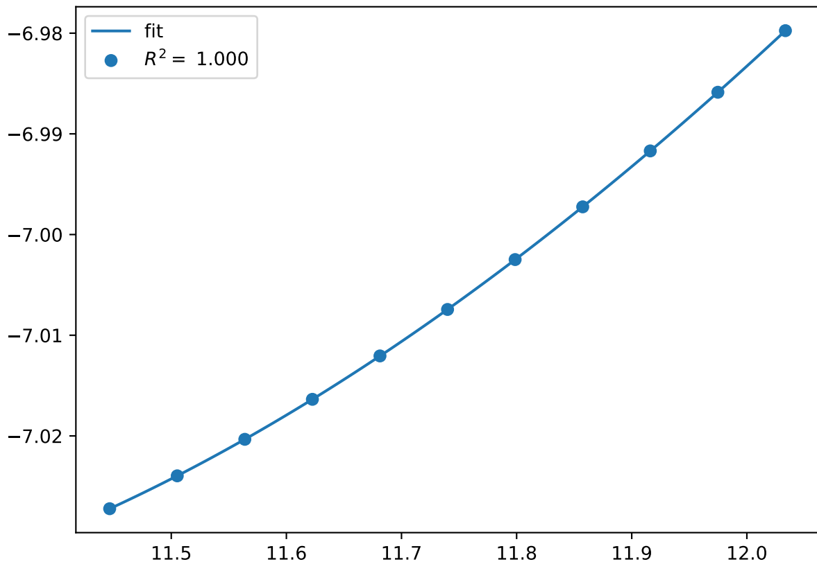
Cr_pv2Co_pv11.mu-BBBAB.NM
