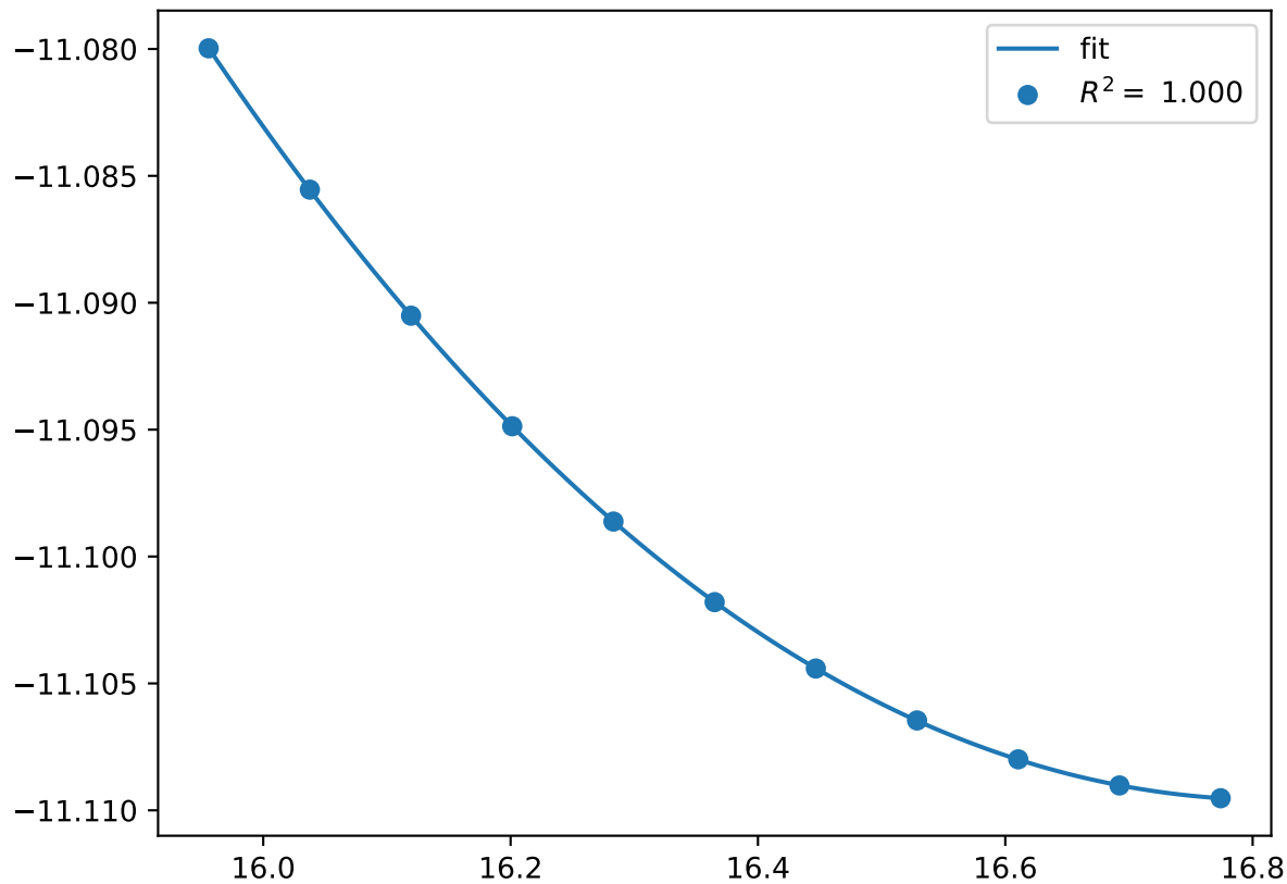
Cr_pv4W_sv8.C14-ABB.FM
