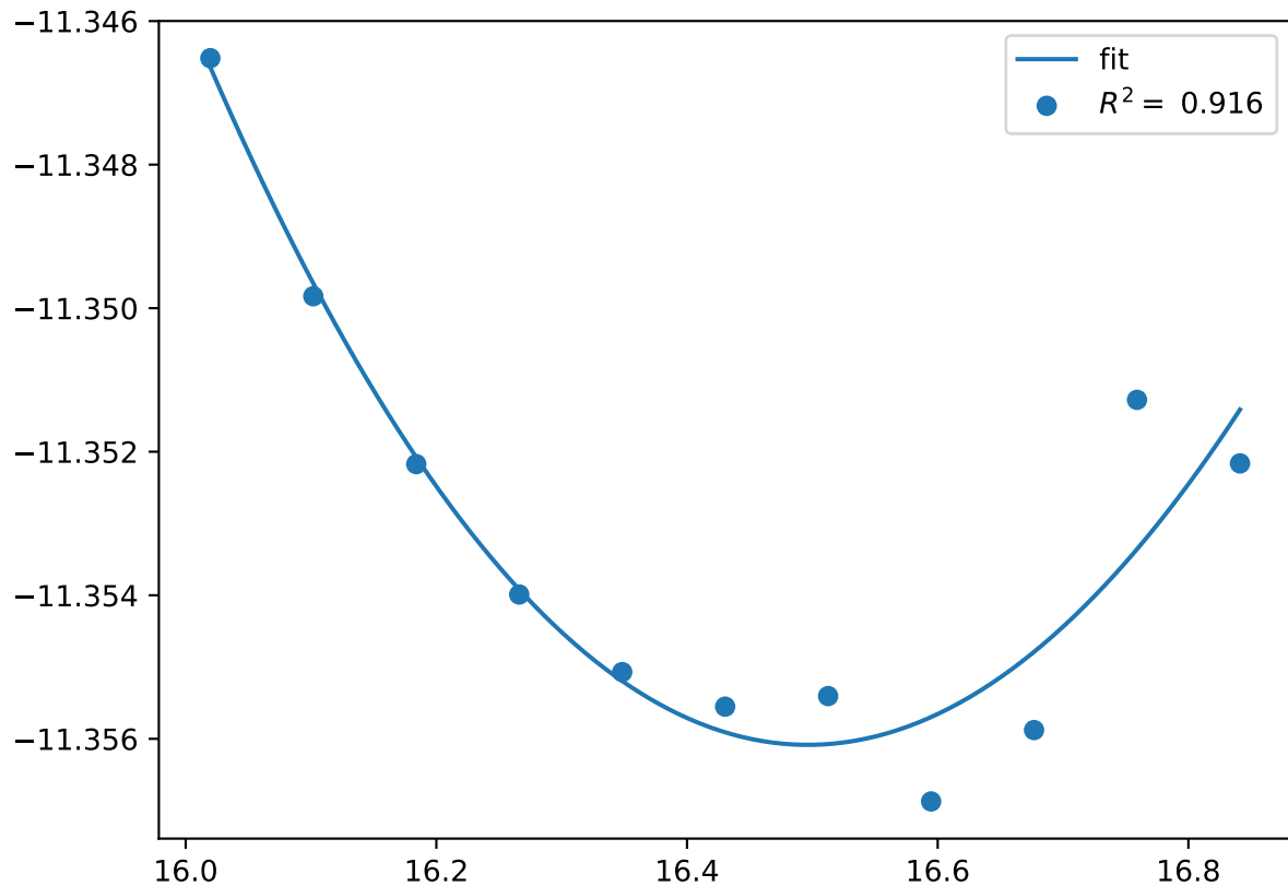
Co_pv4W_sv20.C36-BABBB.FM
