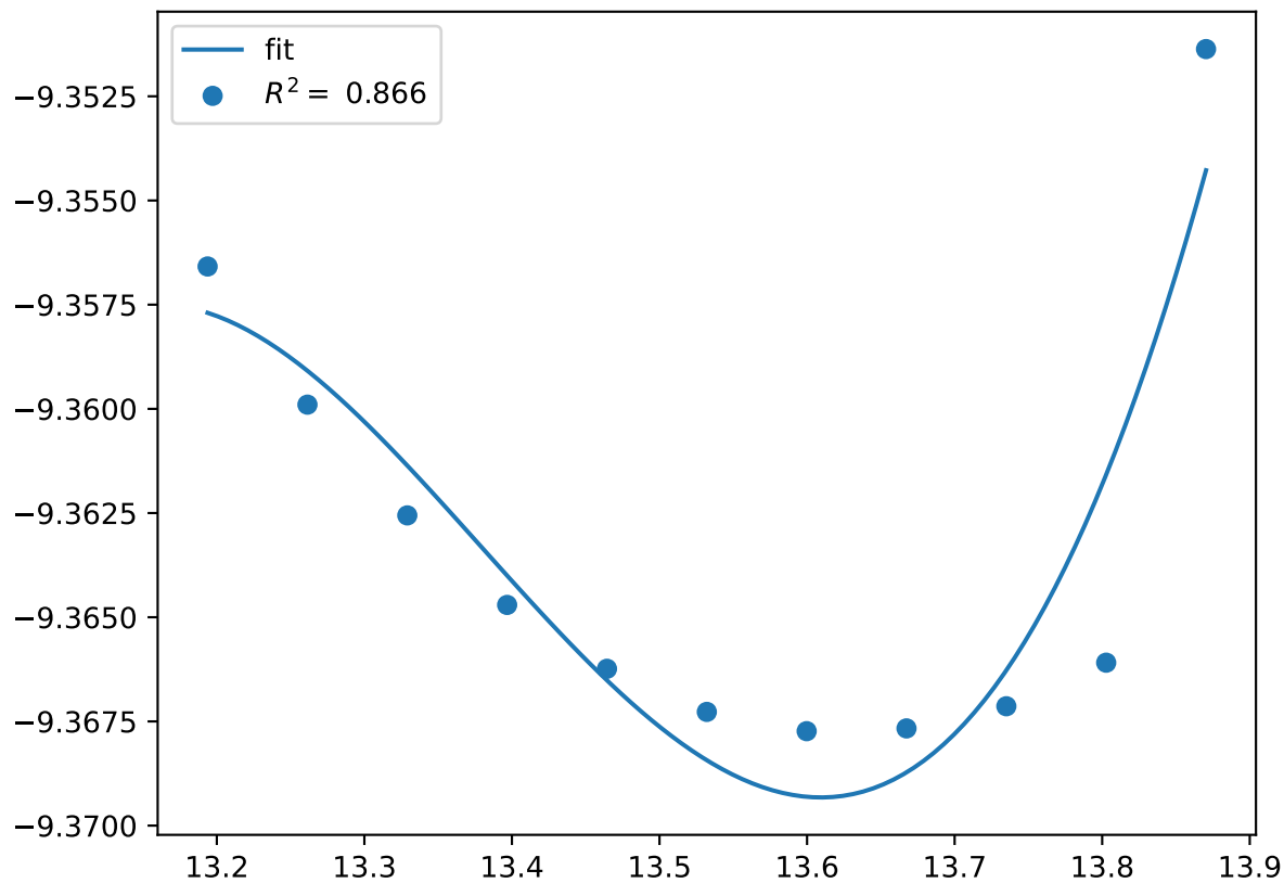
Co_pv16W_sv13.chi-BAAB.FM
