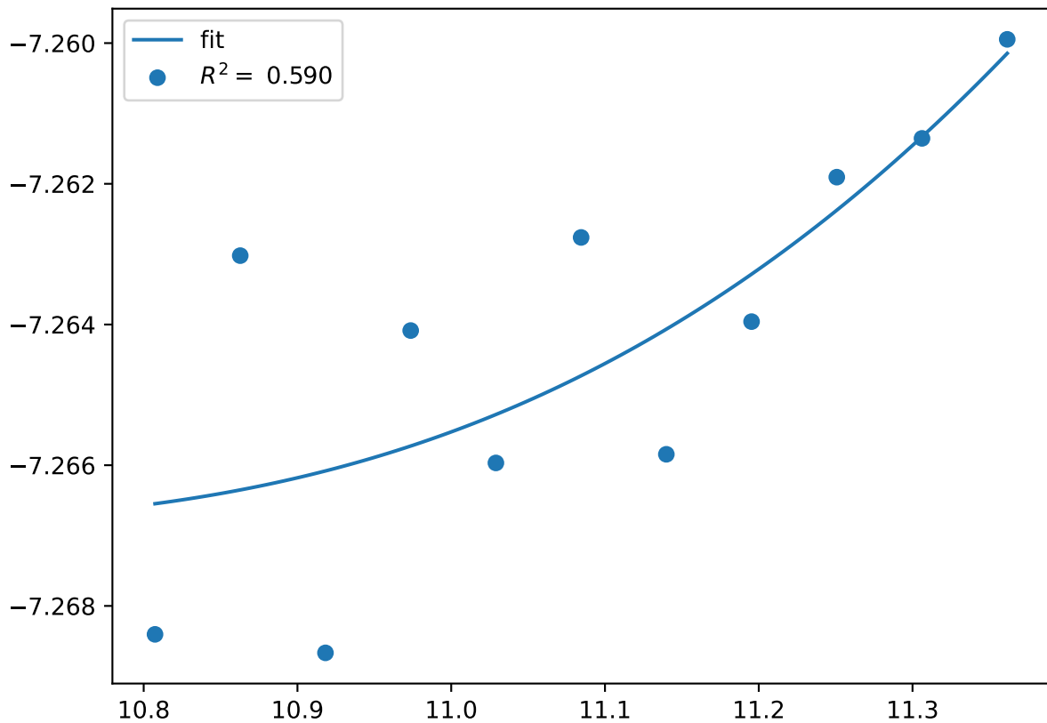
Cr_pv4Co_pv25.chi-BABB.FM
