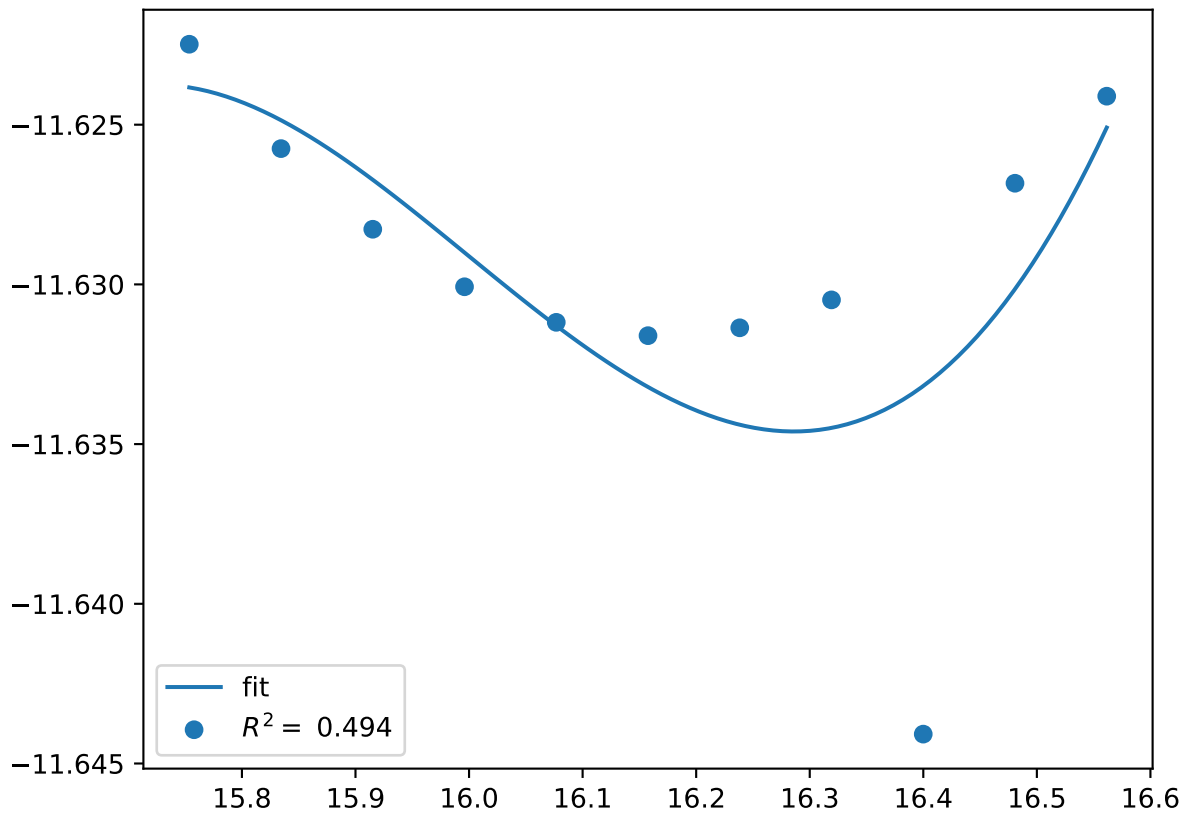
Co_pv4W_sv25.chi-BABB.FM
