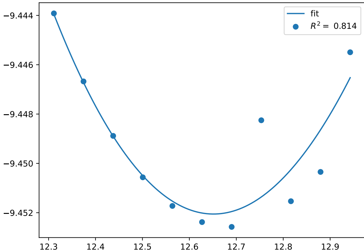
Cr_pv12Co_pv10W_sv8.sigma-BAABC.FM
