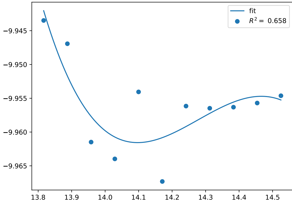
Cr_pv12Co_pv5W_sv12.chi-BBAC.FM
