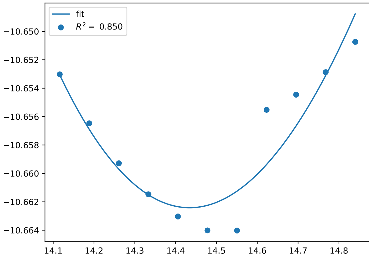
Cr_pv10Co_pv4W_sv16.sigma-ABCCA.FM
