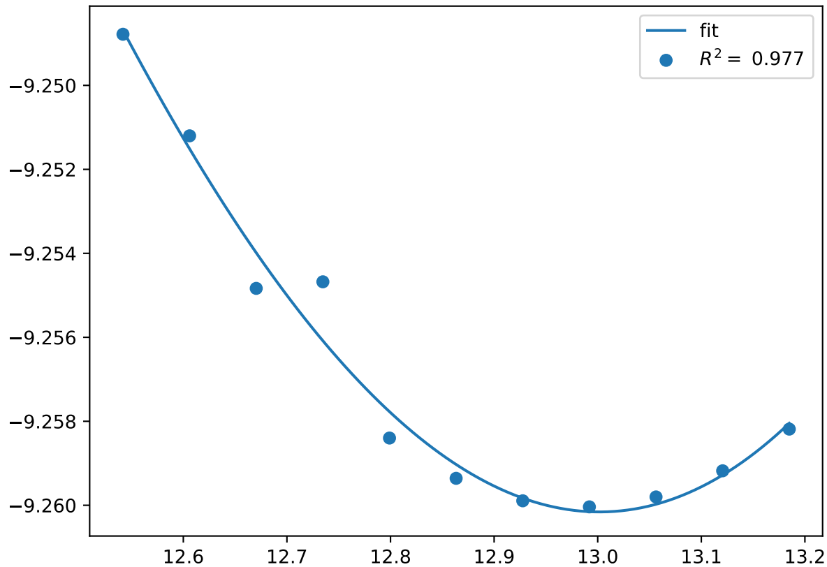
Cr_pv16Co_pv4W_sv4.C36-ABCAA.FM
