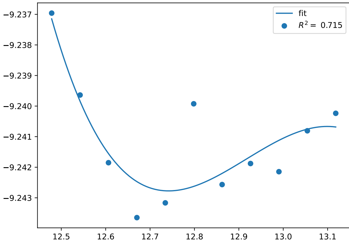
Cr_pv16Co_pv4W_sv4.C36-BACAA.FM
