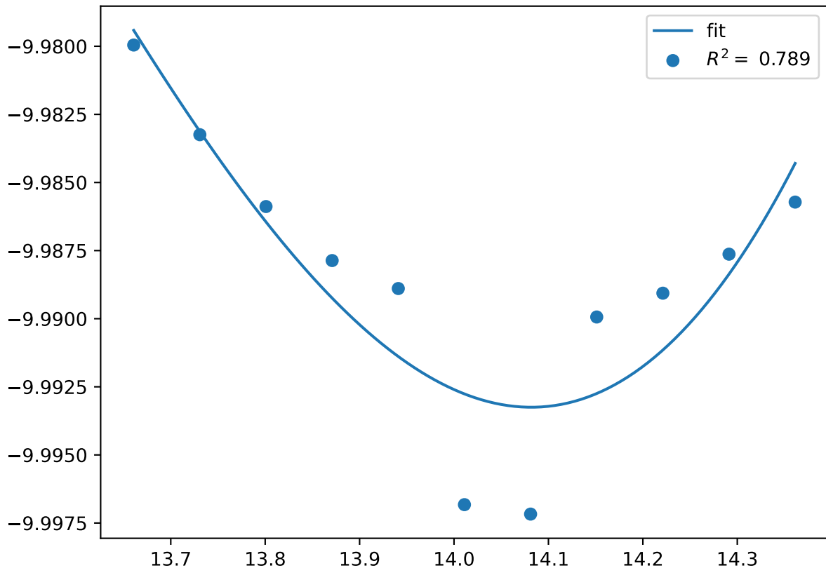
Co_pv13W_sv16.chi-ABAB.FM
