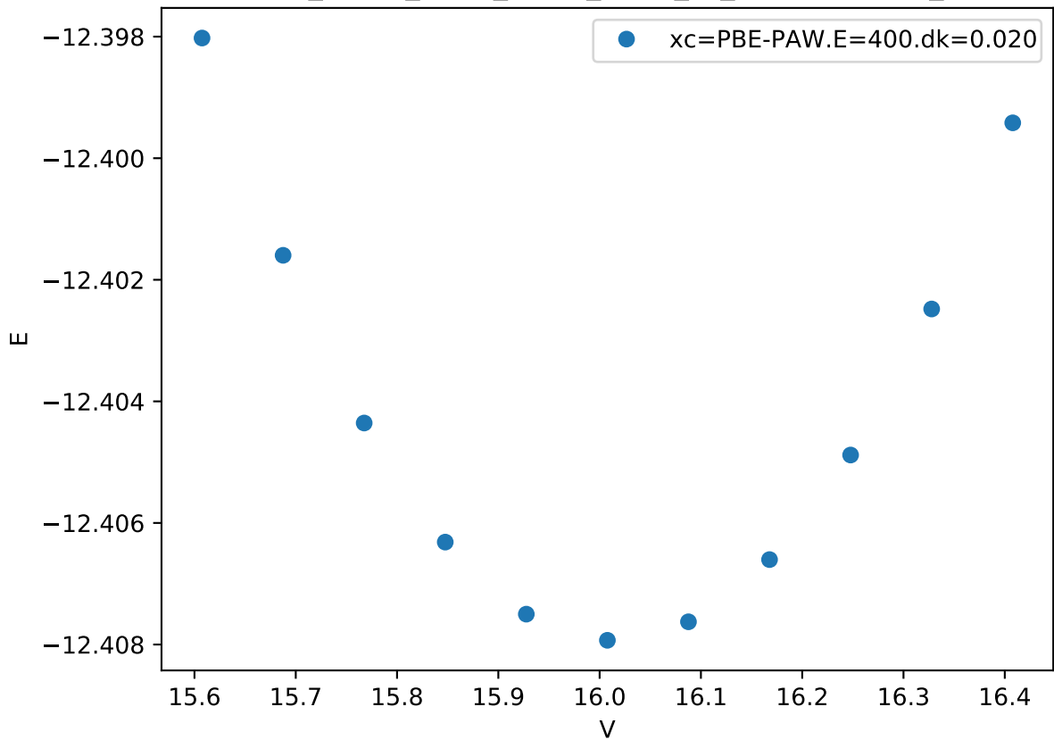
Cr_pv-Co_pv-W_sv/Co_pv-W_sv_sigma-ABBBB_
