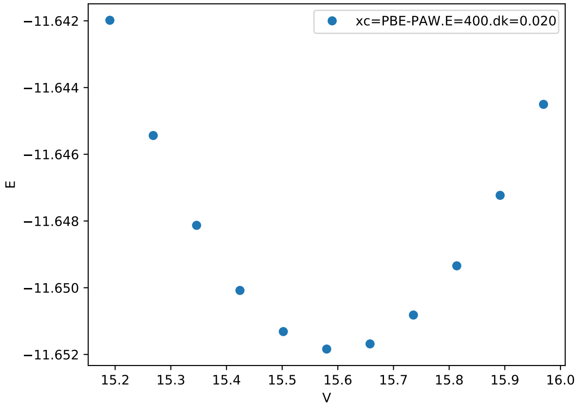
Cr_pv-Co_pv-W_sv/Co_pv-W_sv_C14-BAB.FM_
