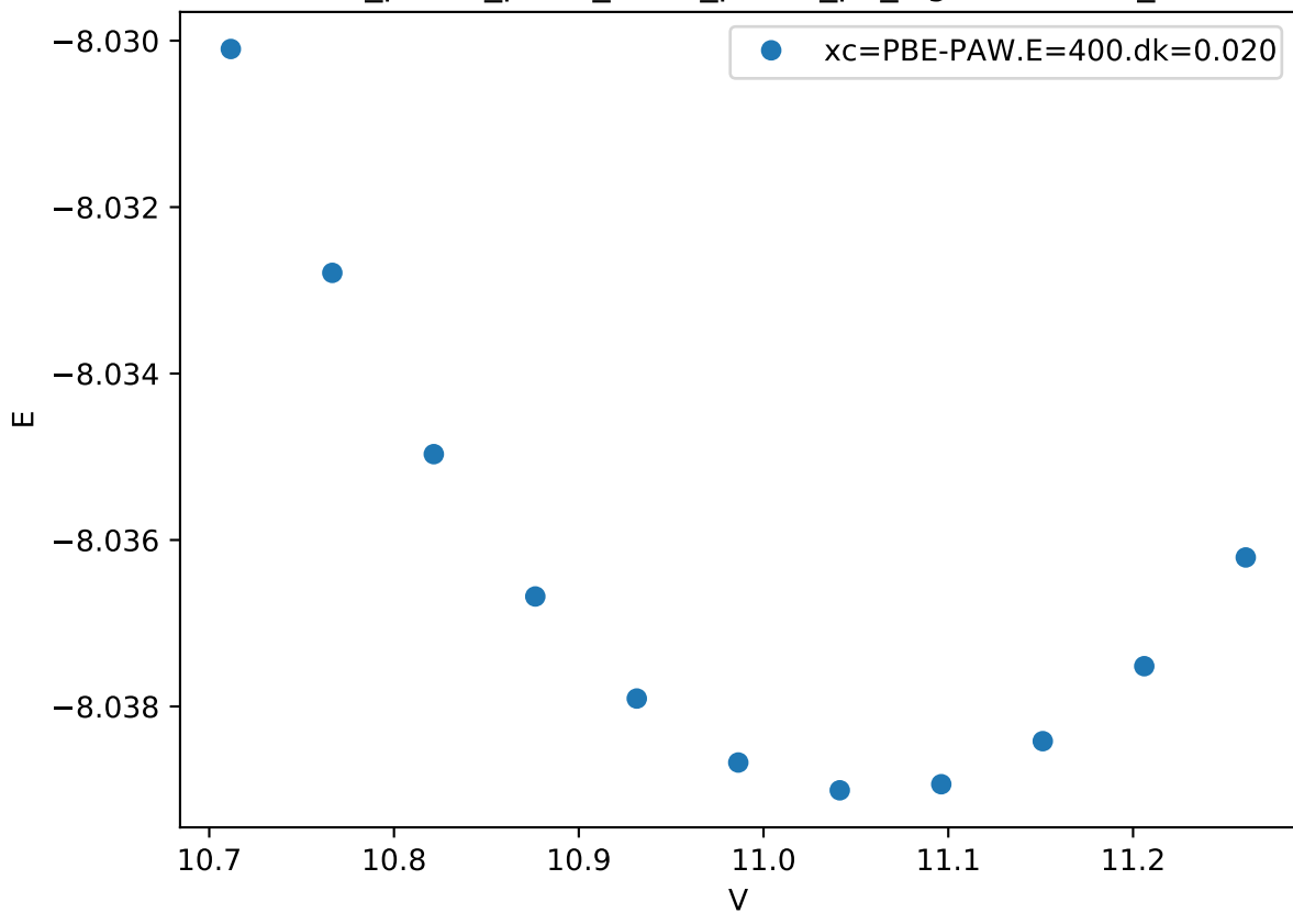
Cr_pv-Co_pv-W_sv/Cr_pv-Co_pv_sigma-AABAB_
