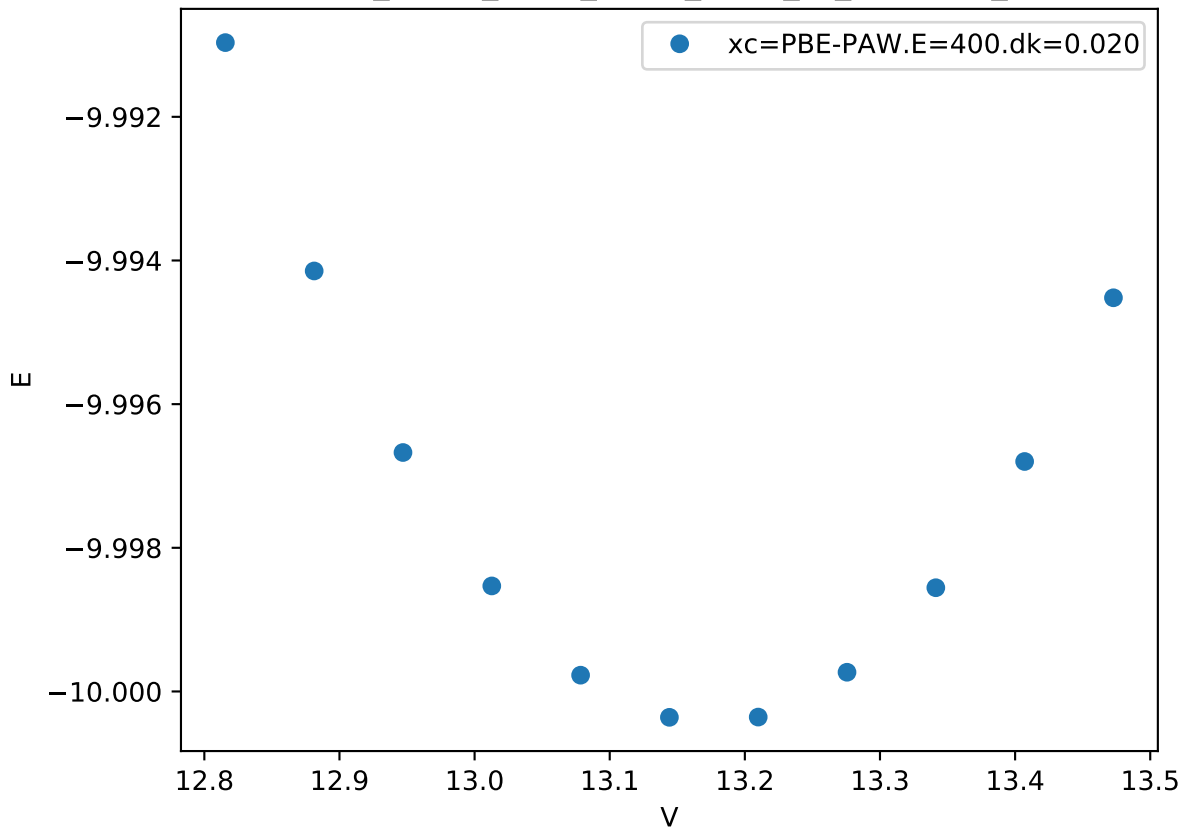
Cr_pv-Co_pv-W_sv/Co_pv-W_sv_C14-BBA_
