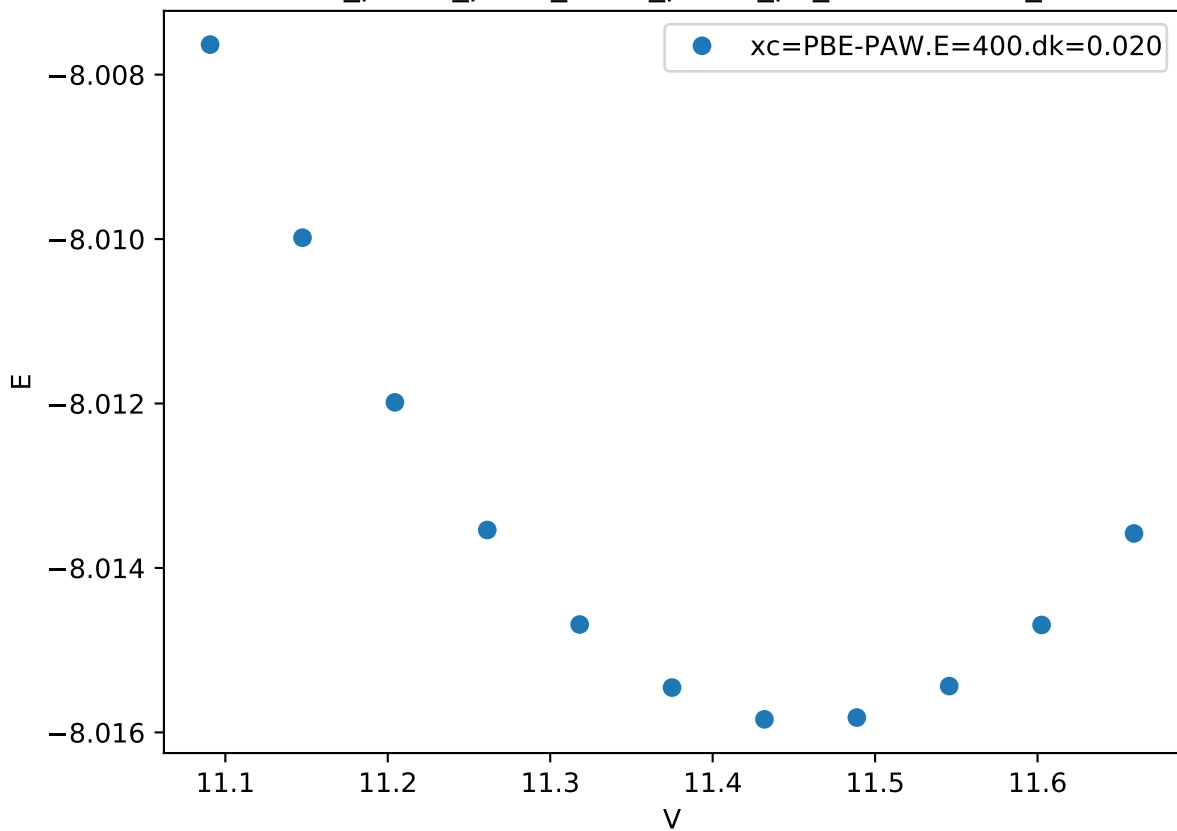
Cr_pv-Co_pv-W_sv/Cr_pv-Co_pv_C14-BBA.FM_
