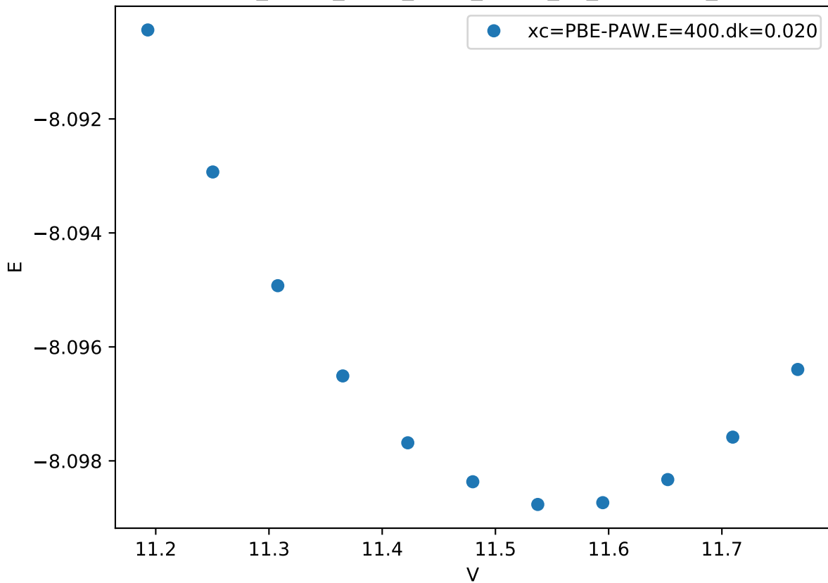
Cr_pv-Co_pv-W_sv/Cr_pv-Co_pv_B2-AB.FM_
