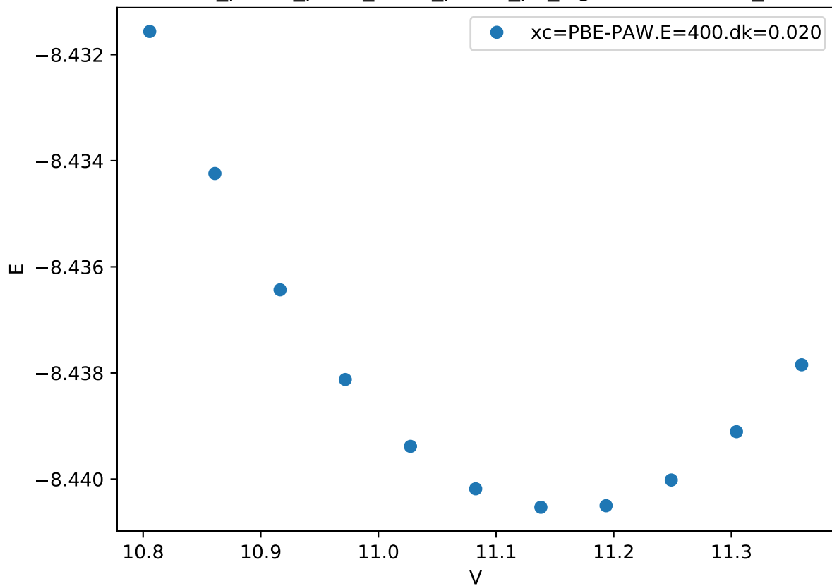
Cr_pv-Co_pv-W_sv/Cr_pv-Co_pv_sigma-ABABA.FM_
