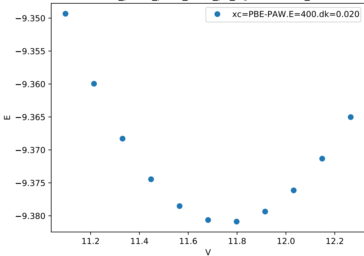
Cr_pv-Co_pv-W_sv/Cr_pv_sigma.UDUUD_
