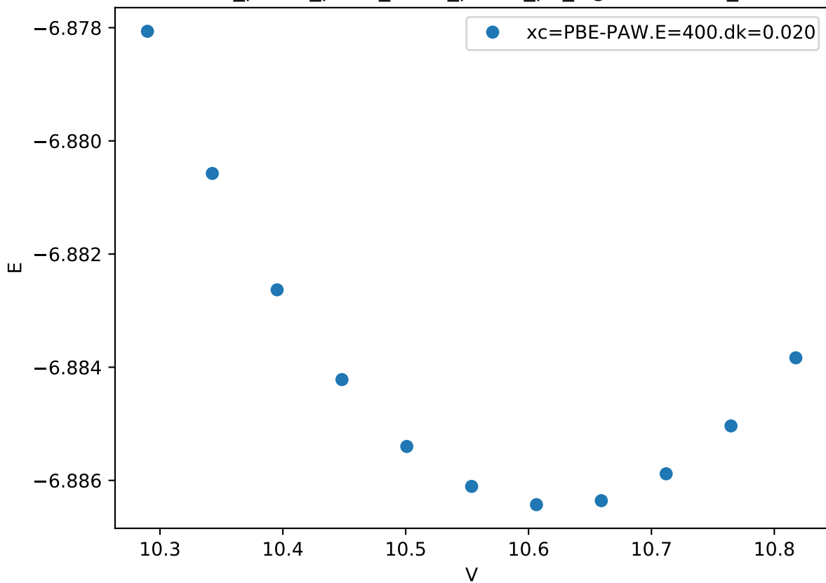
Cr_pv-Co_pv-W_sv/Cr_pv-Co_pv_sigma-ABBBB_
