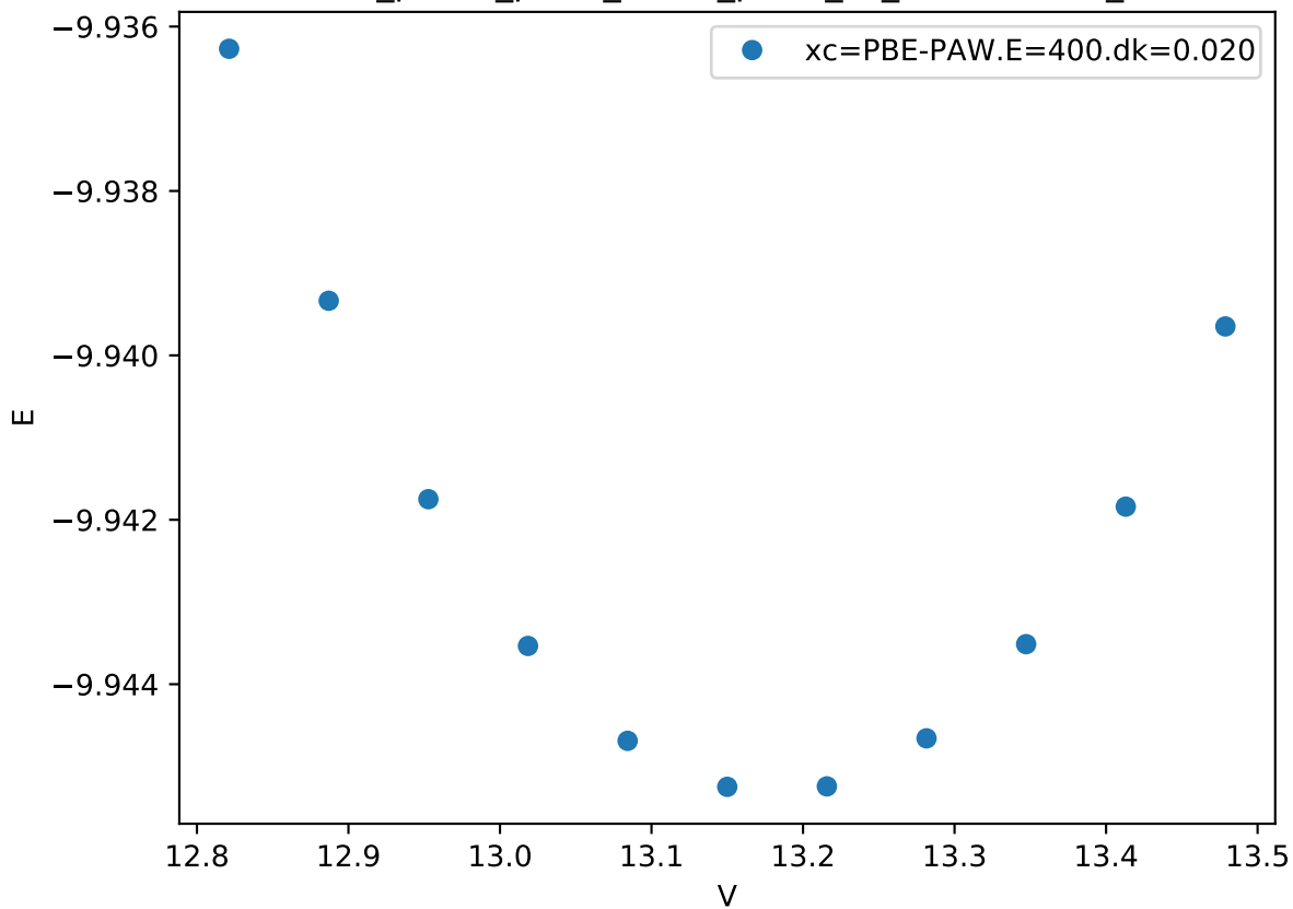
Cr_pv-Co_pv-W_sv/Co_pv-W_sv_L10-NiAl-AB_
