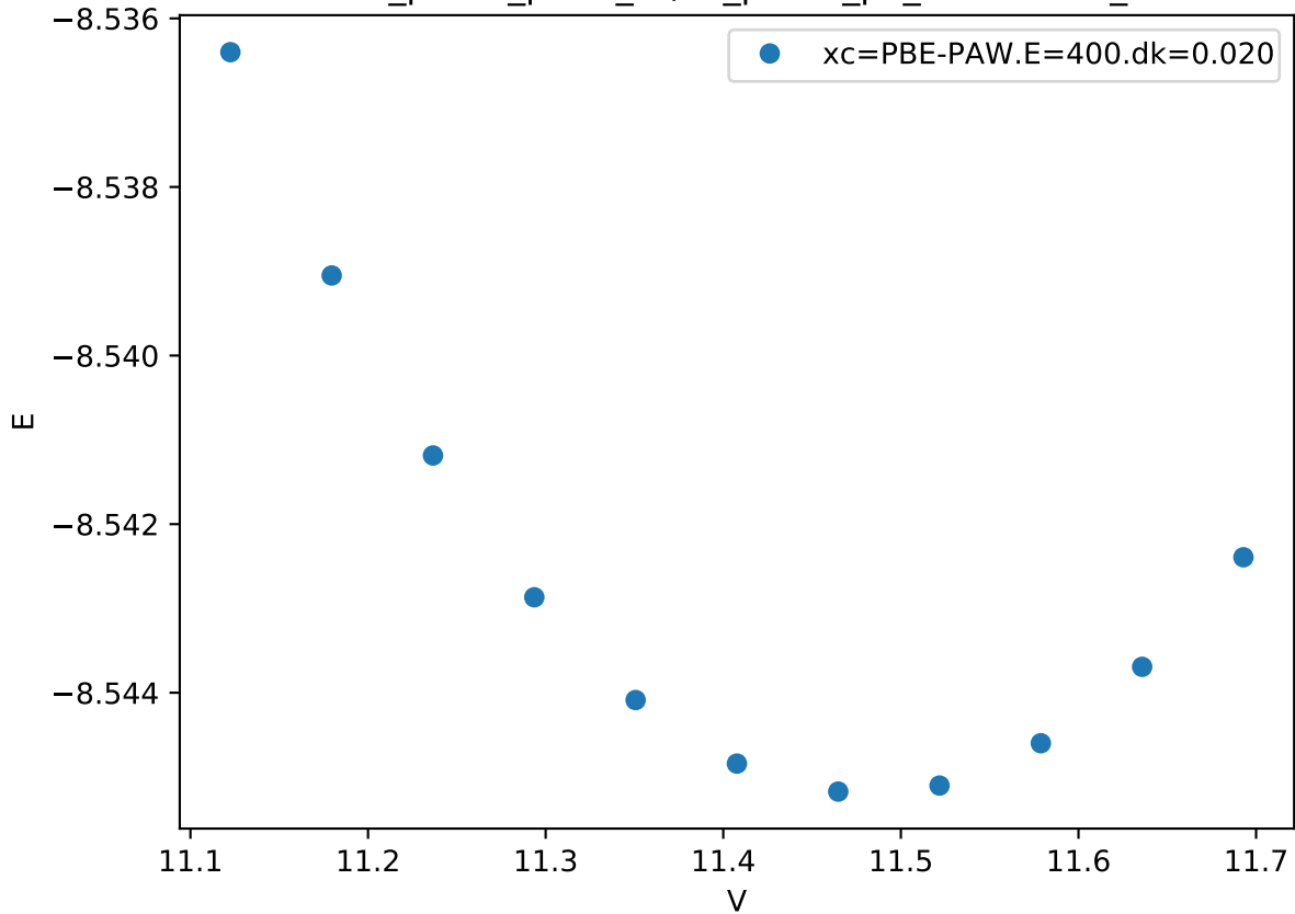
Cr_pv-Co_pv-W_sv/Cr_pv-Co_pv_mu-AAABB_
