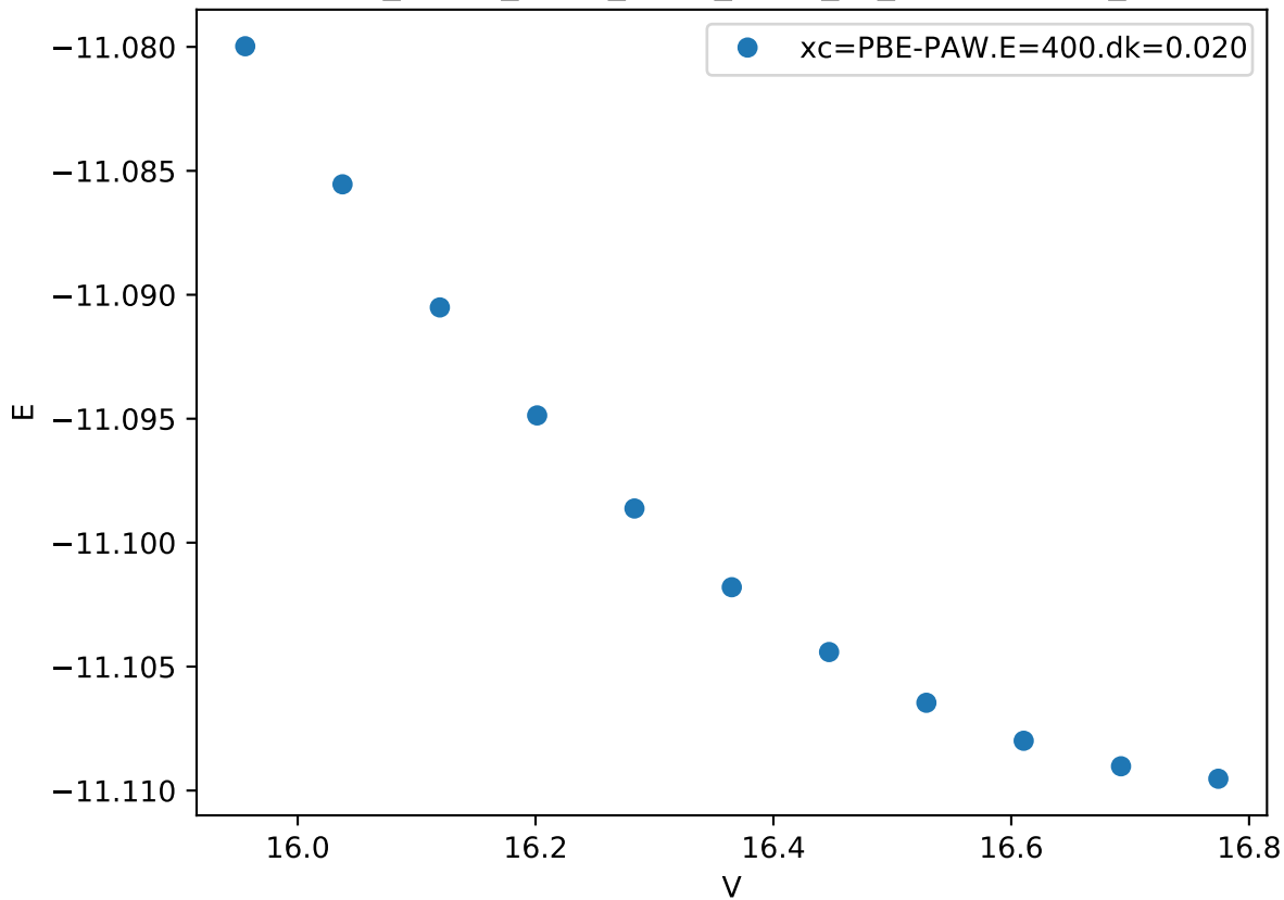
Cr_pv-Co_pv-W_sv/Cr_pv-W_sv_C14-ABB.FM_
