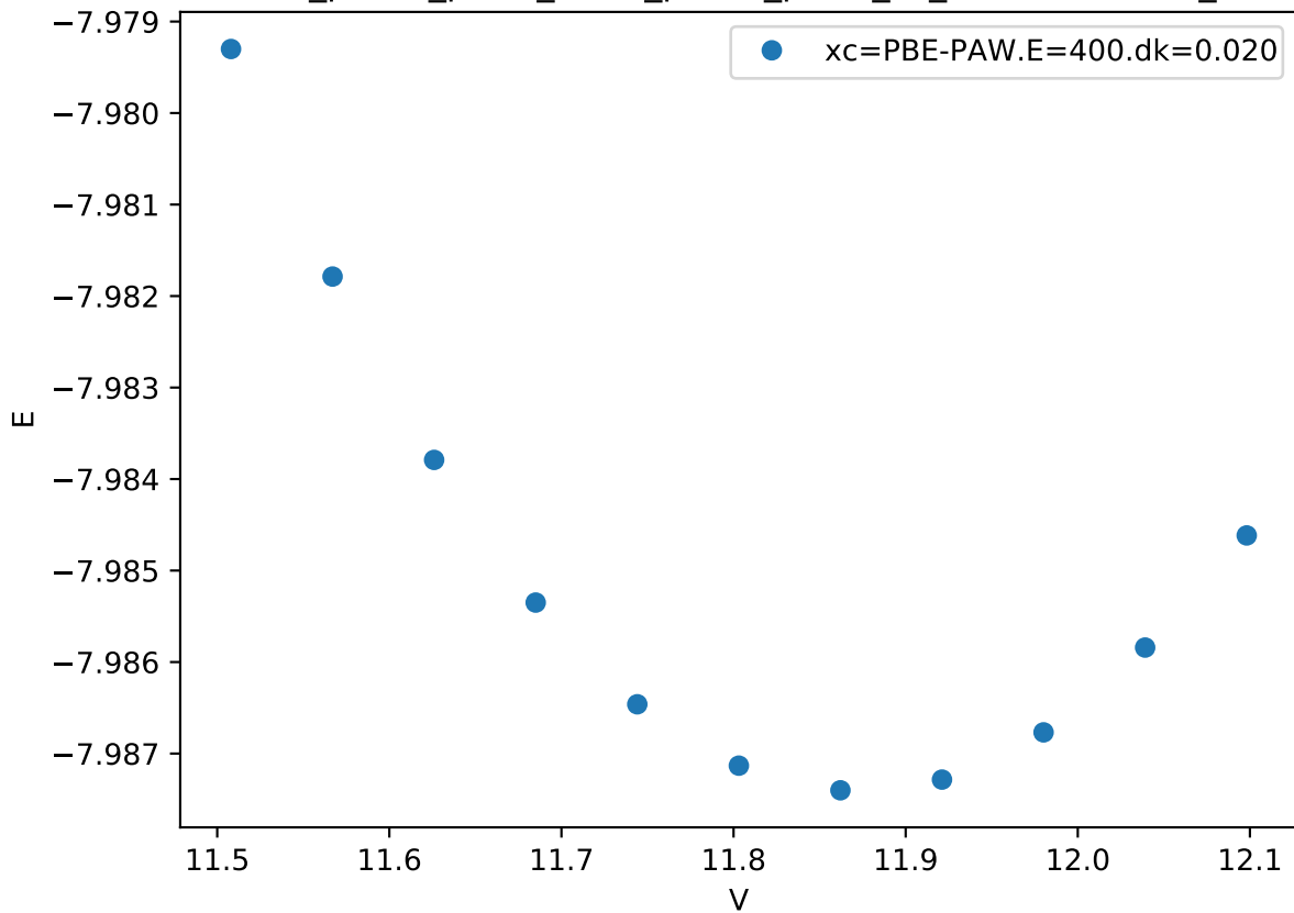
Cr_pv-Co_pv-W_sv/Cr_pv-Co_pv-W_sv_mu-ABCBB.FM_
