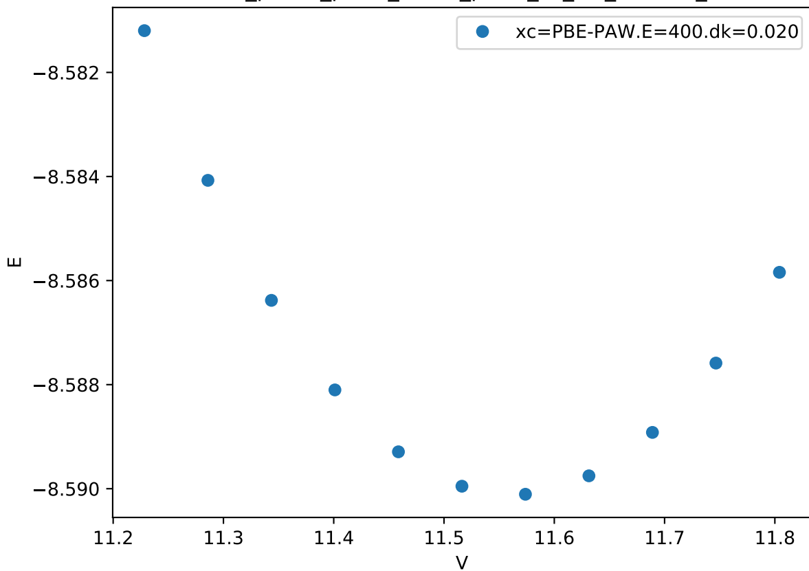
Cr_pv-Co_pv-W_sv/Co_pv-W_sv_D0_19-A3B_
