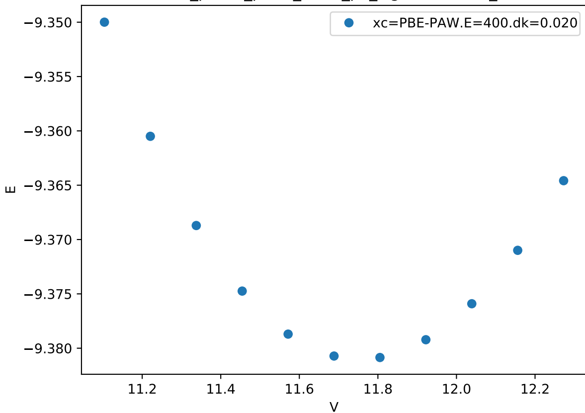
Cr_pv-Co_pv-W_sv/Cr_pv_sigma.UUUDU_
