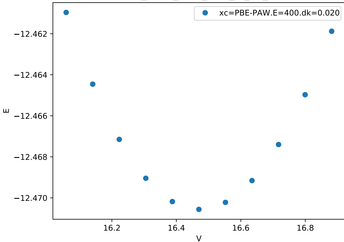
Cr_pv-Co_pv-W_sv/W_sv_fcc_
