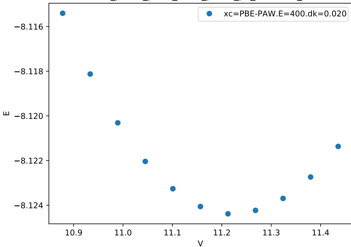
Cr_pv-Co_pv-W_sv/Cr_pv-Co_pv_C14-AAB_
