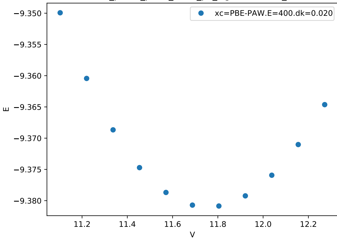
Cr_pv-Co_pv-W_sv/Cr_pv_sigma.UUDUD_
