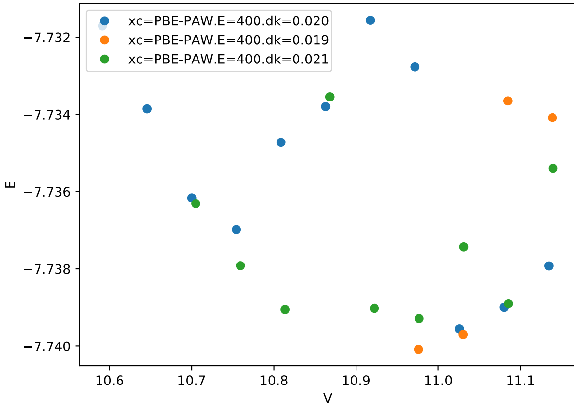
Cr_pv-Co_pv-W_sv/Cr_pv-Co_pv_sigma-ABABB.FM_
