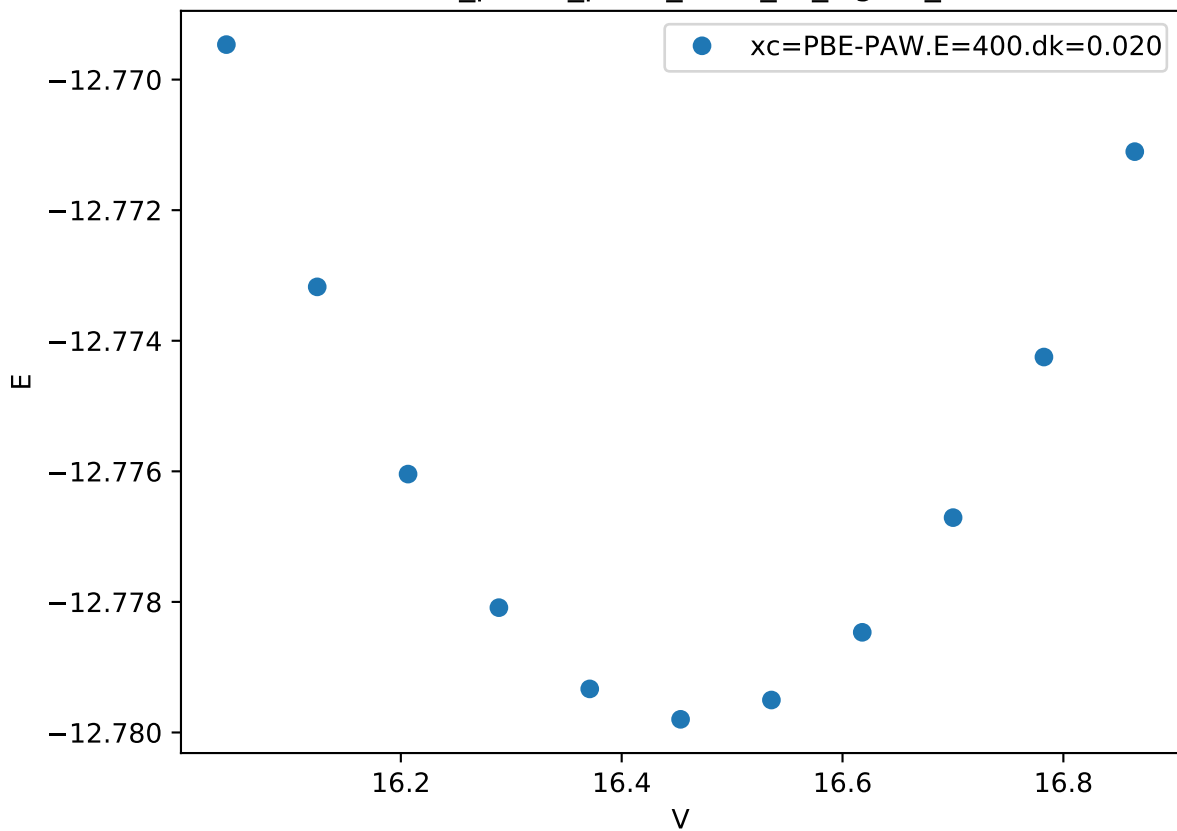
Cr_pv-Co_pv-W_sv/W_sv_sigma_
