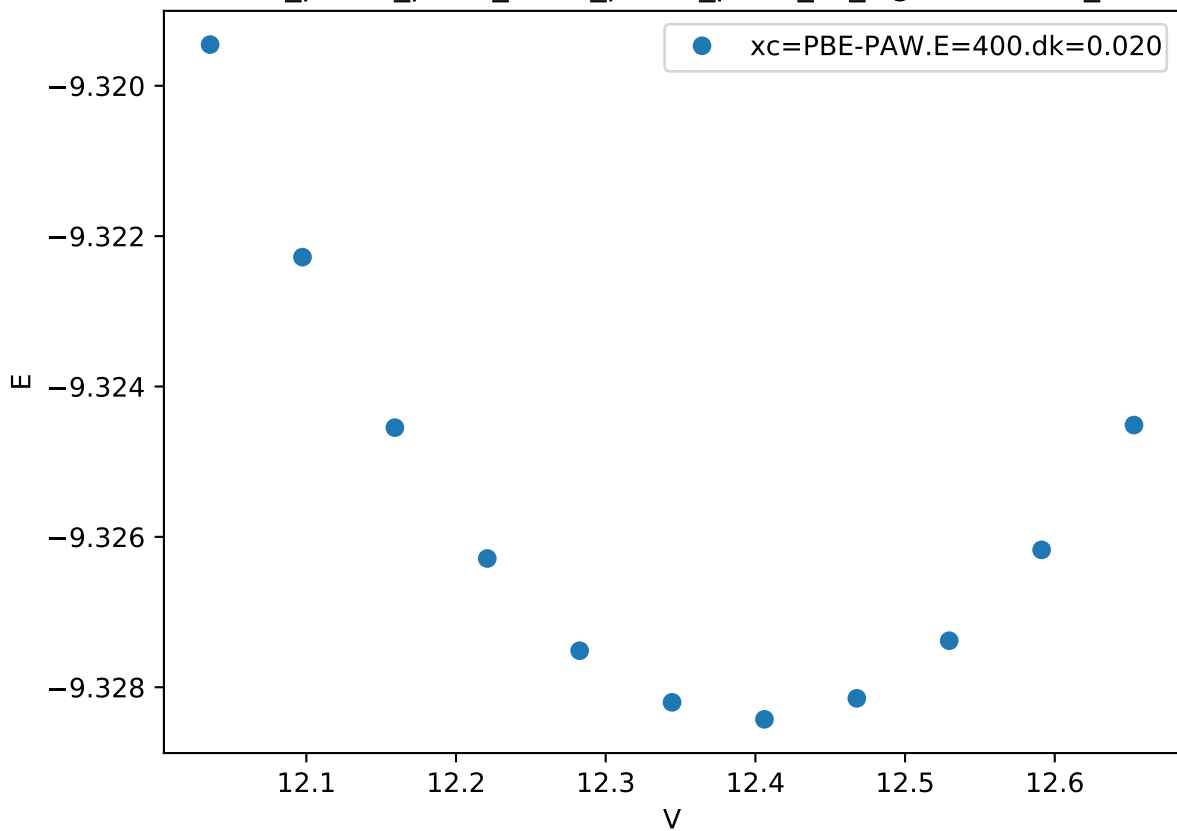
Cr_pv-Co_pv-W_sv/Cr_pv-Co_pv-W_sv_sigma-CCAAB_
