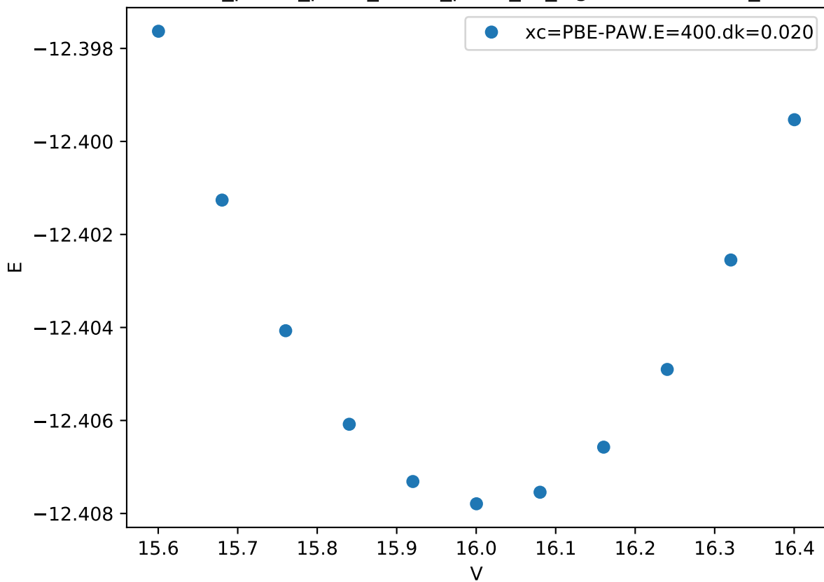
Cr_pv-Co_pv-W_sv/Co_pv-W_sv_sigma-ABBBB.FM_
