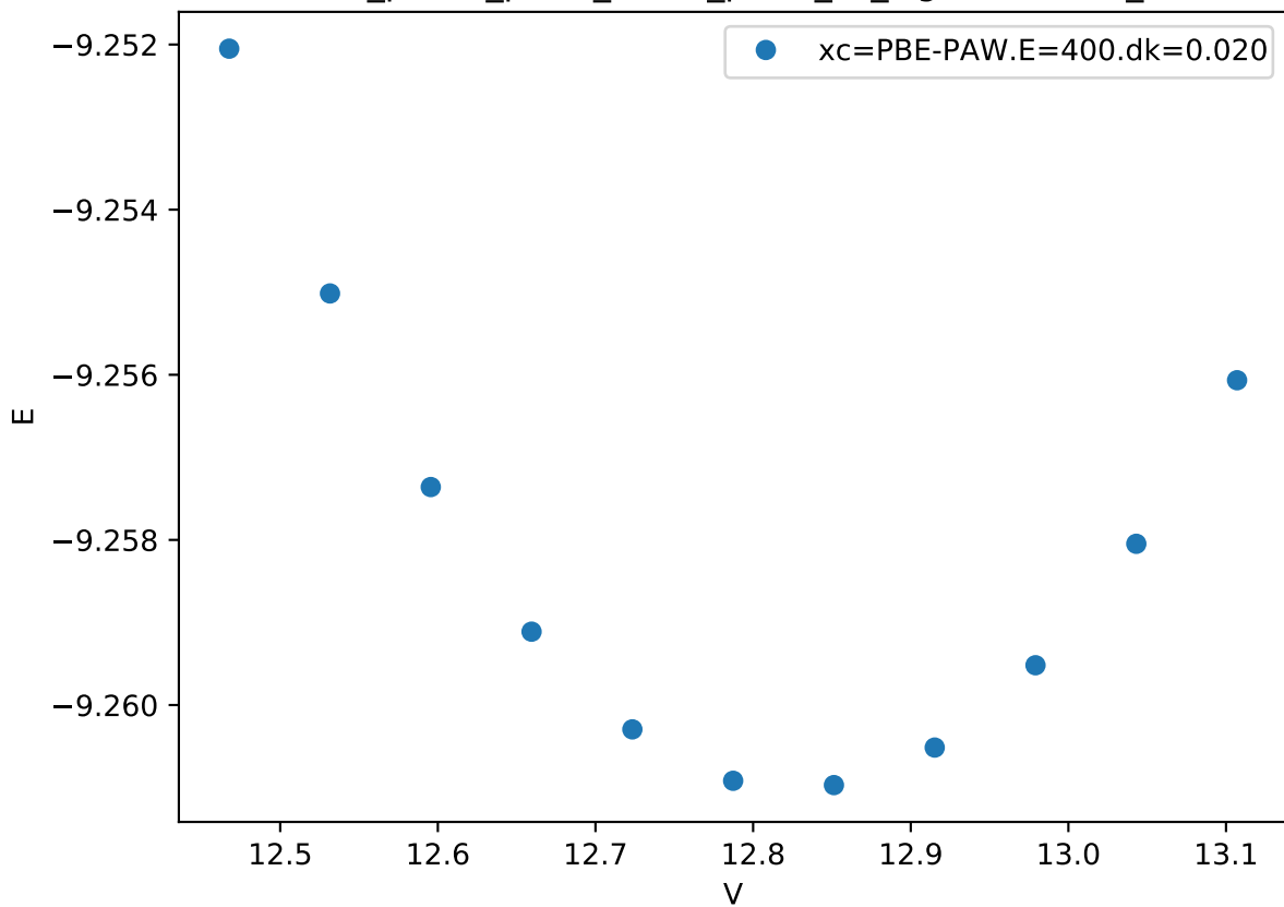
Cr_pv-Co_pv-W_sv/Co_pv-W_sv_sigma-ABAAB_
