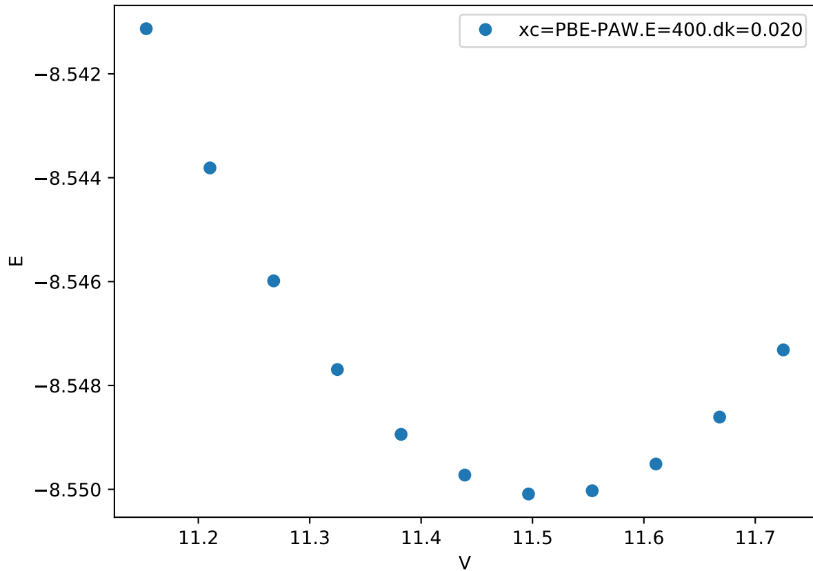
Cr_pv-Co_pv-W_sv/Cr_pv-Co_pv_mu-AABAB_
