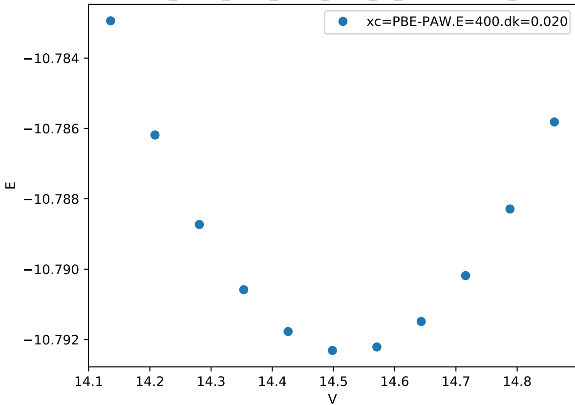
Cr_pv-Co_pv-W_sv/Co_pv-W_sv_sigma-ABABB_
