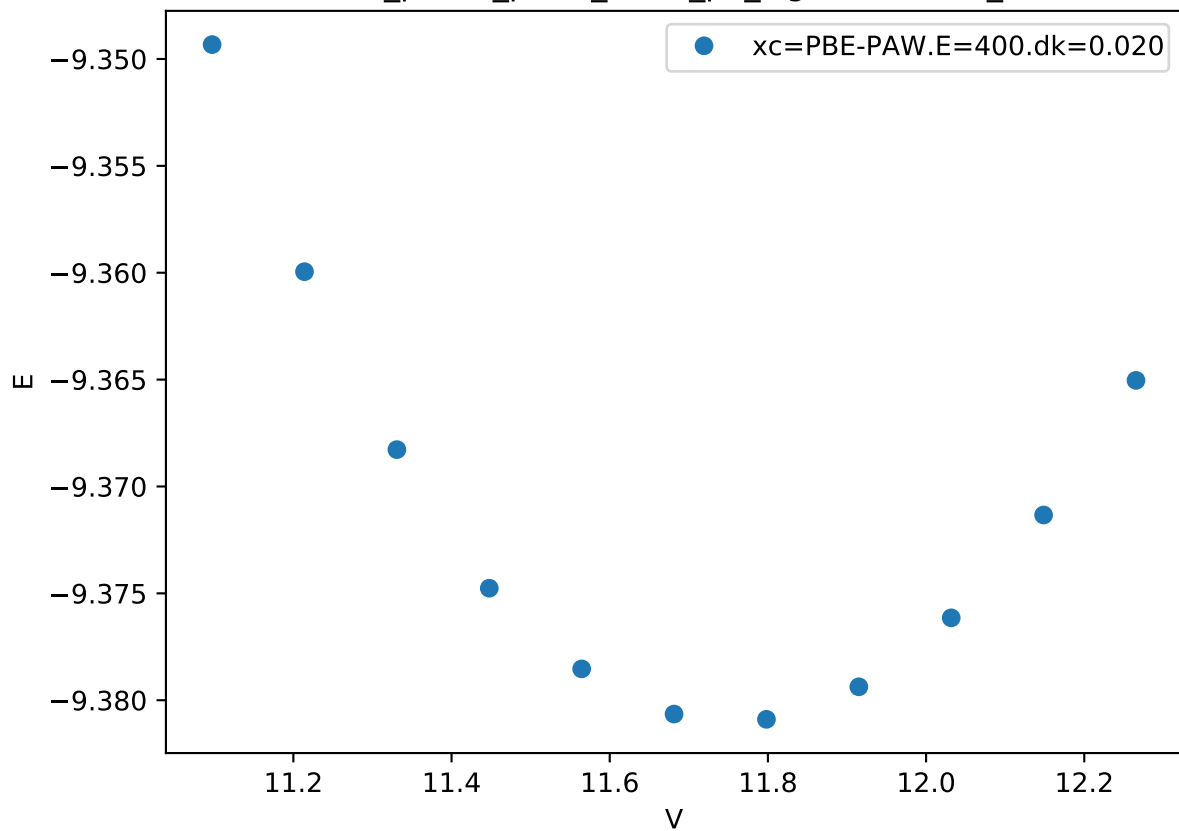
Cr_pv-Co_pv-W_sv/Cr_pv_sigma.UUDDU_
