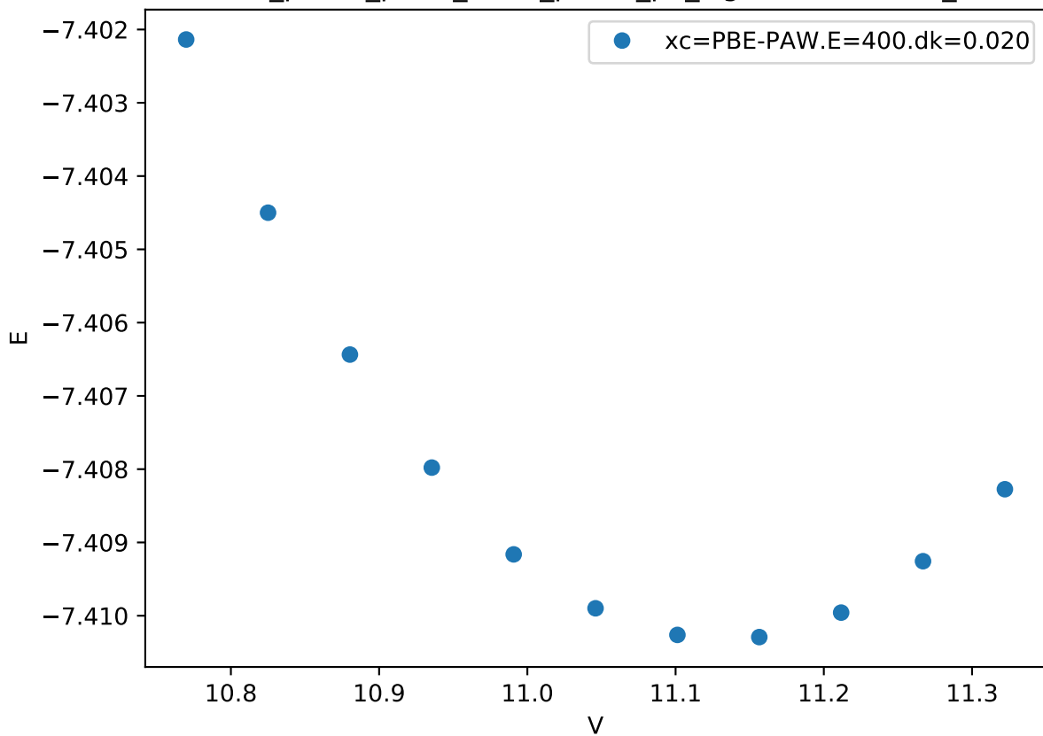
Cr_pv-Co_pv-W_sv/Cr_pv-Co_pv_sigma-AABBB.FM_
