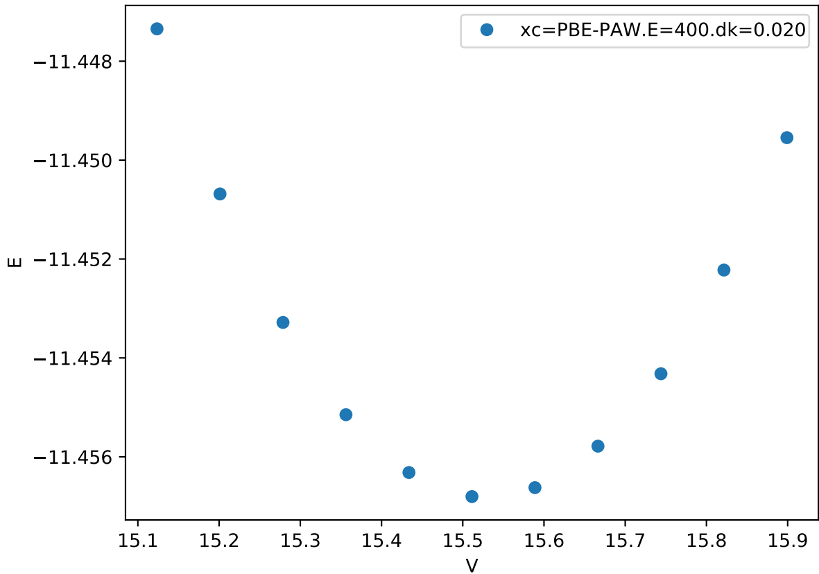
Cr_pv-Co_pv-W_sv/Co_pv-W_sv_sigma-AABBB_
