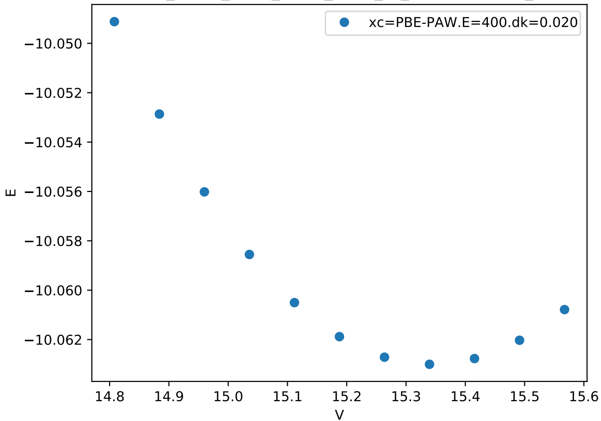
Cr_pv-Co_pv-W_sv/Co_pv-W_sv_mu-ABAAB.FM_
