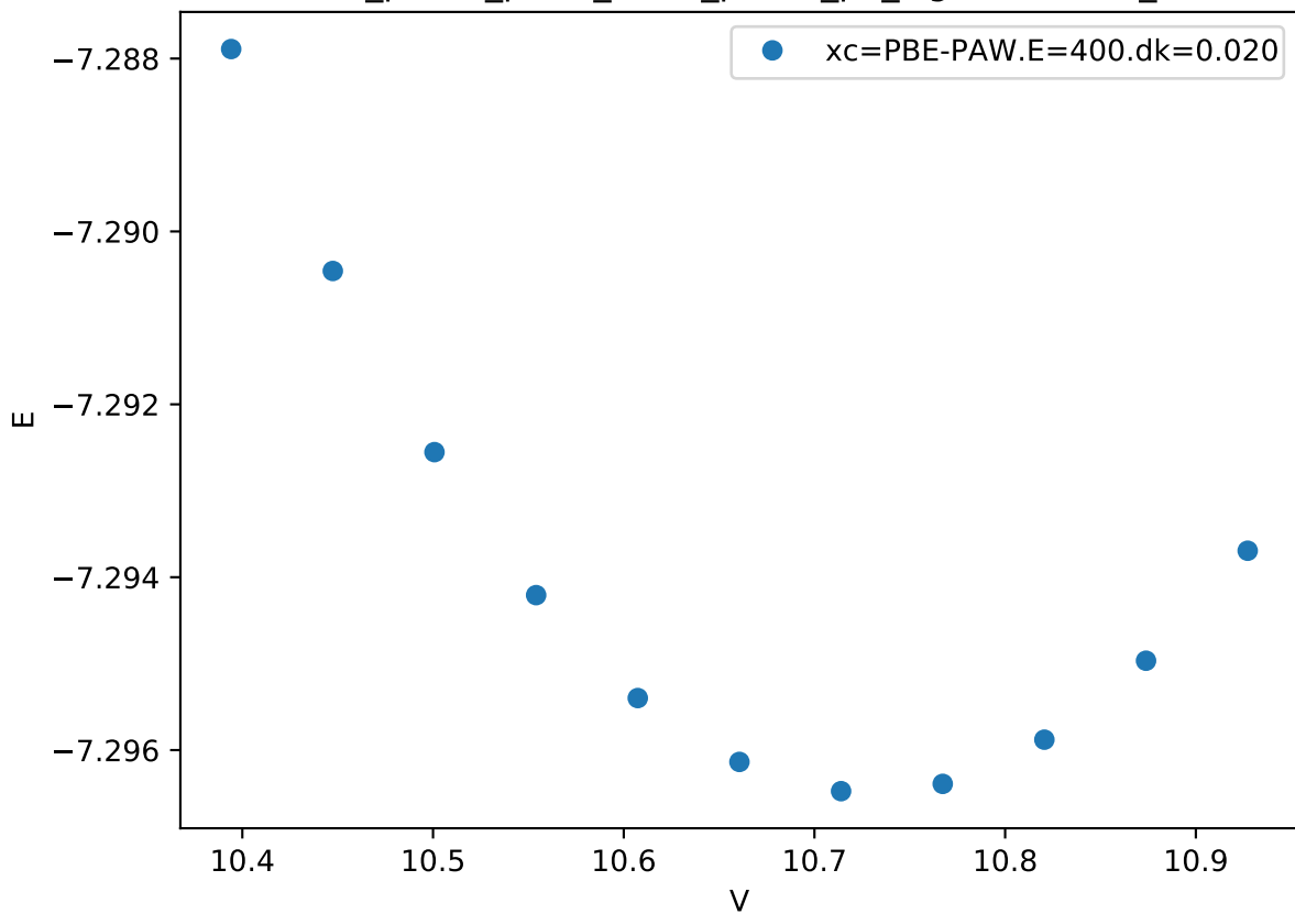
Cr_pv-Co_pv-W_sv/Cr_pv-Co_pv_sigma-AABBB_
