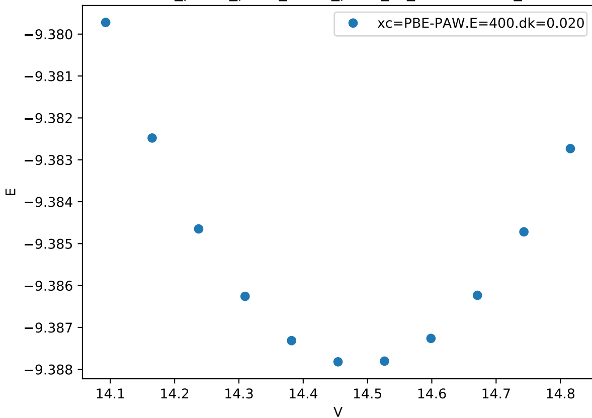
Cr_pv-Co_pv-W_sv/Co_pv-W_sv_C14-AAB.FM_
