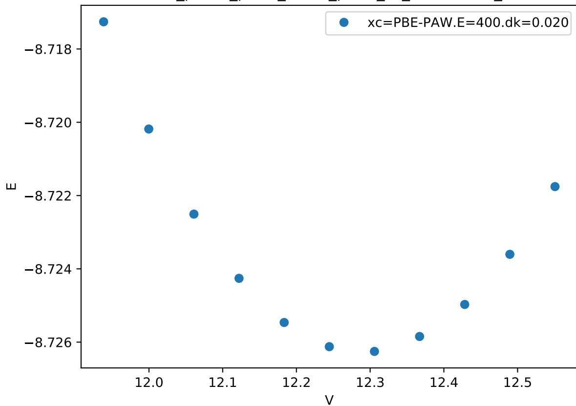
Cr_pv-Co_pv-W_sv/Co_pv-W_sv_mu-AABAB_
