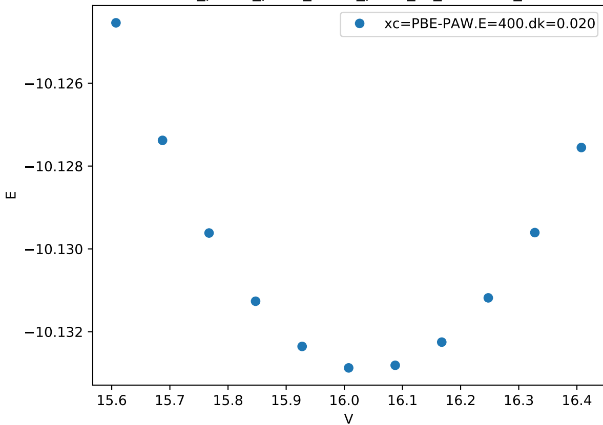
Cr_pv-Co_pv-W_sv/Co_pv-W_sv_C14-ABB_
