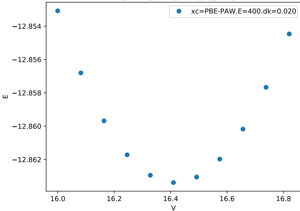
Cr_pv-Co_pv-W_sv/W_sv_A15_
