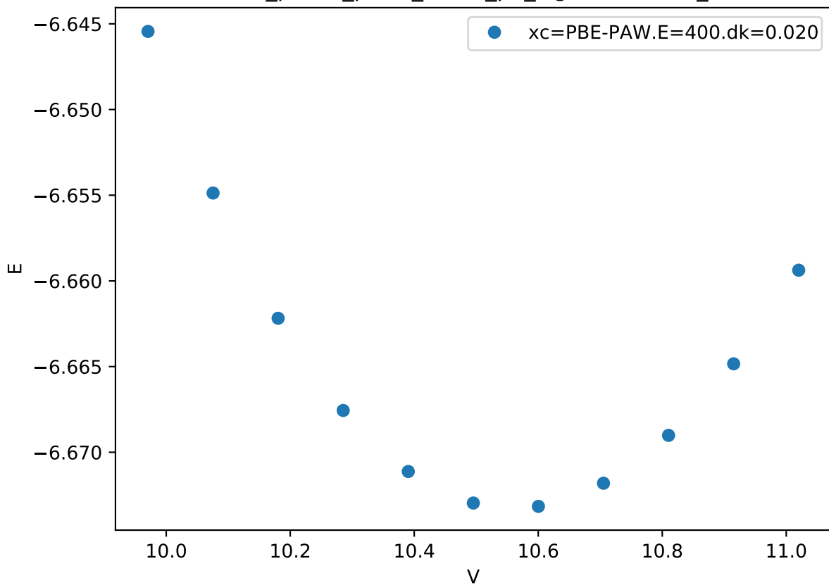
Cr_pv-Co_pv-W_sv/Co_pv_sigma.DDDDU_
