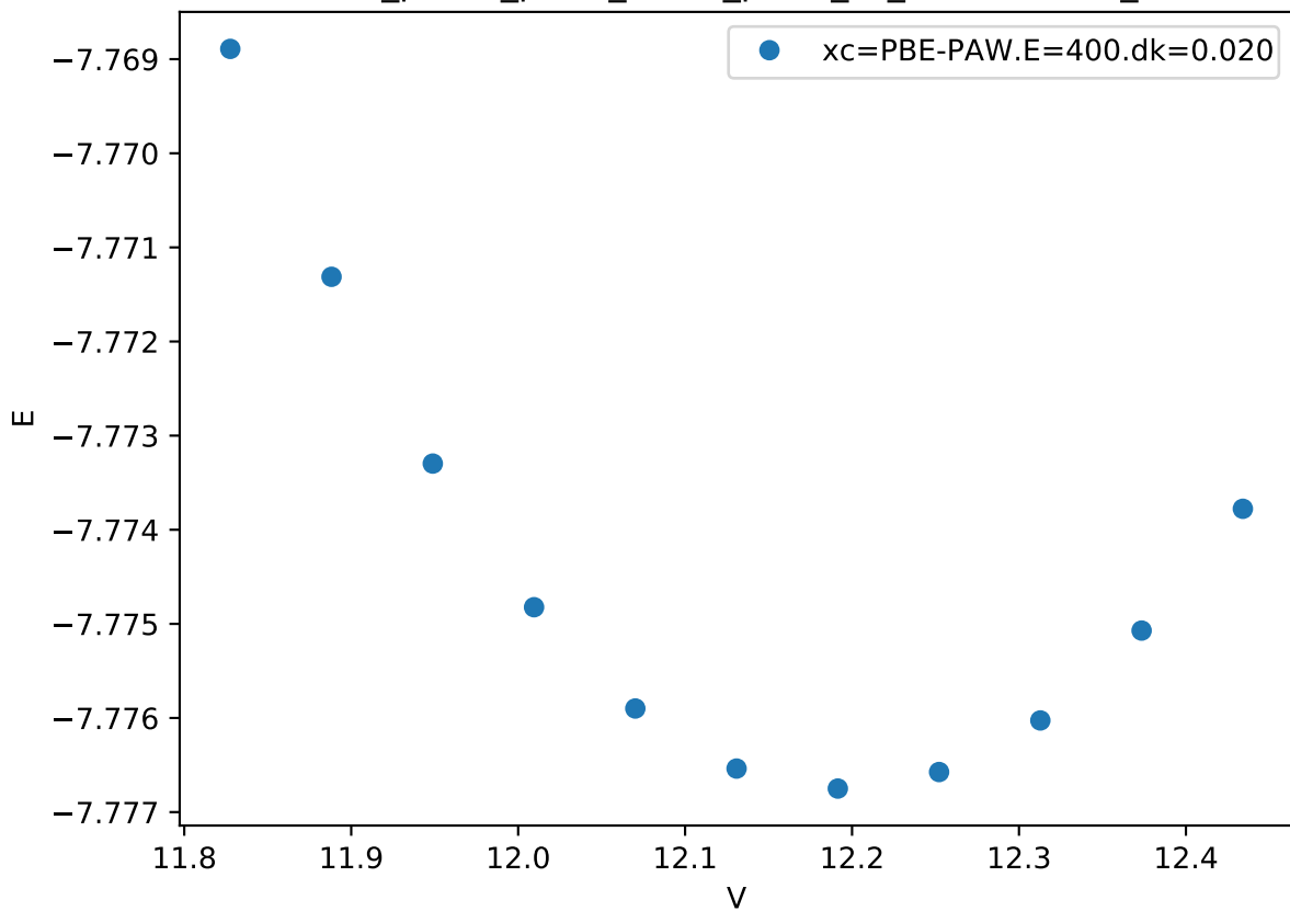
Cr_pv-Co_pv-W_sv/Co_pv-W_sv_C14-ABA.FM_
