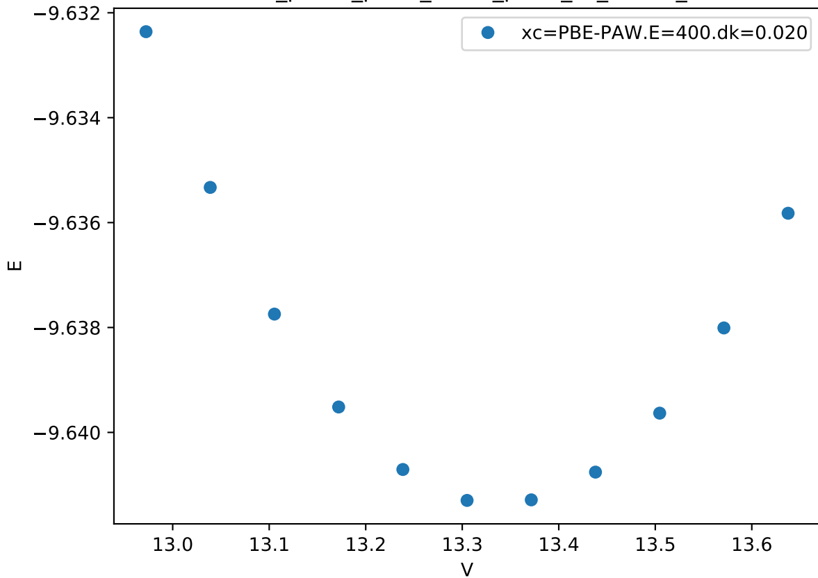
Cr_pv-Co_pv-W_sv/Co_pv-W_sv_B2-AB_
