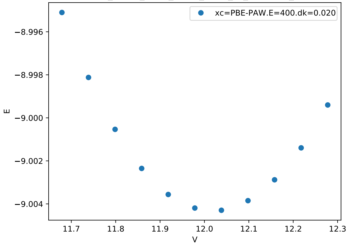
Cr_pv-Co_pv-W_sv/Co_pv-W_sv_C14-BAA_
