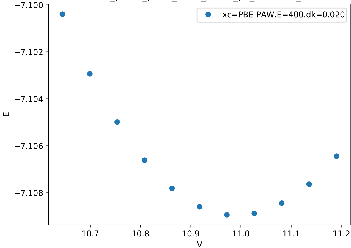
Cr_pv-Co_pv-W_sv/Cr_pv-Co_pv_C14-BAB_
