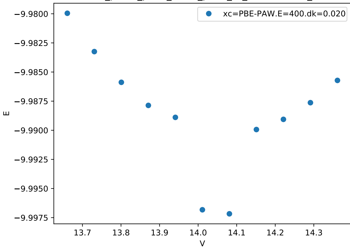
Cr_pv-Co_pv-W_sv/Co_pv-W_sv_chi-ABAB.FM_
