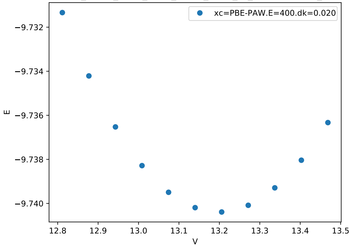
Cr_pv-Co_pv-W_sv/Cr_pv-Co_pv-W_sv_sigma-ABACA_
