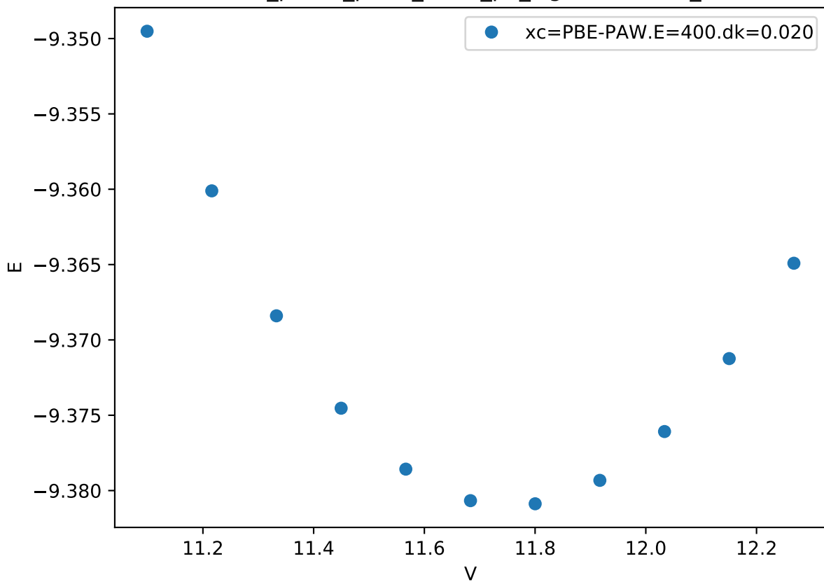
Cr_pv-Co_pv-W_sv/Cr_pv_sigma.DDUDU_
