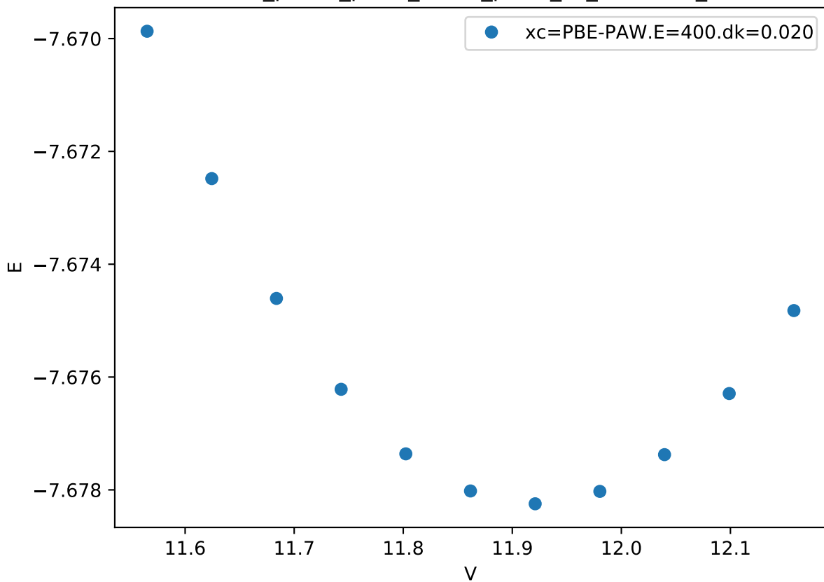
Cr_pv-Co_pv-W_sv/Co_pv-W_sv_C14-ABA_
