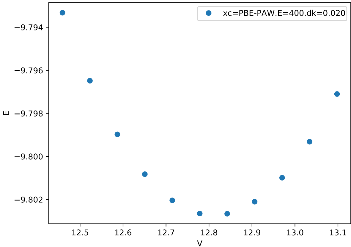
Cr_pv-Co_pv-W_sv/Co_pv-W_sv_mu-AABBB_
