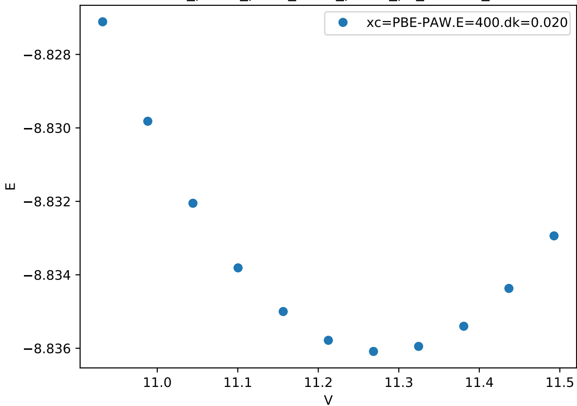
Cr_pv-Co_pv-W_sv/Cr_pv-Co_pv_A15-AB_
