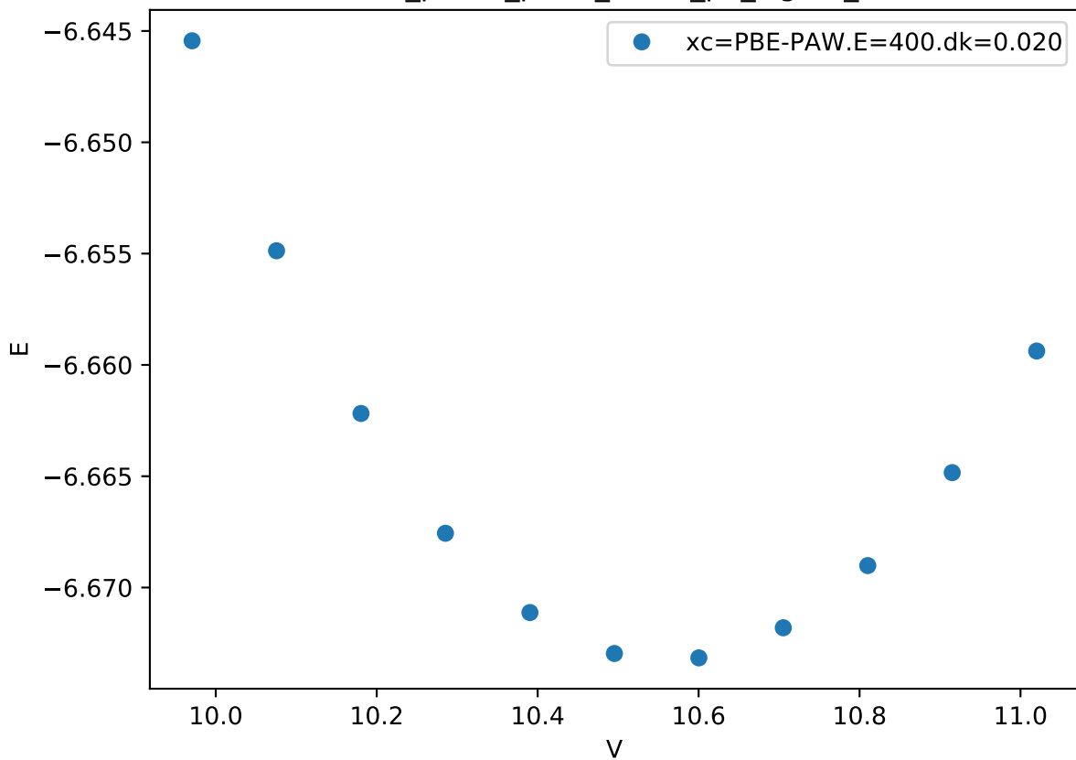
Cr_pv-Co_pv-W_sv/Co_pv_sigma_
