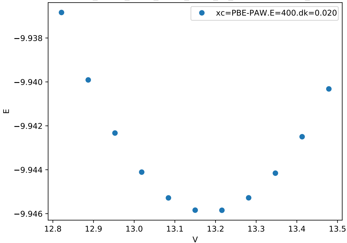
Cr_pv-Co_pv-W_sv/Co_pv-W_sv_L10-NiAl-AB.FM_
