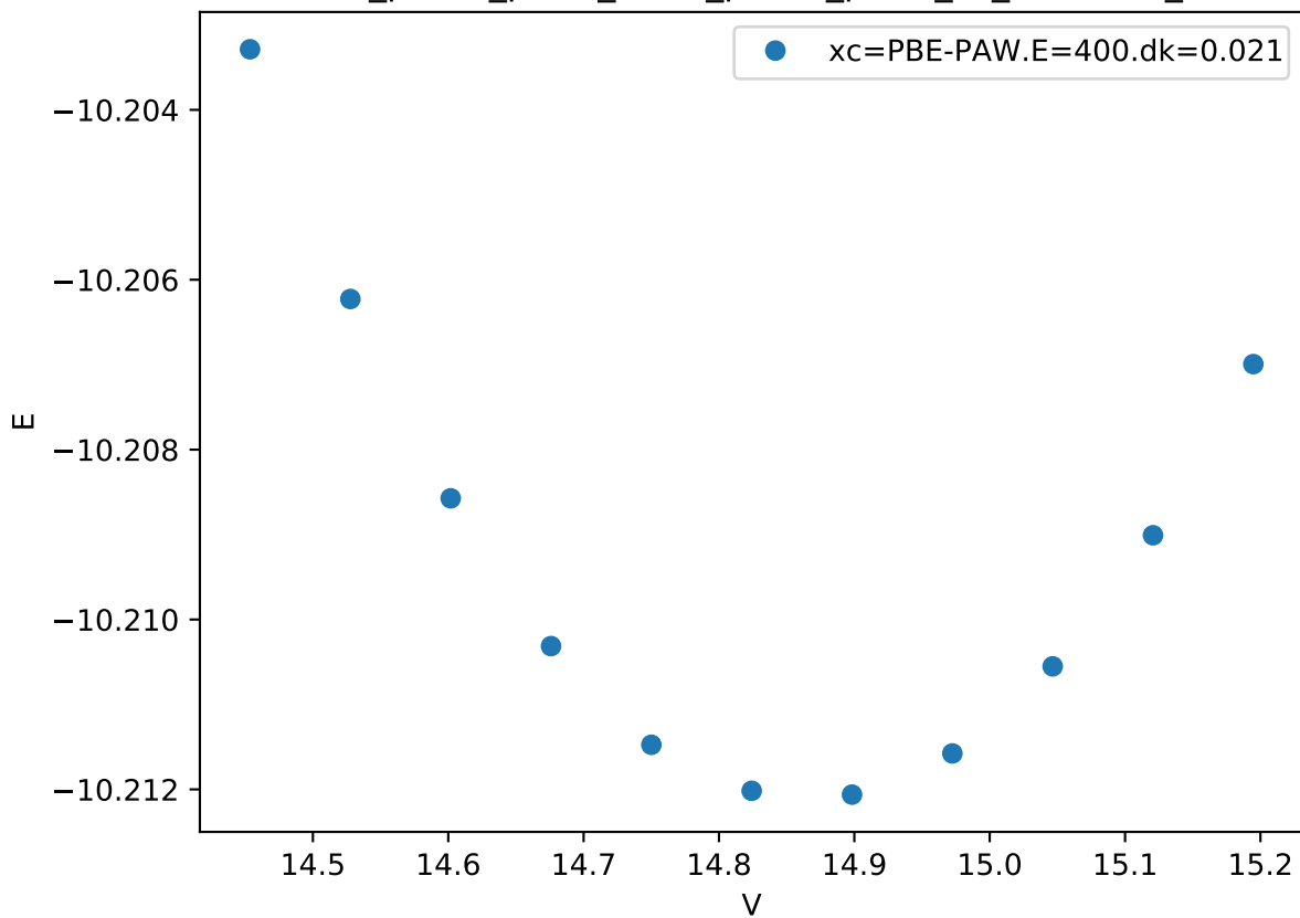
Cr_pv-Co_pv-W_sv/Cr_pv-Co_pv-W_sv_C14-BCA_
