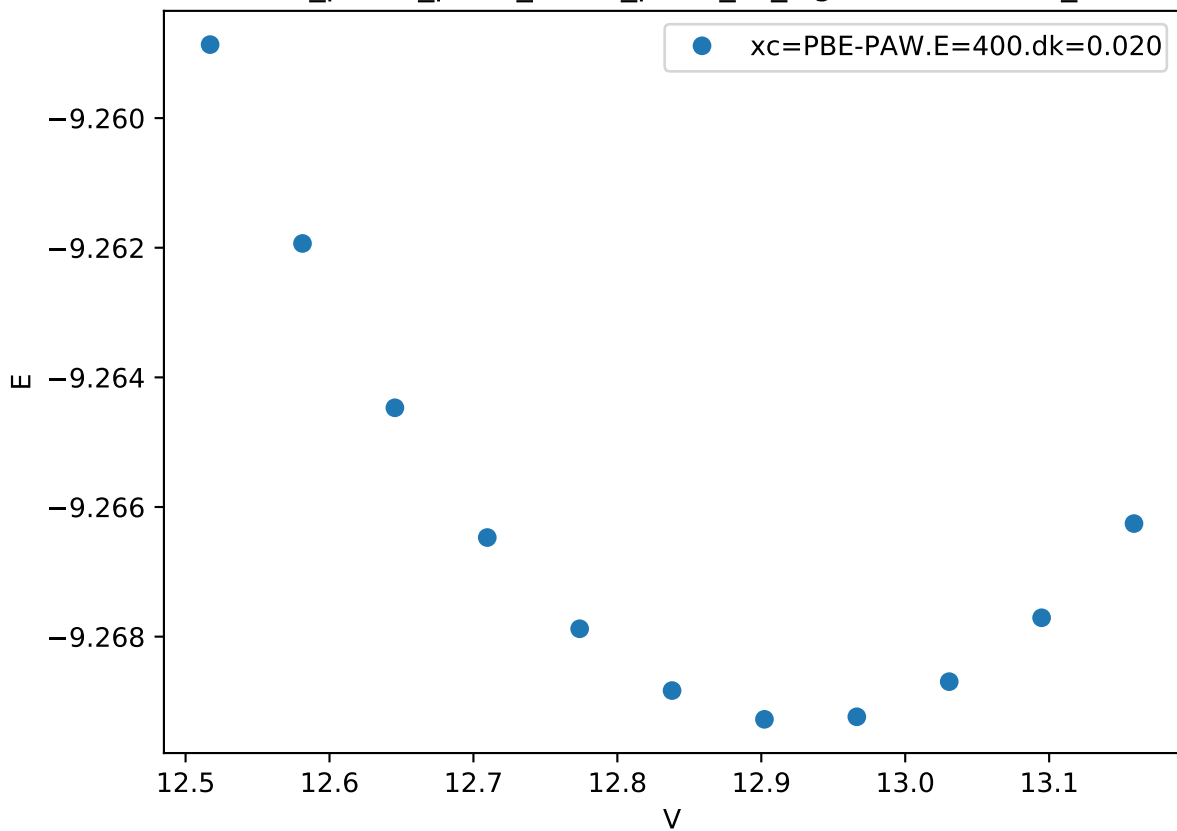
Cr_pv-Co_pv-W_sv/Co_pv-W_sv_sigma-ABABA.FM_
