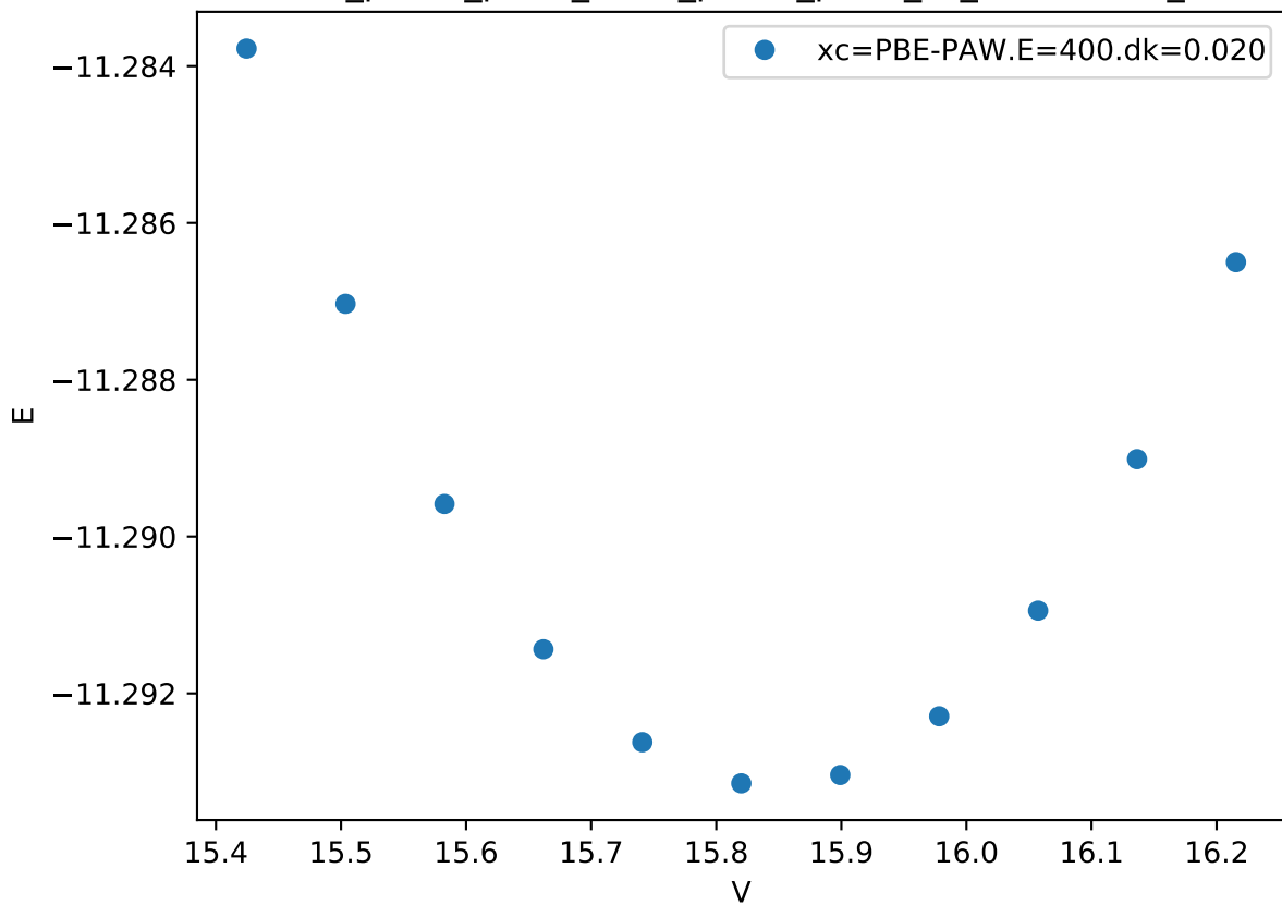
Cr_pv-Co_pv-W_sv/Cr_pv-Co_pv-W_sv_mu-ACCBC_
