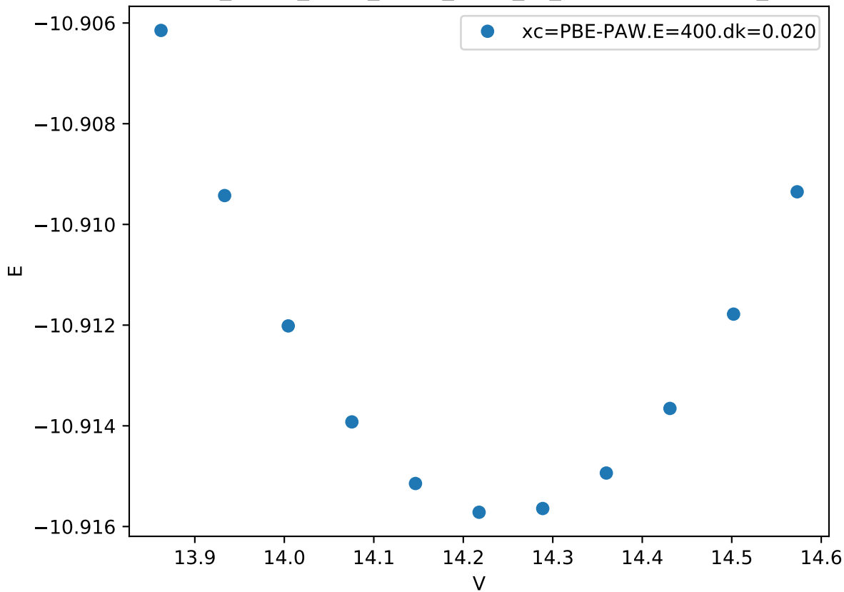
Cr_pv-Co_pv-W_sv/Co_pv-W_sv_sigma-ABBAB.FM_
