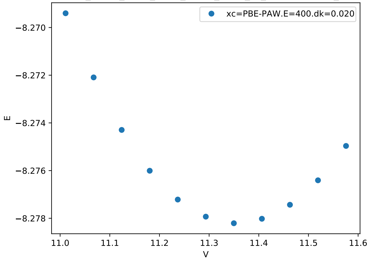
Cr_pv-Co_pv-W_sv/Cr_pv-Co_pv-W_sv_sigma-CAABB_
