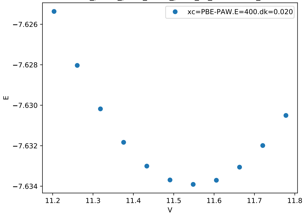
Cr_pv-Co_pv-W_sv/Co_pv-W_sv_mu-AABAA_
