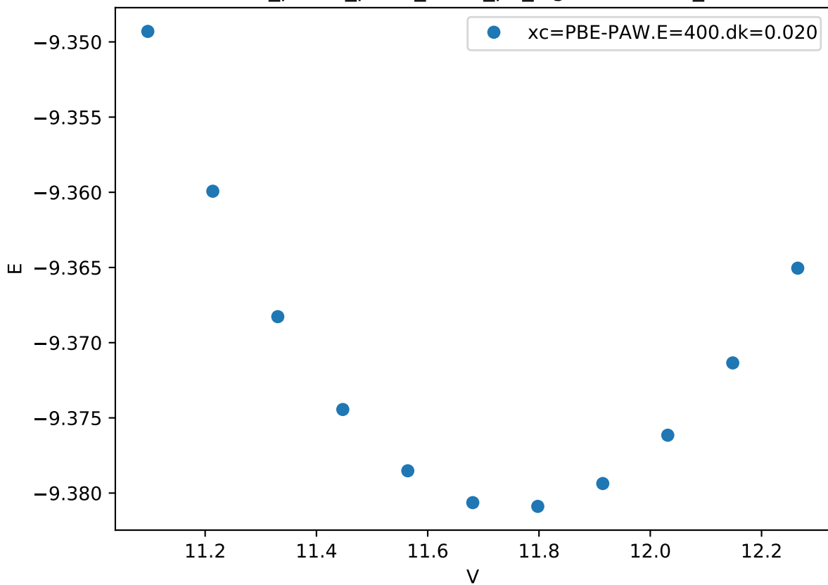
Cr_pv-Co_pv-W_sv/Cr_pv_sigma.DUUUD_
