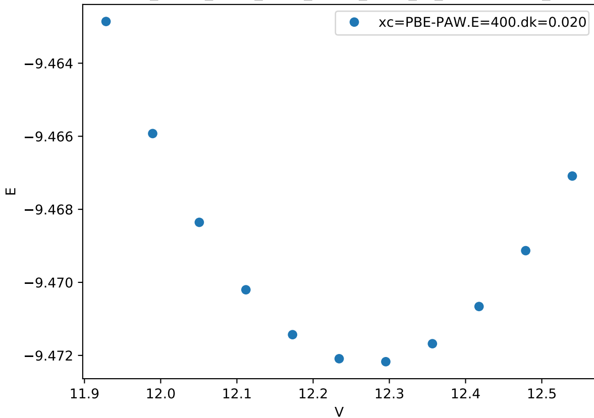
Cr_pv-Co_pv-W_sv/Cr_pv-Co_pv-W_sv_C14-ABC.FM_
