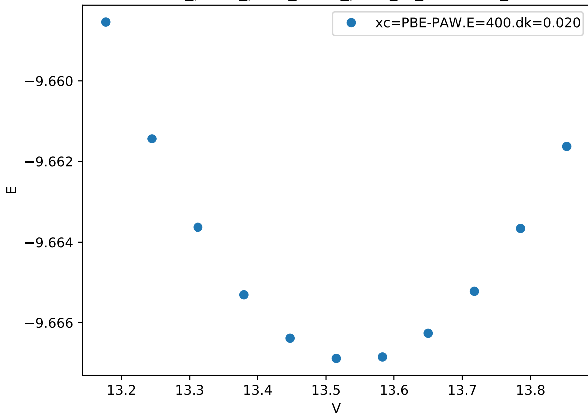
Cr_pv-Co_pv-W_sv/Co_pv-W_sv_B2-AB.FM_
