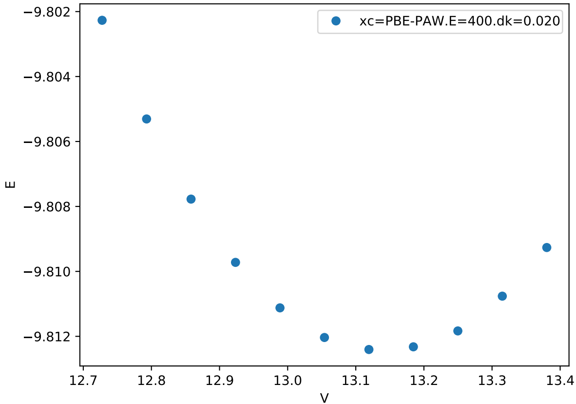
Cr_pv-Co_pv-W_sv/Cr_pv-Co_pv-W_sv_sigma-ABAAC.FM_
