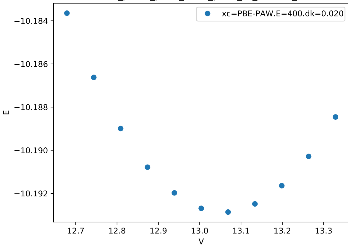
Cr_pv-Co_pv-W_sv/Cr_pv-W_sv_A15-AB_
