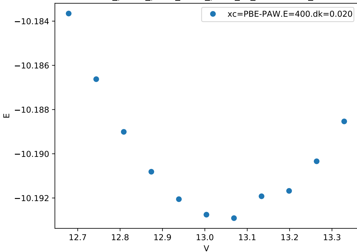
Cr_pv-Co_pv-W_sv/Cr_pv-W_sv_A15-AB.FM_
