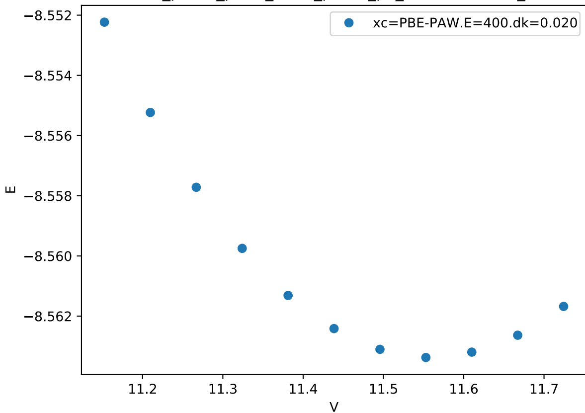
Cr_pv-Co_pv-W_sv/Cr_pv-Co_pv_mu-AABAB.FM_
