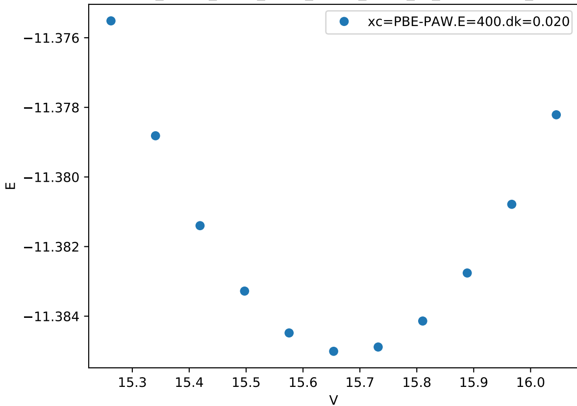
Cr_pv-Co_pv-W_sv/Cr_pv-Co_pv-W_sv_mu-ACCCB_
