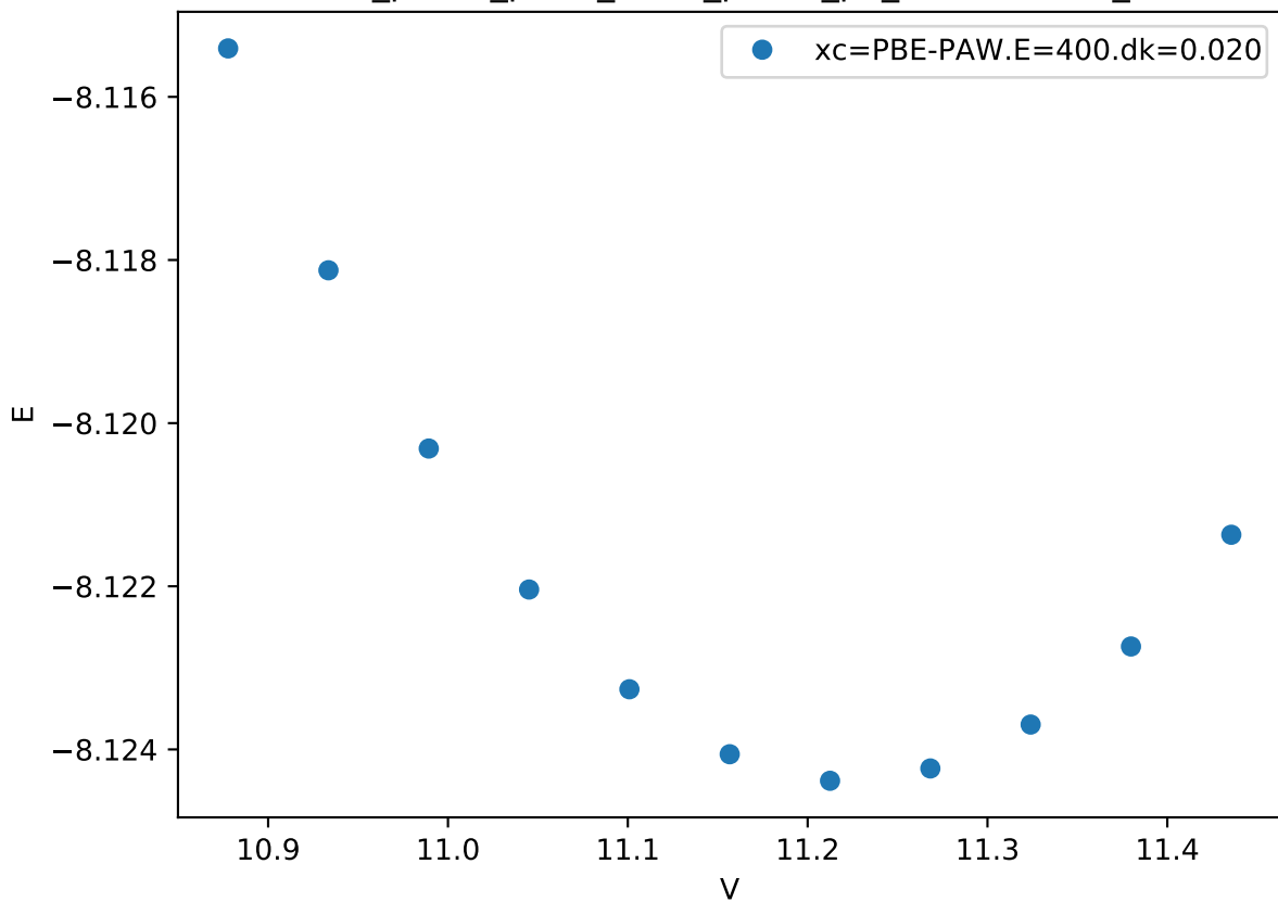
Cr_pv-Co_pv-W_sv/Cr_pv-Co_pv_C14-AAB.FM_
