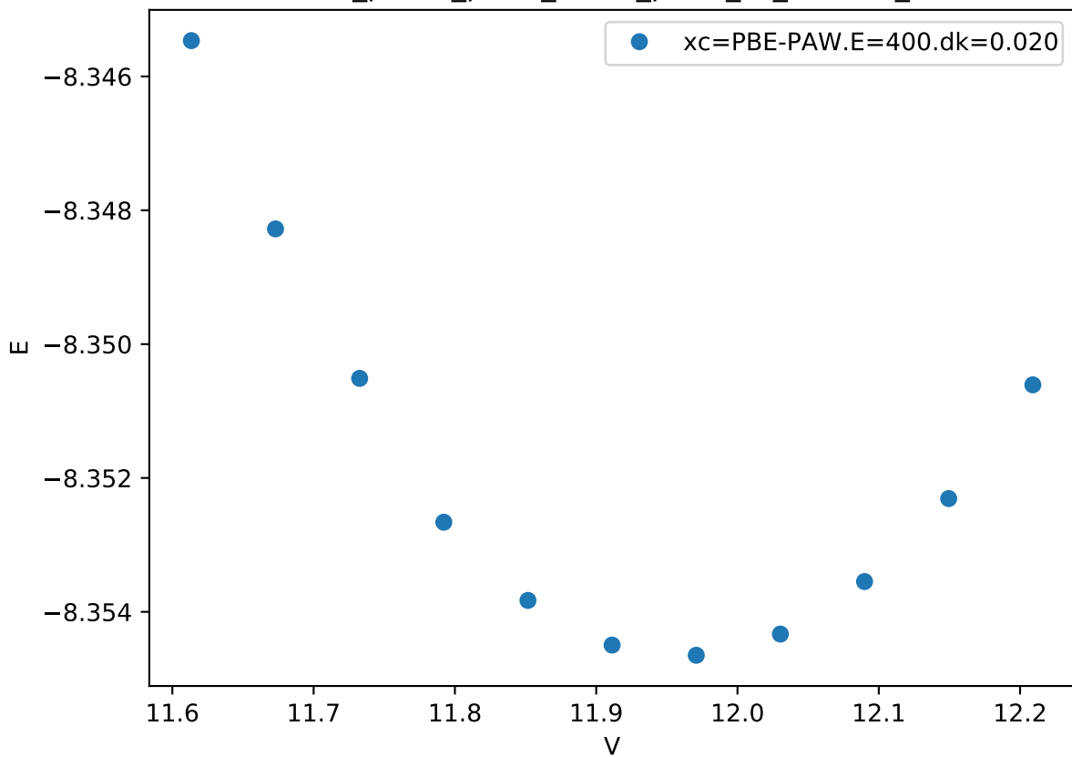
Cr_pv-Co_pv-W_sv/Co_pv-W_sv_A15-AB_
