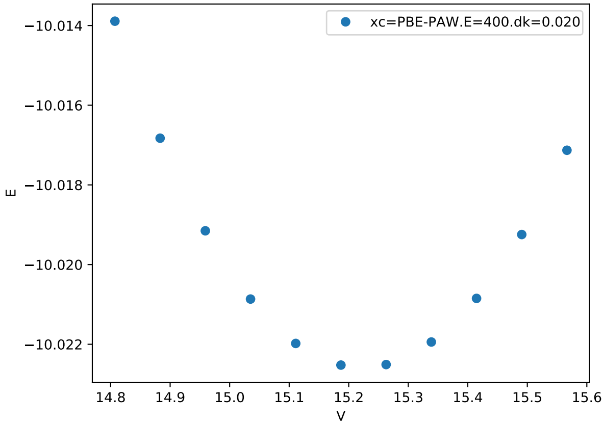
Cr_pv-Co_pv-W_sv/Co_pv-W_sv_mu-ABAAB_
