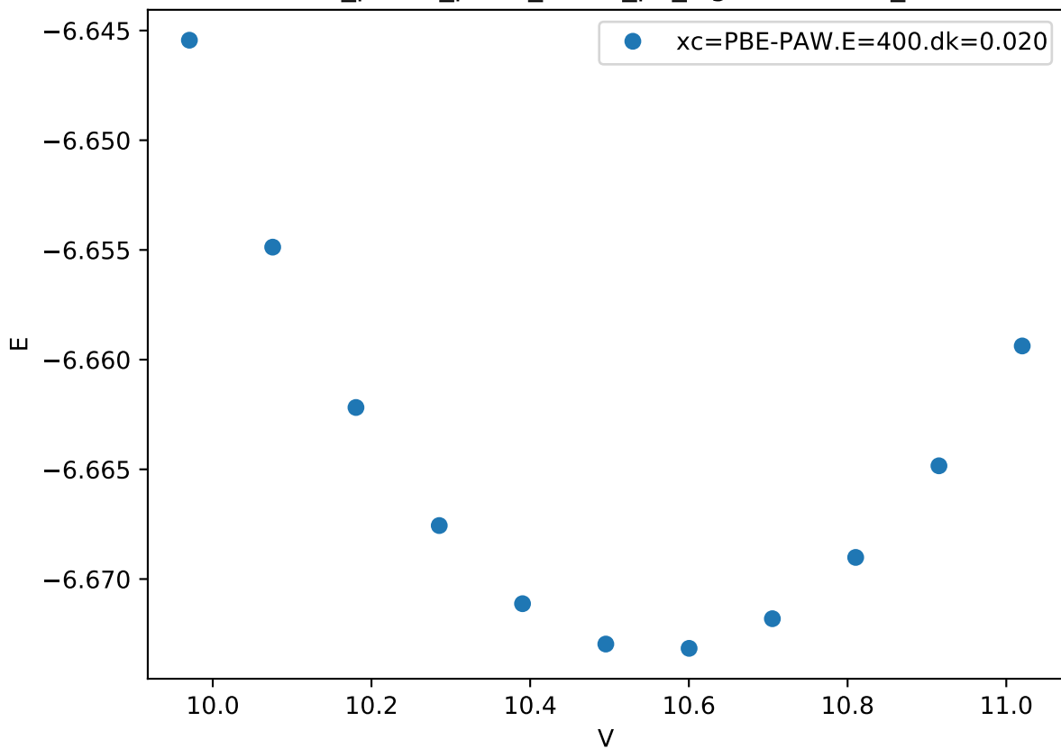
Cr_pv-Co_pv-W_sv/Co_pv_sigma.DDUUU_
