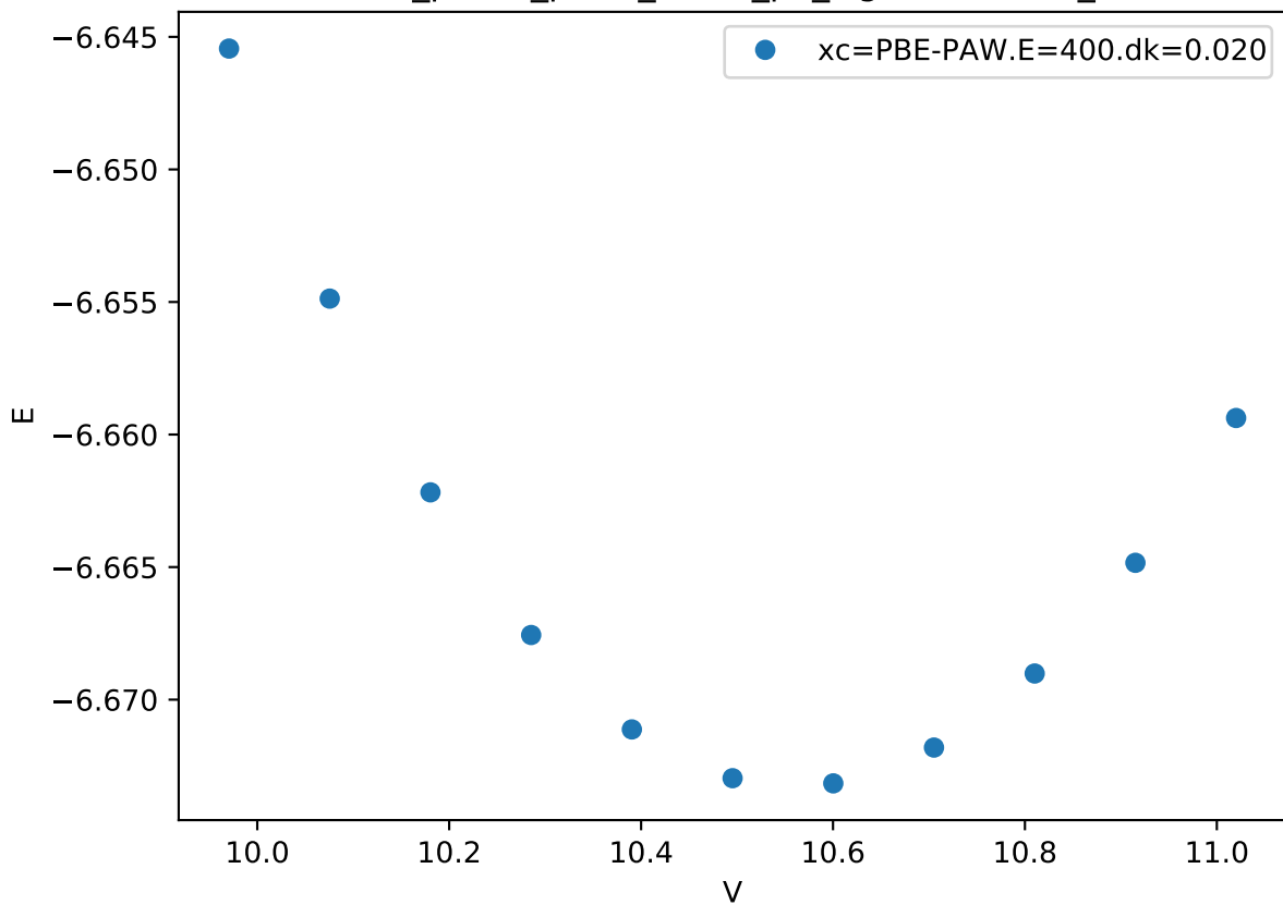
Cr_pv-Co_pv-W_sv/Co_pv_sigma.DDUDU_
