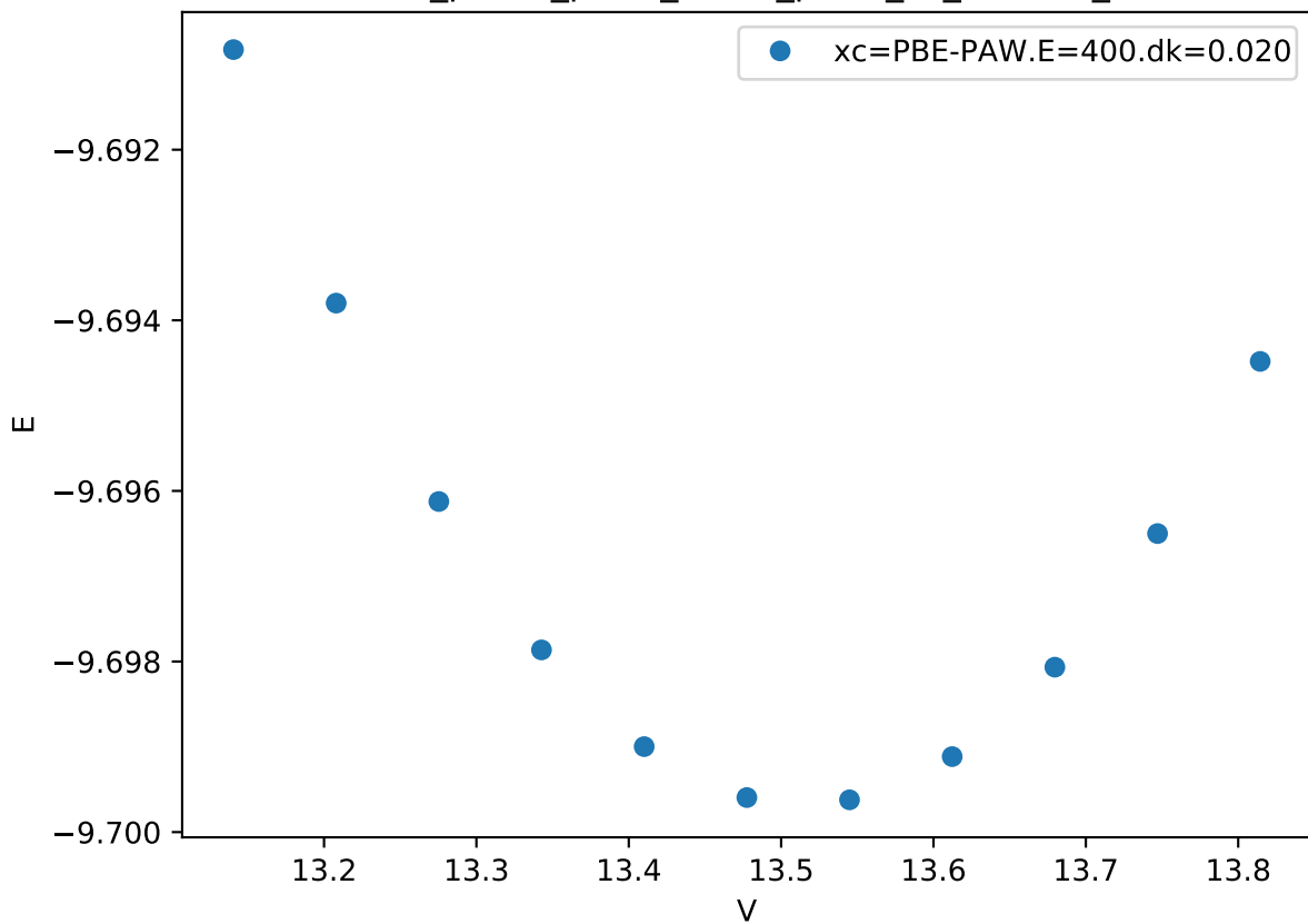
Cr_pv-Co_pv-W_sv/Co_pv-W_sv_B32-AB_
