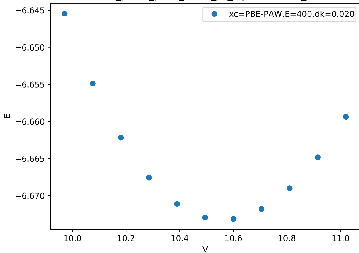
Cr_pv-Co_pv-W_sv/Co_pv_sigma.UDUUD_
