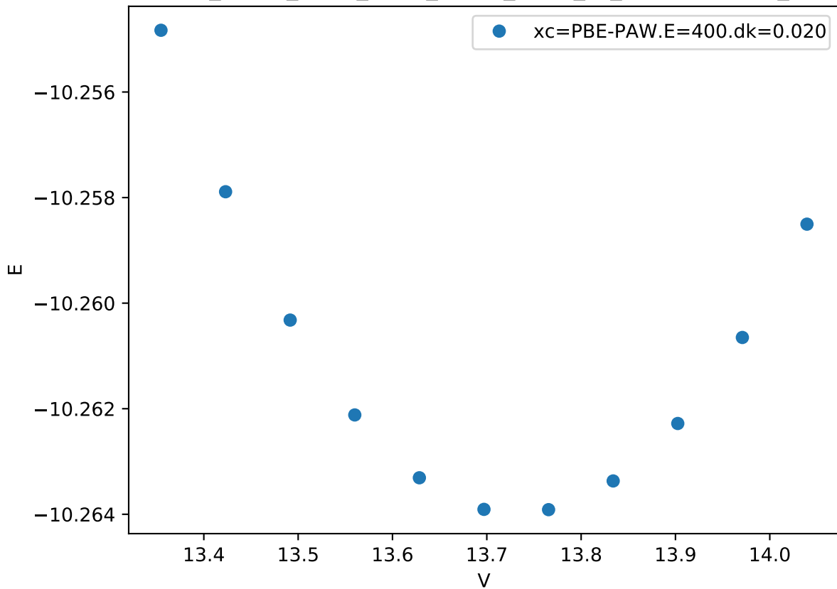
Cr_pv-Co_pv-W_sv/Cr_pv-Co_pv-W_sv_sigma-CCBCA_
