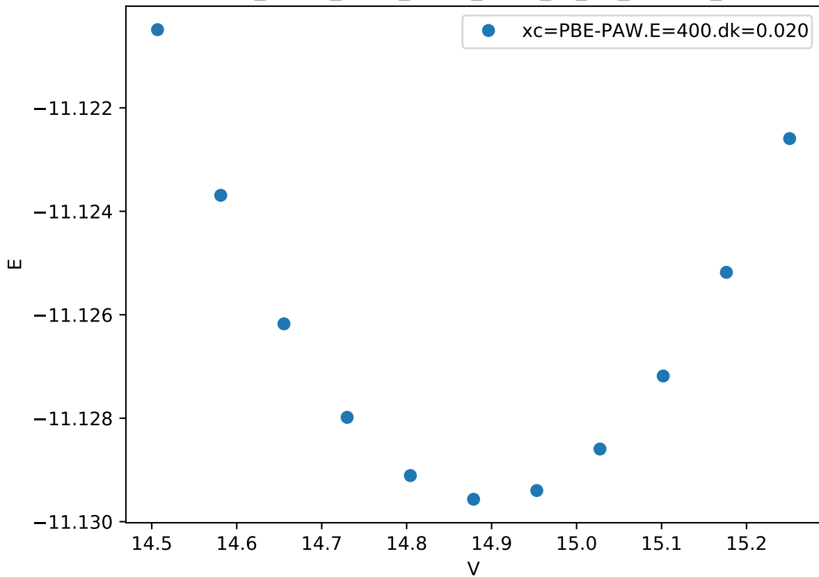
Cr_pv-Co_pv-W_sv/Co_pv-W_sv_D0_19-AB3_
