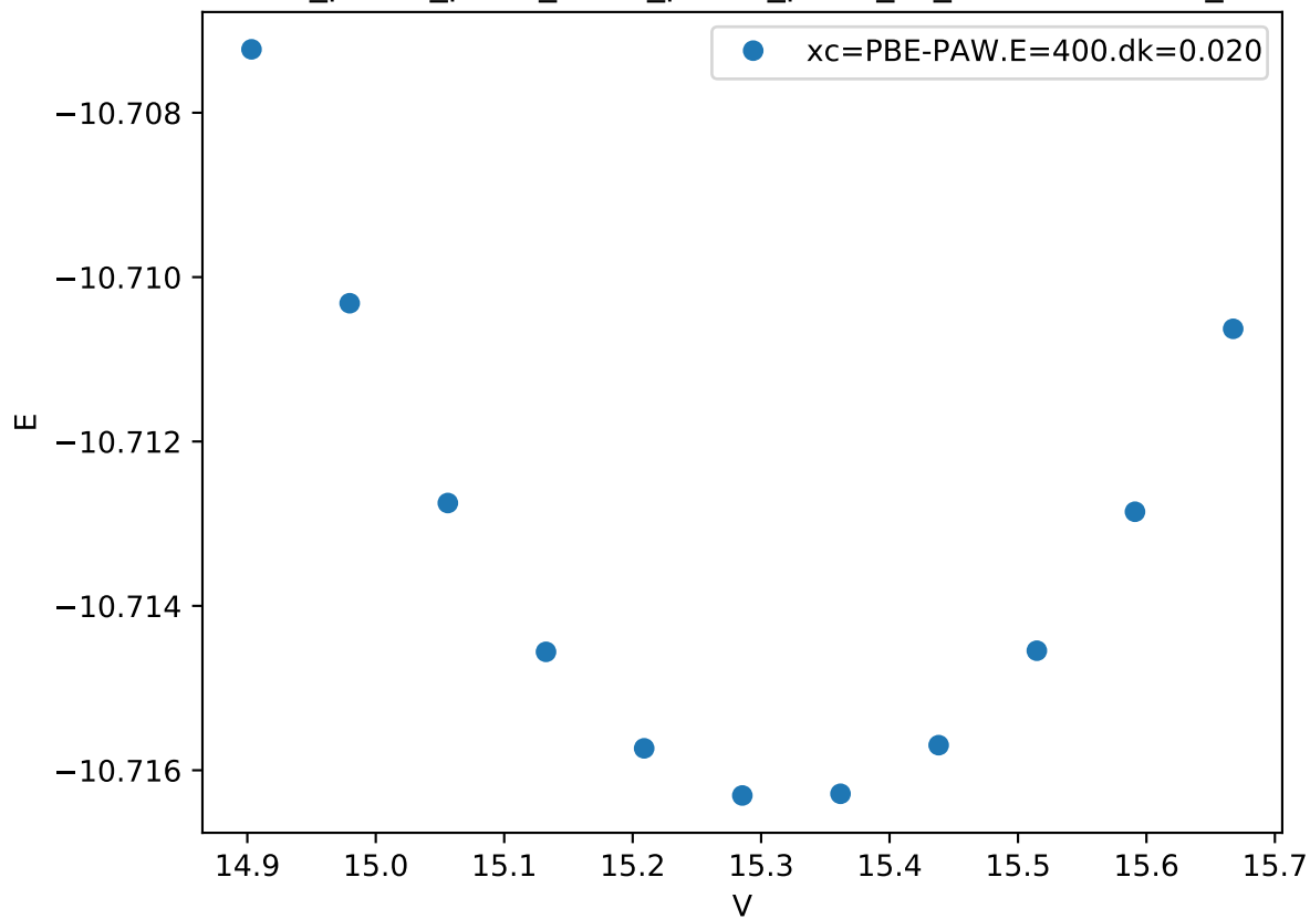
Cr_pv-Co_pv-W_sv/Cr_pv-Co_pv-W_sv_mu-ACCAB.FM_
