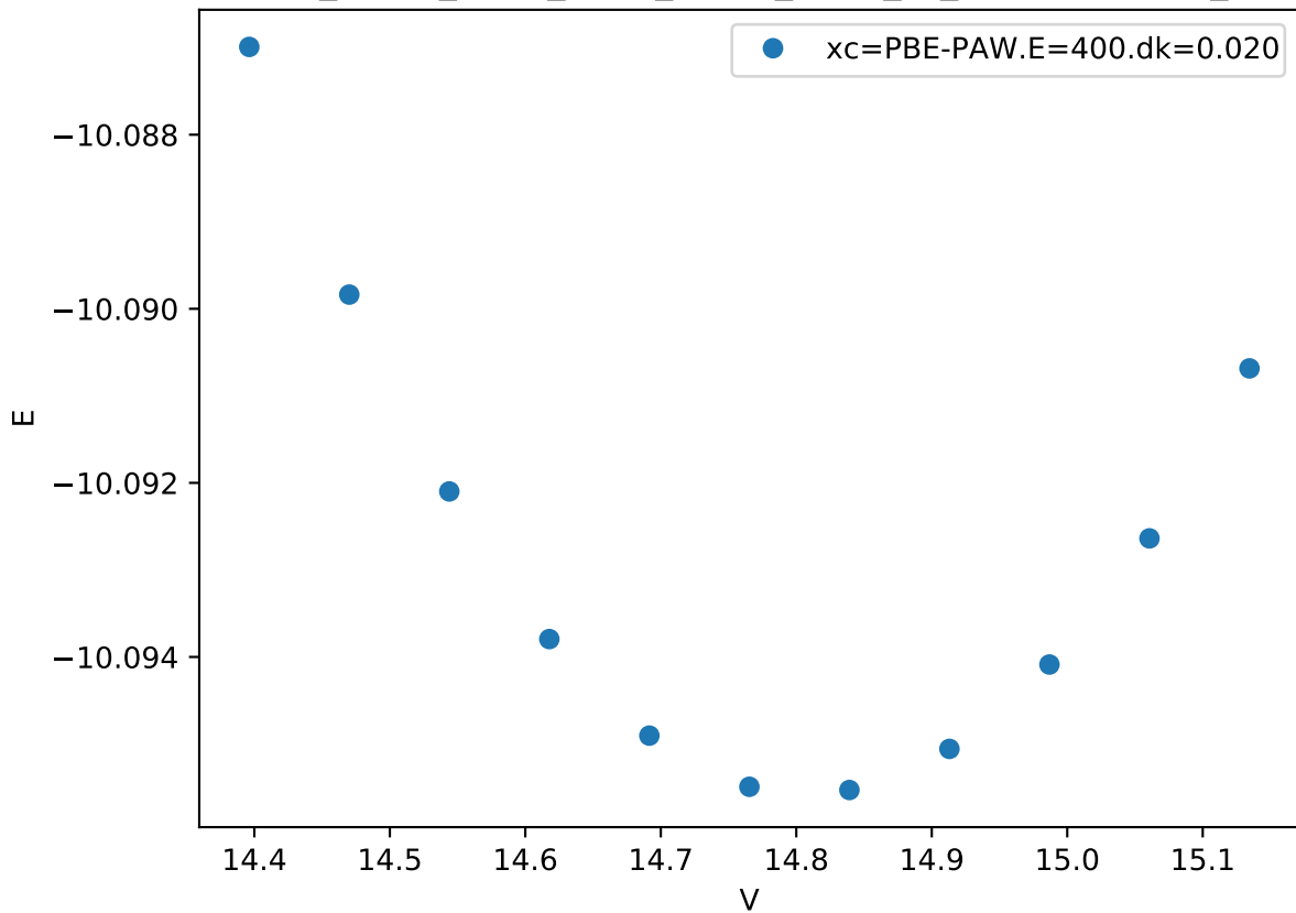
Cr_pv-Co_pv-W_sv/Cr_pv-Co_pv-W_sv_mu-ACABA.FM_
