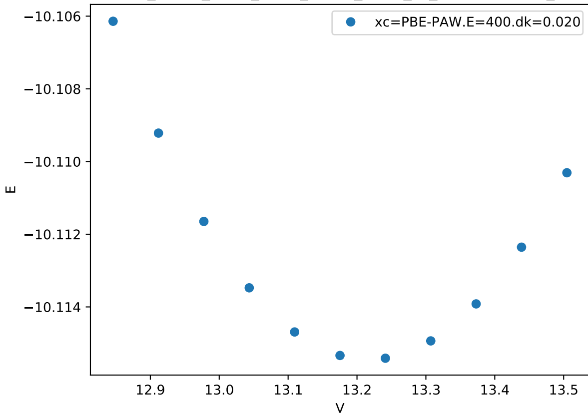
Cr_pv-Co_pv-W_sv/Cr_pv-Co_pv-W_sv_sigma-ACABC_
