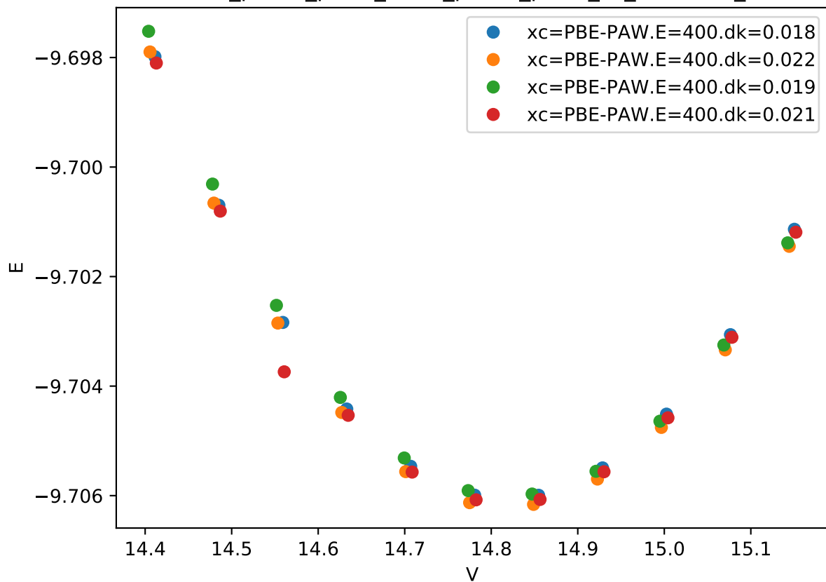
Cr_pv-Co_pv-W_sv/Cr_pv-Co_pv-W_sv_C14-ACB_
