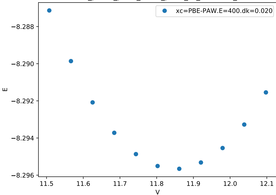
Cr_pv-Co_pv-W_sv/Co_pv-W_sv_D03-A3B_
