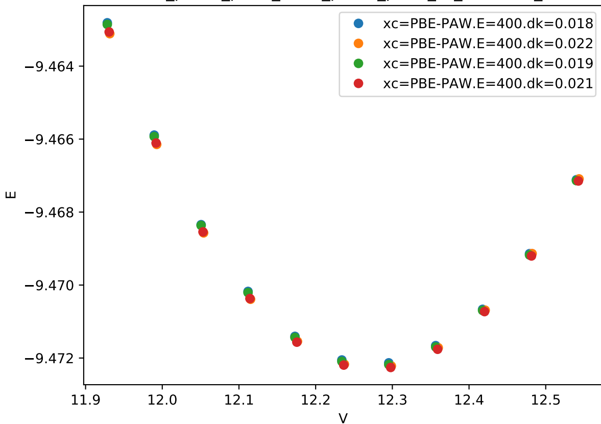
Cr_pv-Co_pv-W_sv/Cr_pv-Co_pv-W_sv_C14-ABC_
