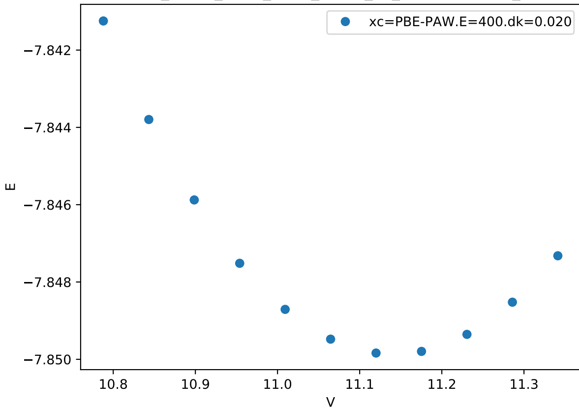
Cr_pv-Co_pv-W_sv/Cr_pv-Co_pv_mu-ABABA.FM_
