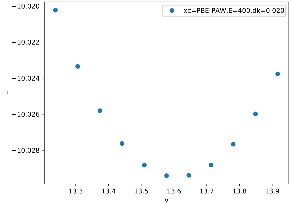
Cr_pv-Co_pv-W_sv/Co_pv-W_sv_sigma-AABAB_
