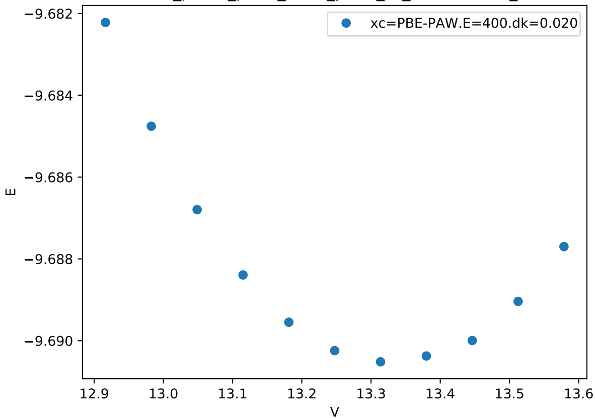
Cr_pv-Co_pv-W_sv/Cr_pv-W_sv_C14-ABA.FM_
