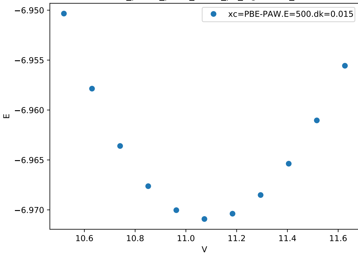
Cr_pv-Co_pv-W_sv/Co_pv_sigma.FM_
