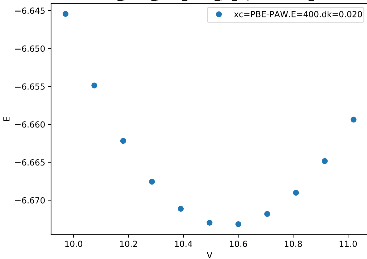
Cr_pv-Co_pv-W_sv/Co_pv_sigma.DDDDD_
