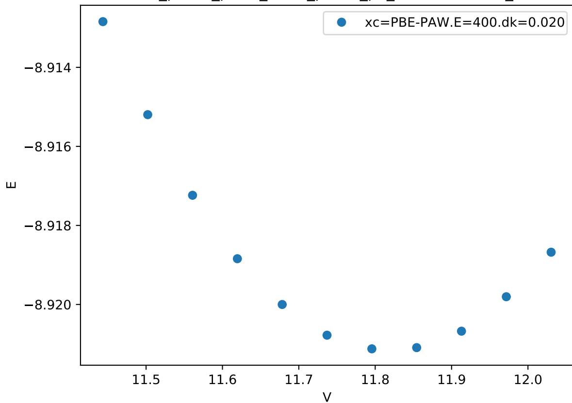
Cr_pv-Co_pv-W_sv/Cr_pv-Co_pv_mu-AAAAB.FM_
