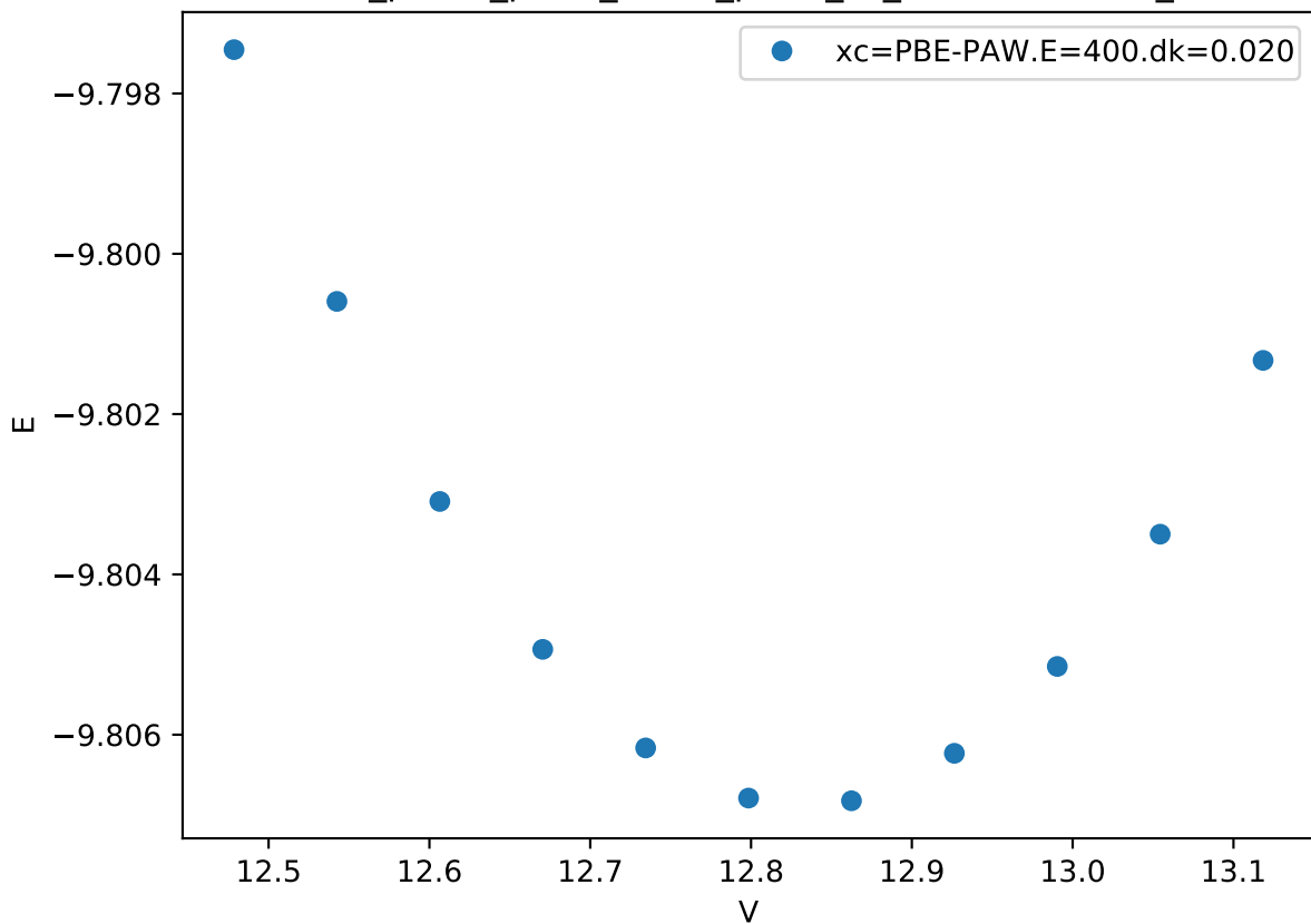
Cr_pv-Co_pv-W_sv/Co_pv-W_sv_mu-AABBB.FM_
