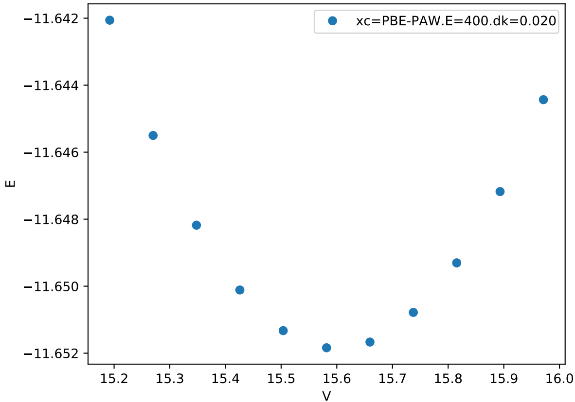
Cr_pv-Co_pv-W_sv/Co_pv-W_sv_C14-BAB_
