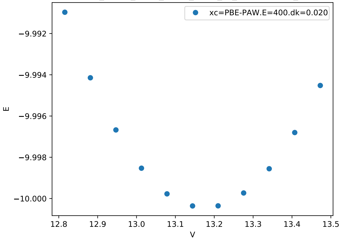
Cr_pv-Co_pv-W_sv/Co_pv-W_sv_C14-BBA.FM_
