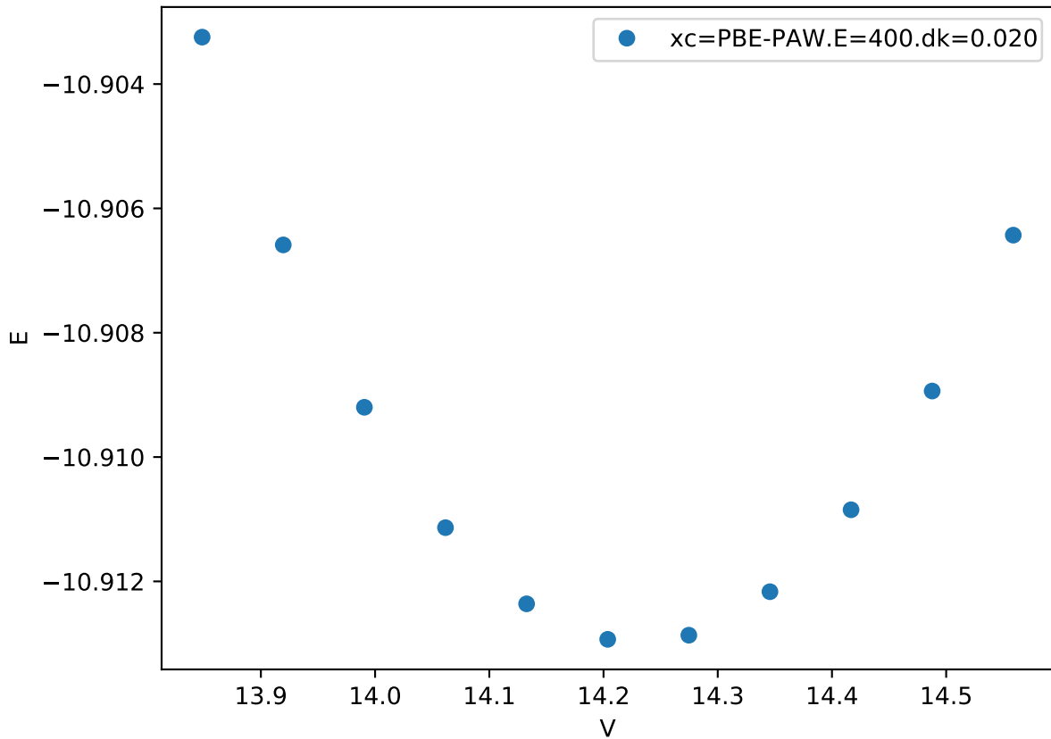
Cr_pv-Co_pv-W_sv/Co_pv-W_sv_sigma-ABBAB_
