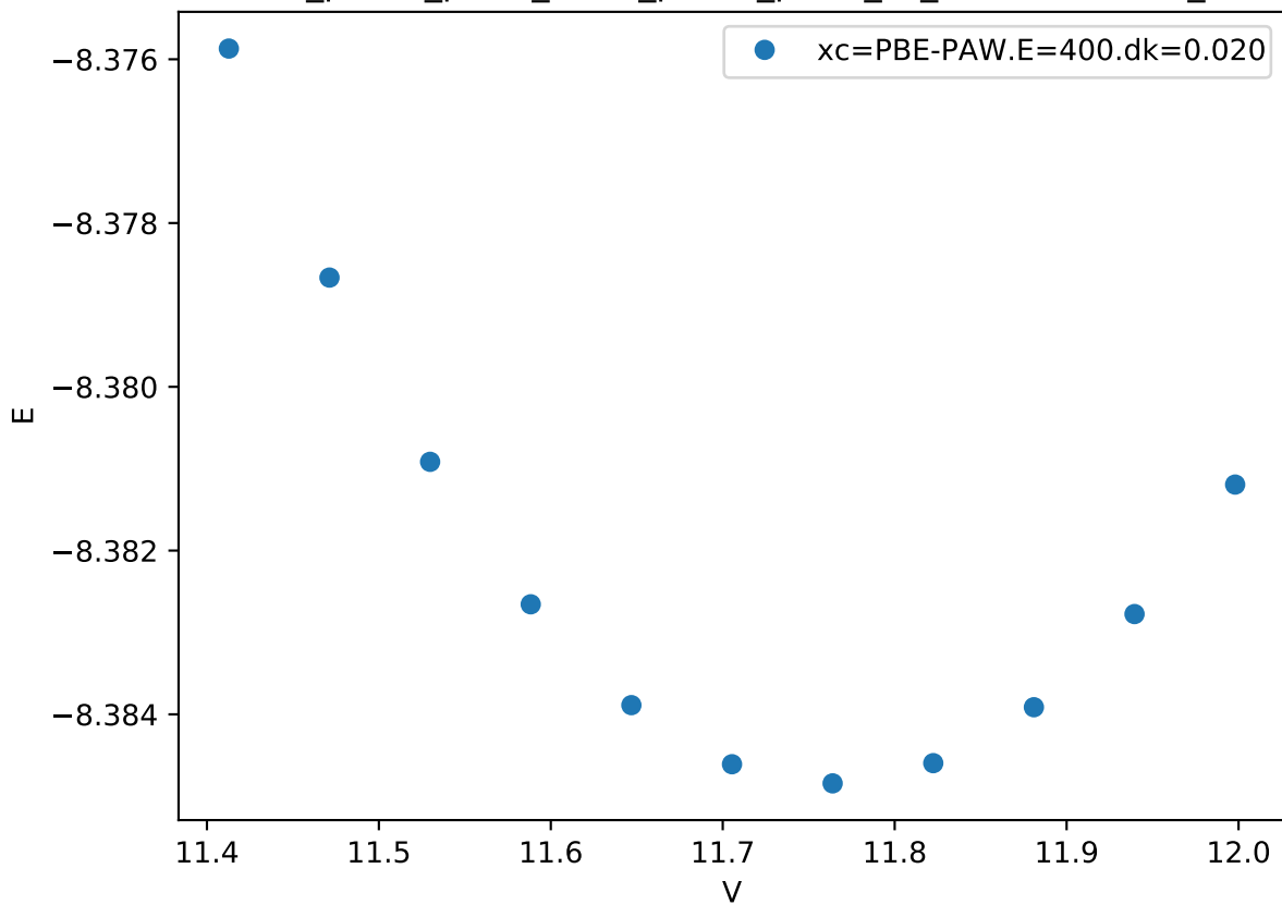
Cr_pv-Co_pv-W_sv/Cr_pv-Co_pv-W_sv_mu-ABABC.FM_
