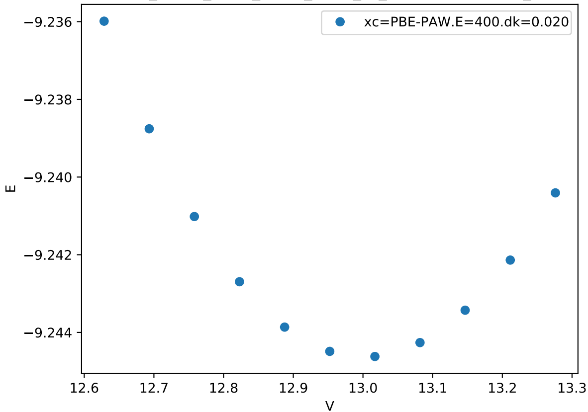
Cr_pv-Co_pv-W_sv/Co_pv-W_sv_sigma-ABBAA.FM_
