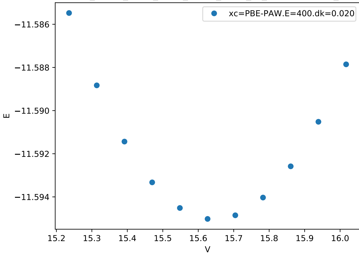
Cr_pv-Co_pv-W_sv/Cr_pv-Co_pv-W_sv_sigma-ABCCC_
