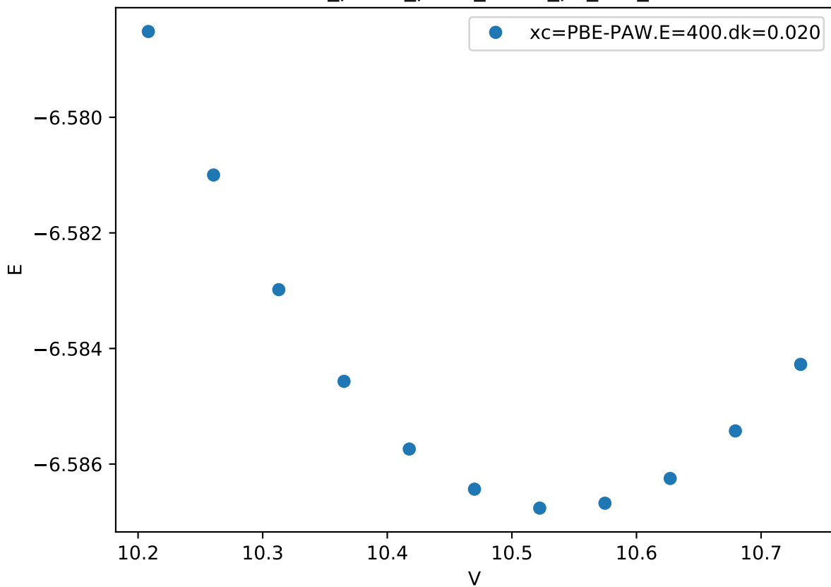
Cr_pv-Co_pv-W_sv/Co_pv_bcc_
