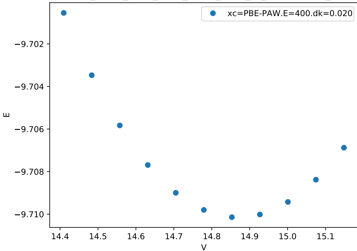
Cr_pv-Co_pv-W_sv/Cr_pv-Co_pv-W_sv_C14-ACB.FM_
