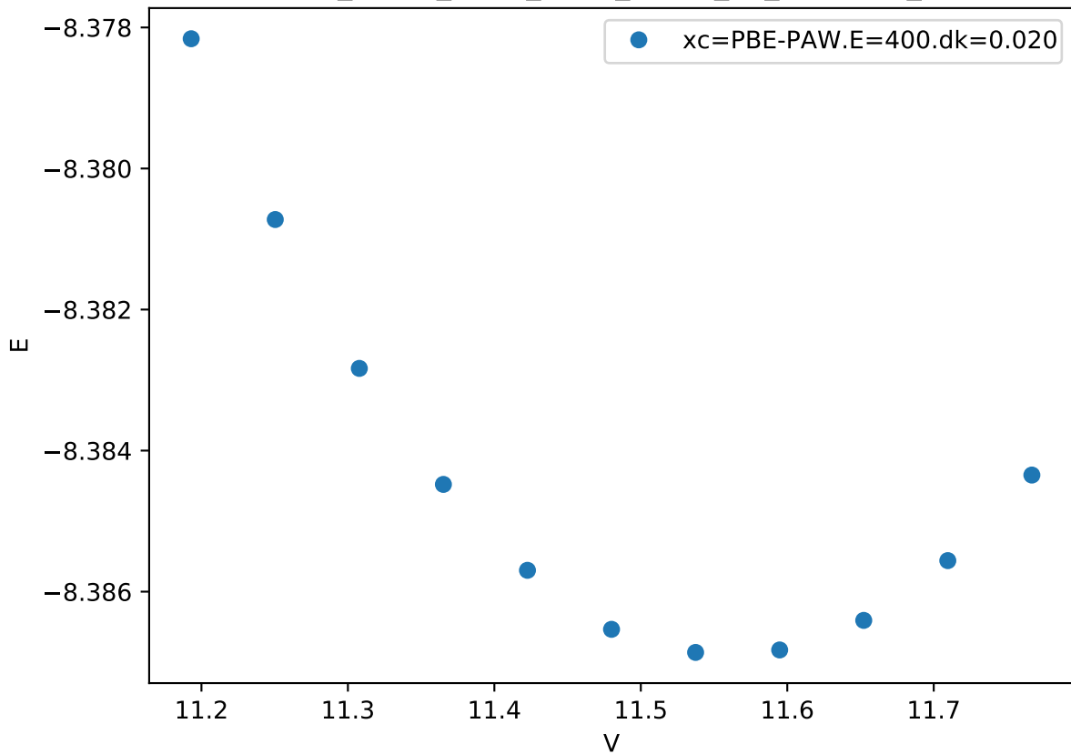
Cr_pv-Co_pv-W_sv/Cr_pv-Co_pv_C14-BAA_
