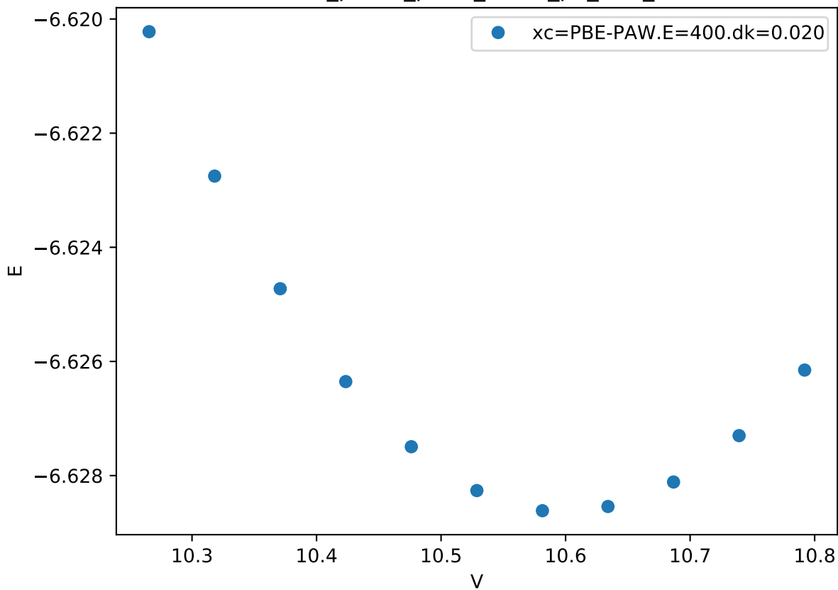
Cr_pv-Co_pv-W_sv/Co_pv_A15_
