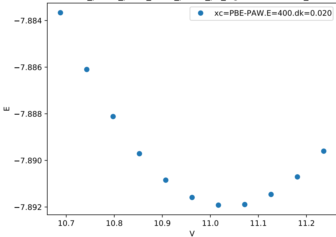
Cr_pv-Co_pv-W_sv/Cr_pv-Co_pv_sigma-BABAB.FM_
