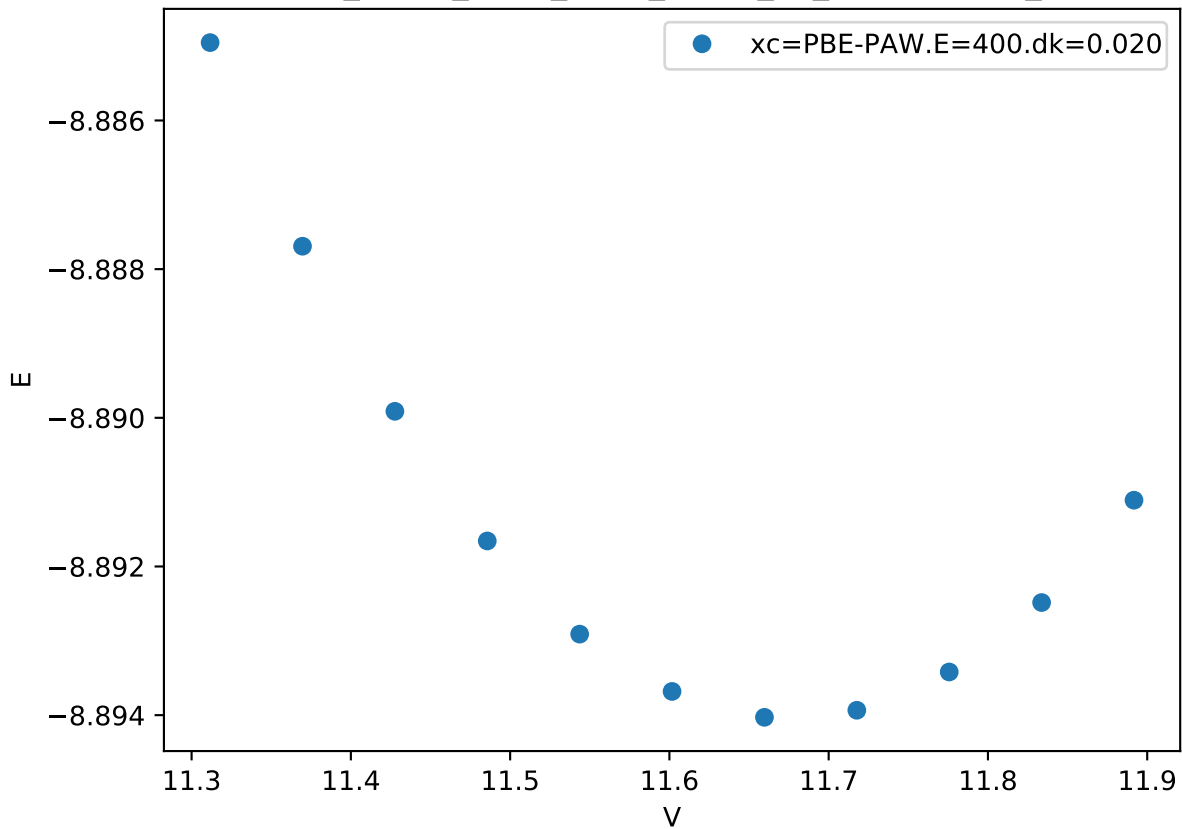
Cr_pv-Co_pv-W_sv/Cr_pv-Co_pv_C14-ABA.FM_
