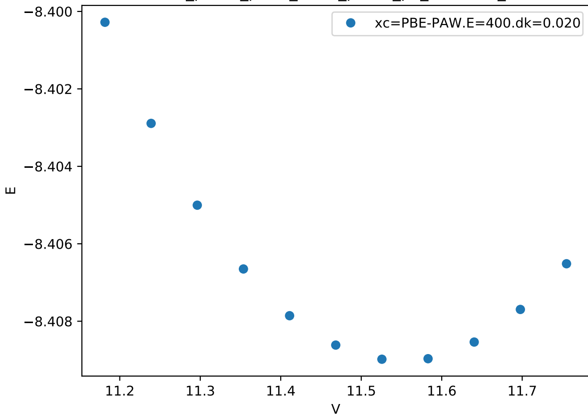
Cr_pv-Co_pv-W_sv/Cr_pv-Co_pv_C15-A2B_
