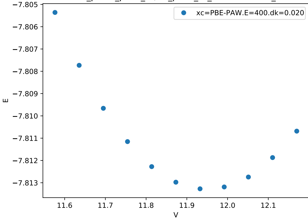
Cr_pv-Co_pv-W_sv/Co_pv-W_sv_mu-AABAA.FM_
