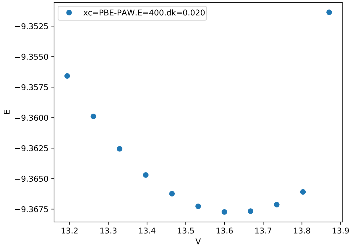
Cr_pv-Co_pv-W_sv/Co_pv-W_sv_chi-BAAB.FM_
