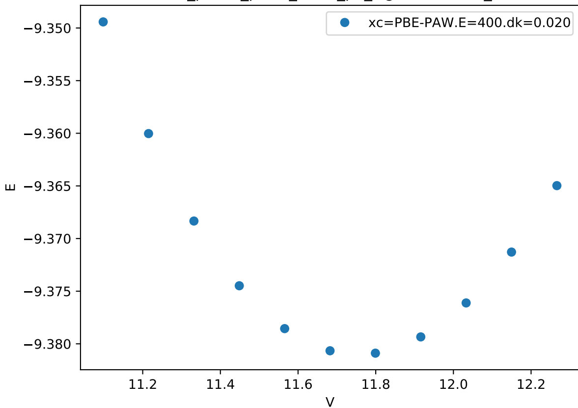
Cr_pv-Co_pv-W_sv/Cr_pv_sigma.DDUUD_
