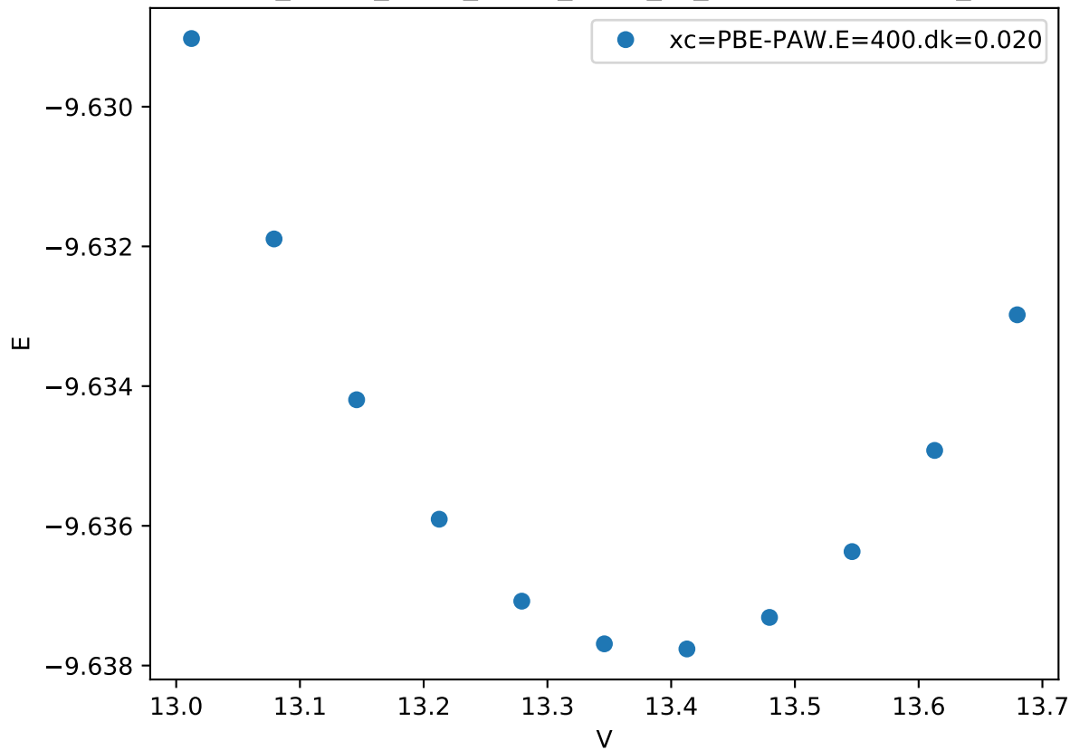
Cr_pv-Co_pv-W_sv/Co_pv-W_sv_sigma-BBAA.FM_
