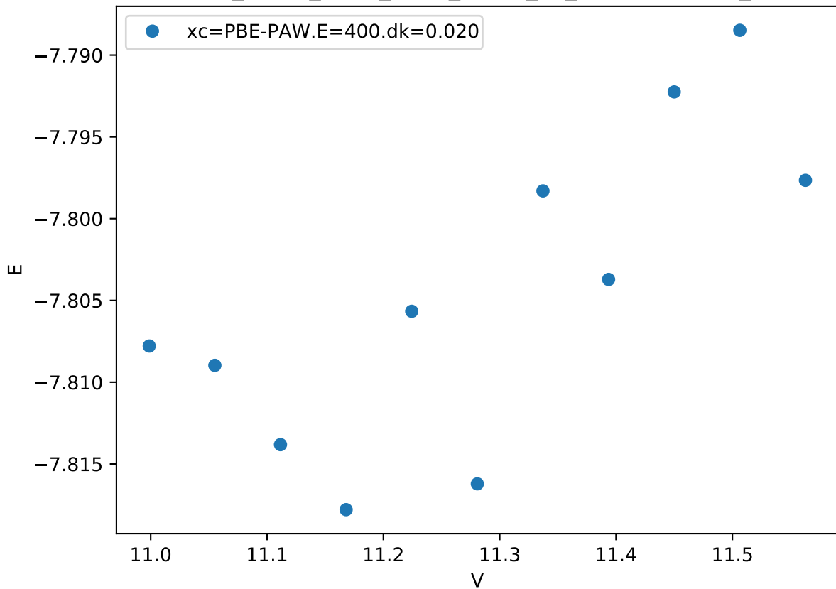
Cr_pv-Co_pv-W_sv/Cr_pv-Co_pv_mu-ABAAB.FM_
