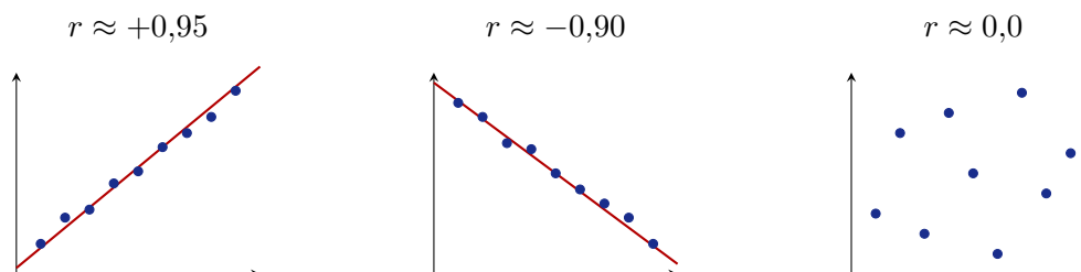
Figura 3: Três padrões típicos de diagrama de dispersão. Esquerda: associação positiva forte. Centro: associação negativa forte. Direita: ausência de associação linear.
