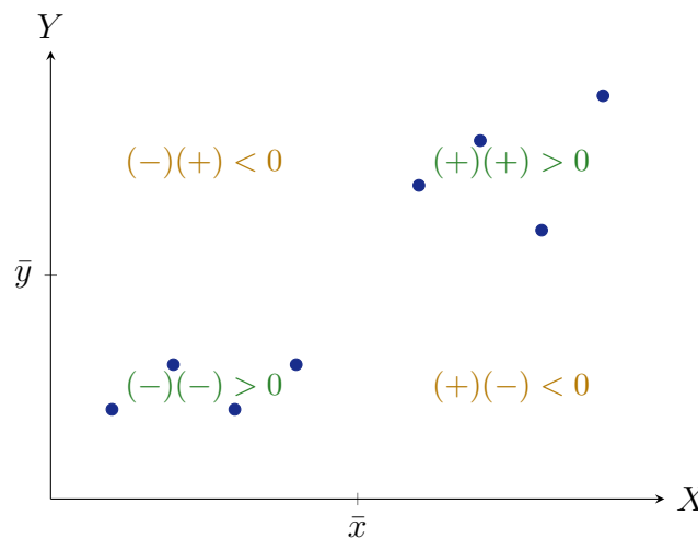
Figura 1: Sinal de (x_i - \bar{x})(y_i - \bar{y}) em cada quadrante formado pelo ponto (\bar{x}, \bar{y}) . Quando os pontos se concentram no 1.º e 3.º quadrantes, a covariância é positiva; quando se concentram no 2.º e 4.º, é negativa.
