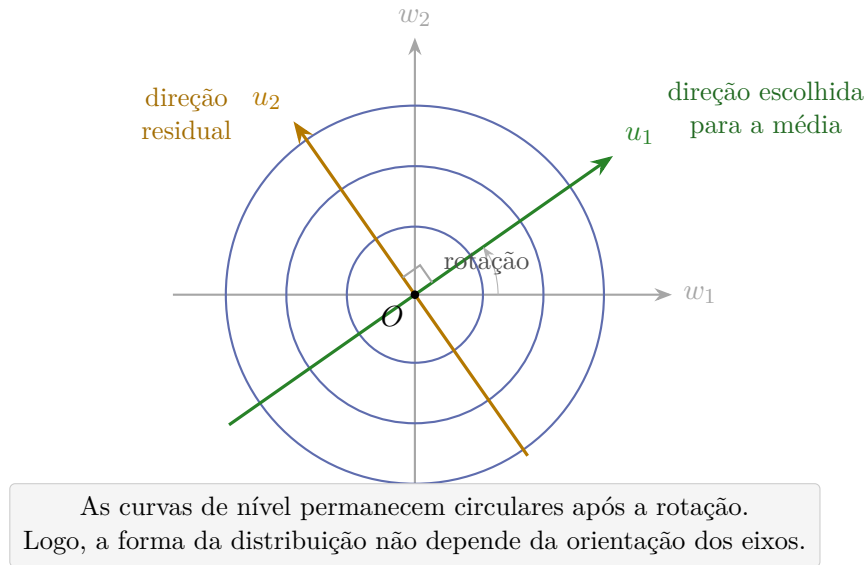
Figura 3: Ilustração bidimensional da simetria esférica da normal multivariada padrão. As curvas de nível são círculos centrados na origem, mostrando que o valor da função densidade depende apenas da distância à origem. Por isso, uma rotação do sistema de coordenadas não altera a forma da distribuição. Essa invariância permite escolher um novo sistema ortonormal de eixos: um eixo u_1 na direção associada à média e um eixo ortogonal u_2 em uma direção residual.
