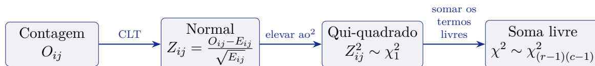
Figura 3: Pipeline conceitual da estatística qui-quadrado. O Teorema Central do Limite justifica, heurísticamente, que cada desvio padronizado Z_{ij} é aproximadamente N(0, 1) ; elevar ao quadrado produz um \chi_1^2 ; a soma dos (r - 1)(c - 1) termos efetivamente livres (após as restrições impostas pelos totais marginais) produz a distribuição \chi_{(r-1)(c-1)}^2 .
