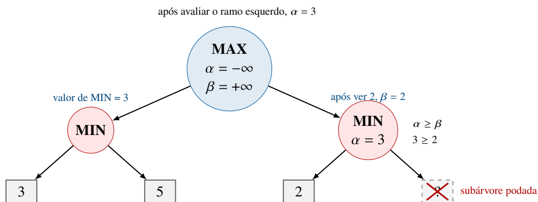
Figura 2: No ramo direito, assim que MIN encontra um filho com valor 2, obtemos \beta = 2 . Como nesse nó vale \alpha \geq \beta (isto é, 3 \geq 2 ), os filhos restantes podem ser podados; mesmo que fossem avaliados, MIN jamais devolveria um valor maior que 2, e portanto MAX nunca preferiria esse ramo ao valor 3 já conhecido.
