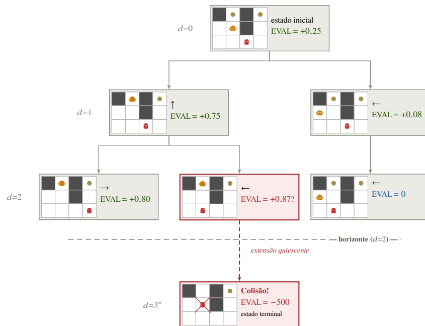
Figura 4: Exemplo de busca quiescente em uma árvore adversarial com alternância de turnos (MAX e MIN). A avaliação heurística considera a proximidade do agente à comida mais próxima e penaliza a proximidade do fantasma a essa mesma comida. No horizonte ( d = 2 ), o nó em vermelho é não quiescente: embora receba uma avaliação aparentemente favorável ( EVAL = +0.87 ), esse valor é enganoso e foi ajustado para fins didáticos, pois ignora uma consequência adversa imediata. A extensão quiescente revela uma colisão no nível seguinte ( EVAL = -500 ), corrigindo a avaliação desse ramo.
