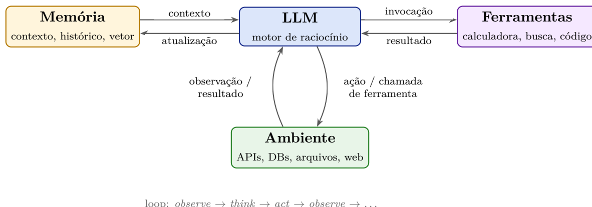
Figura 2: O loop agêntico. O LLM atua como motor de raciocínio central, recebendo contexto da memória, invocando ferramentas para agir sobre o ambiente, e incorporando os resultados de volta ao contexto para o próximo ciclo.
