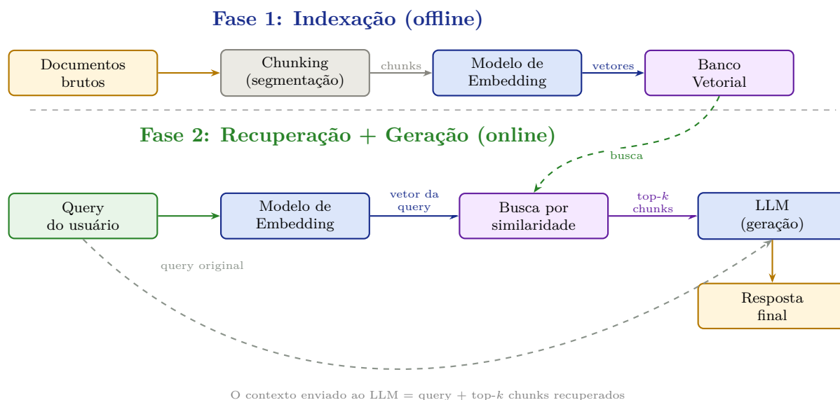
Figura 6: Pipeline RAG em duas fases. Na fase de indexação (offline), documentos são segmentados, transformados em vetores e armazenados. Na fase de recuperação (online), a query do usuário é transformada em vetor, os chunks mais similares são recuperados, e o LLM gera a resposta com base nesses chunks.
