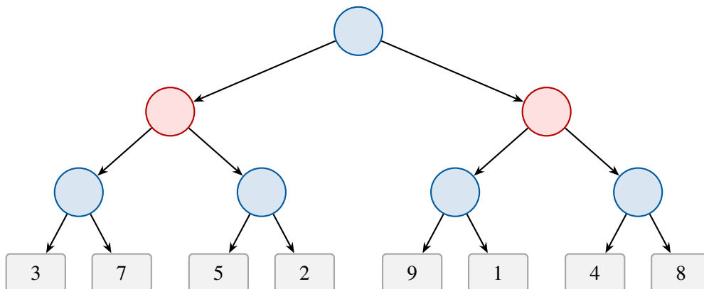
Figura 9: Árvore de jogo da atividade de cálculo Minimax e poda alfa-beta. Círculos azuis são de MAX, círculos vermelhos são de MIN, e retângulos cinza exibem utilidades terminais.
