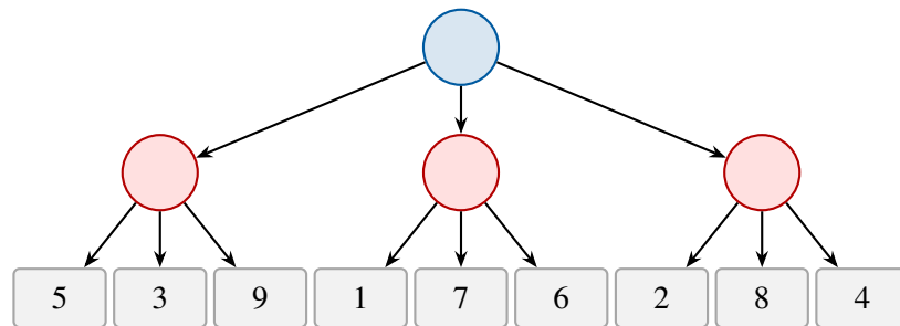
Figura 10: Árvore de jogo para o exercício de poda alfa-beta. A raiz é MAX, os três nós internos no nível seguinte são MIN e as folhas exibem as utilidades usadas na execução da esquerda para a direita.
