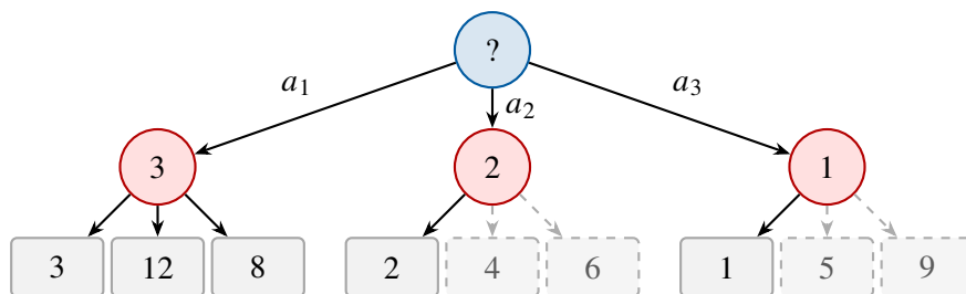
Figura 6: Execução esquemática da poda alfa-beta. Depois de avaliar o primeiro filho dos ramos a_2 e a_3 , os demais filhos desses nós MIN são podados. Setas e caixas tracejadas representam estados que não precisam ser expandidos nem avaliados.
