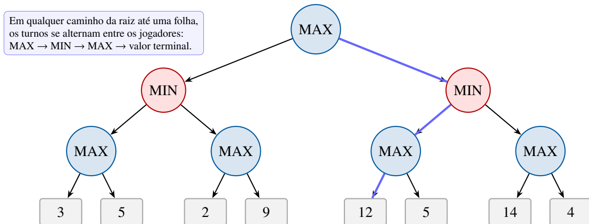
Figura 1: Árvore de jogo esquemática. A alternância entre jogadores ocorre ao longo de cada caminho da raiz até uma folha, refletindo a sucessão de turnos no jogo. O caminho azul é a linha Minimax: no ramo a , MIN pode forçar valor 5; no ramo b , MIN pode forçar 12. MAX escolhe b e, depois da escolha de MIN por b_1 , seleciona a folha de utilidade 12.
