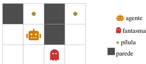
Figura 7: Estado inicial do ambiente usado no exemplo trabalhado da função de avaliação heurística. O agente deve coletar pílulas enquanto evita o fantasma. A função de avaliação combinará o progresso já obtido, a proximidade da pílula mais próxima e a distância até o fantasma.
