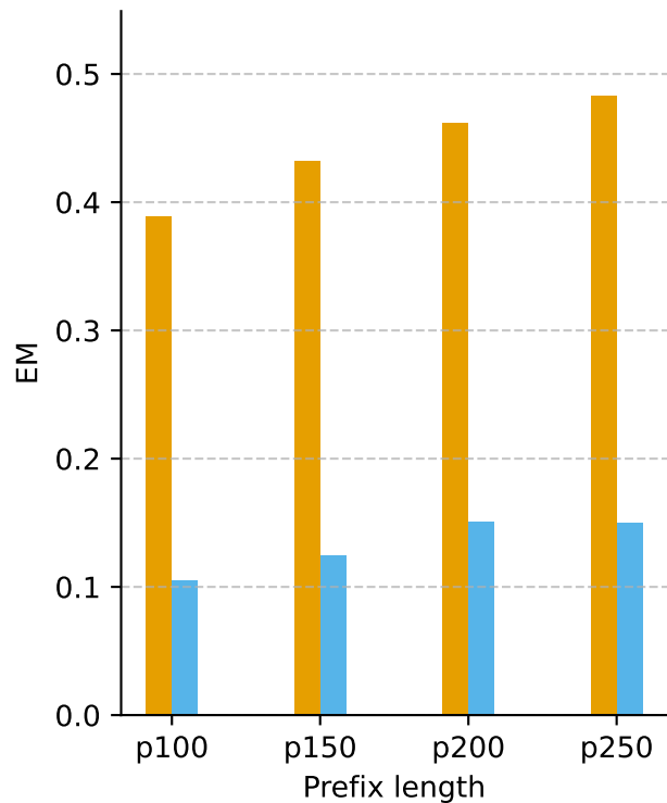
3B
