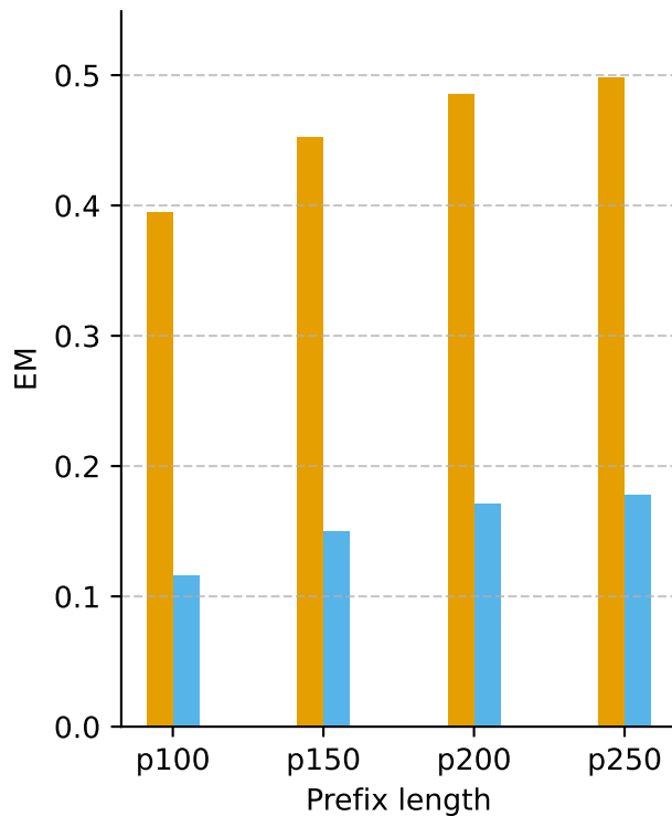
7B
