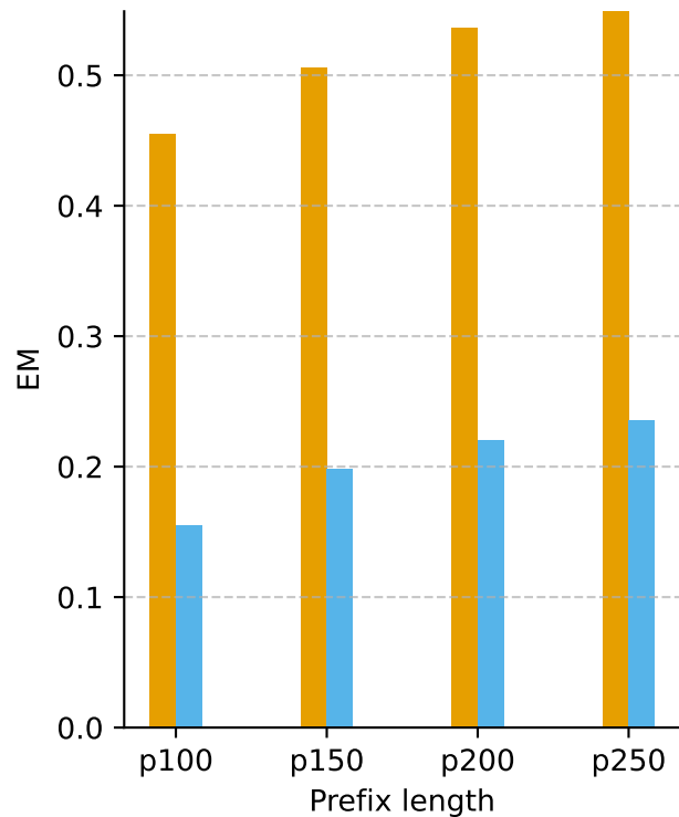
15B
