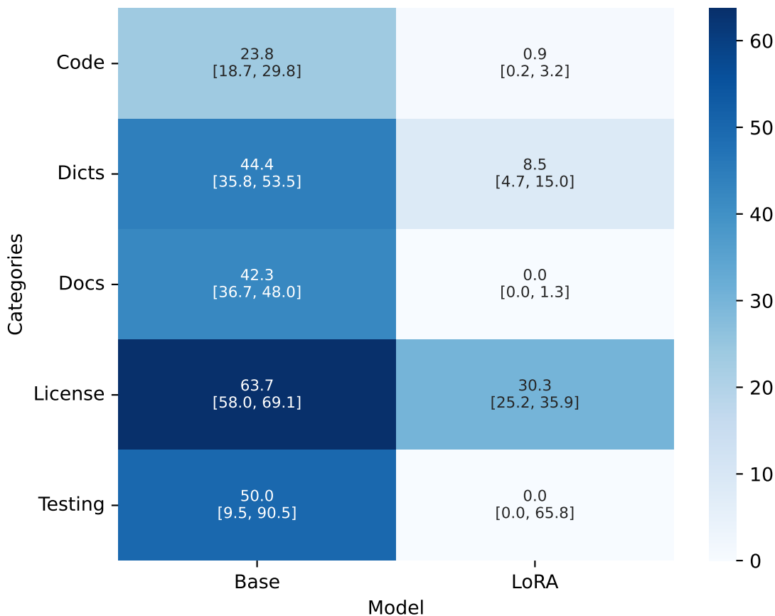
Fine-tune (% , 95% Wilson CI)
