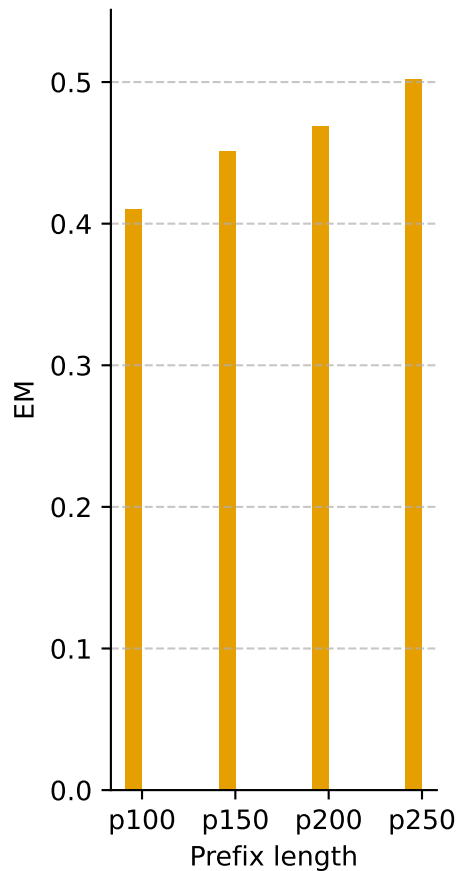
int4
