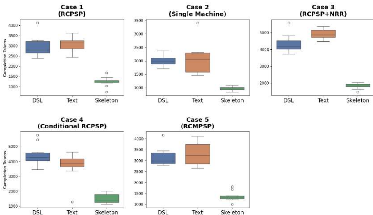
Рис. 9. Диаграммы размаха количества выходных токенов в разрезе подходов и типов задач.
