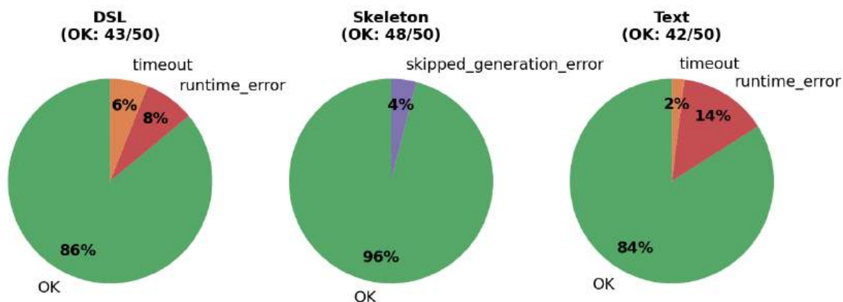
Рис. 10. Распределение статусов компиляции и выполнения сгенерированных решений по подходам.
