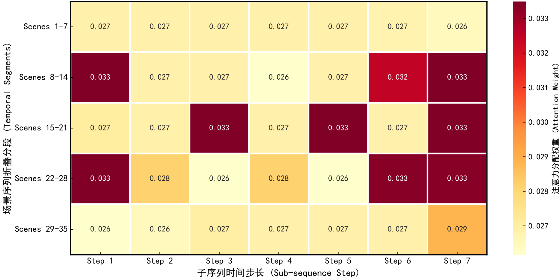
多尺度虚拟场景序列自适应注意力热力矩阵 (Attention Heatmap)
