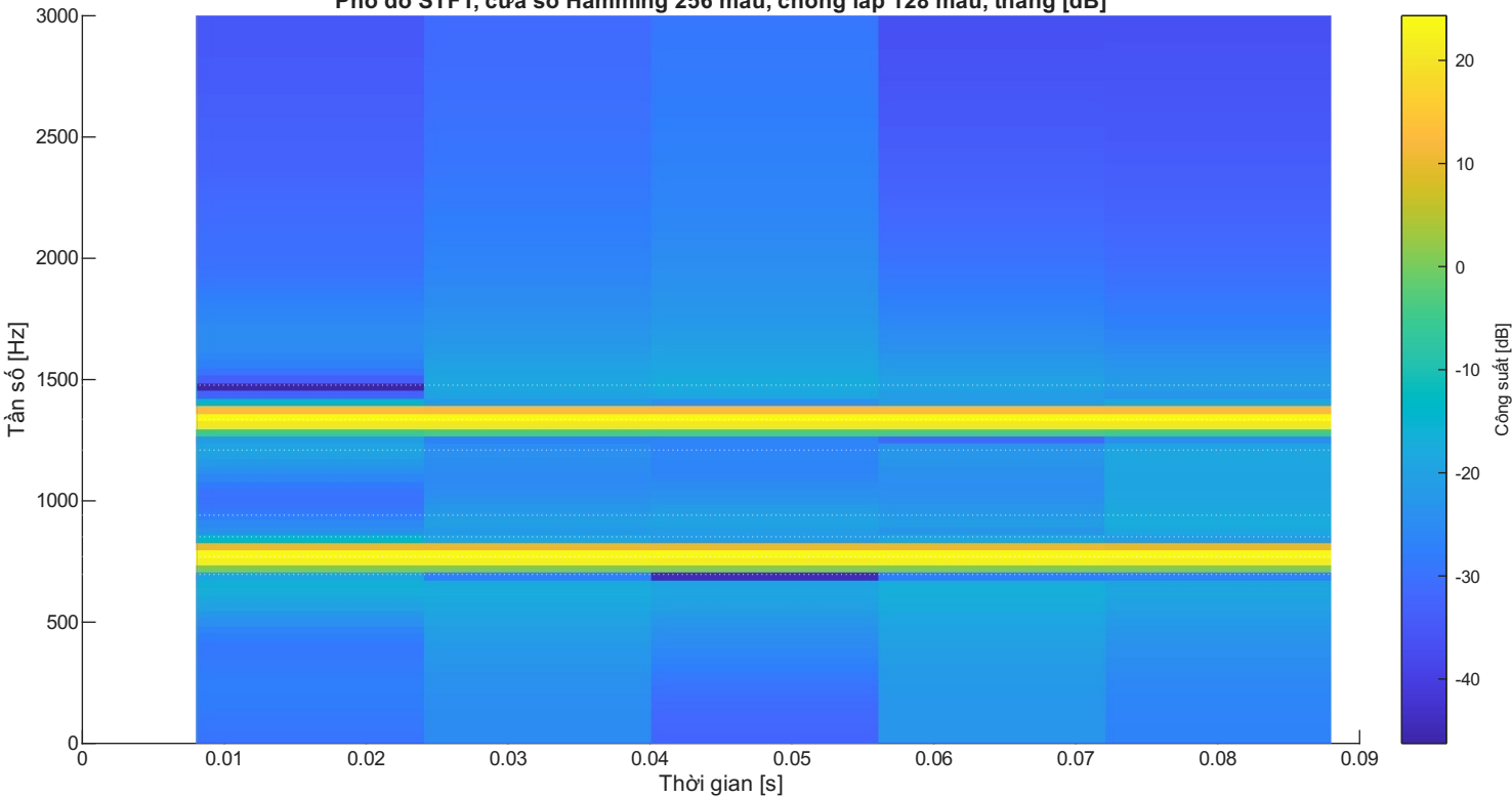
Phổ đồ STFT, cửa sổ Hamming 256 mẫu, chồng lấp 128 mẫu, thang [dB]
