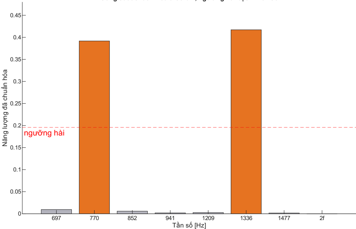
Công suất chuẩn hóa theo bin, ngưỡng hài bậc 2 = 0.196
