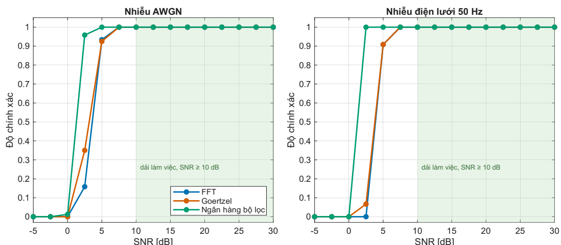
Hình 4.2. Độ chính xác theo SNR với nhiễu AWGN (trái) và nhiễu điện lưới 50 Hz (phải), \rho \geq 0,70 . Vùng tô nền là dải làm việc \text{SNR} \geq 10 \text{ dB} . Với nhiễu AWGN, ngân hàng bộ lọc đạt \text{acc} = 1 từ 5 dB, hai phương pháp còn lại từ 7,5 dB.
