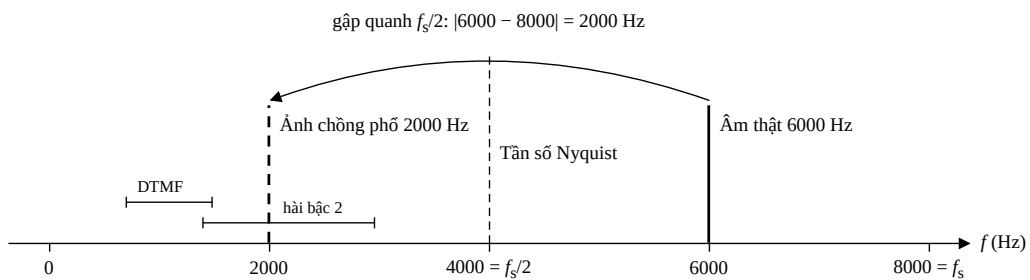
Hình 1.1. Chồng phổ với f_s = 8000\text{ Hz} . Âm 6000\text{ Hz} bị gập về 2000\text{ Hz} , còn dải DTMF nằm dưới f_s/2 nên không bị gập.
