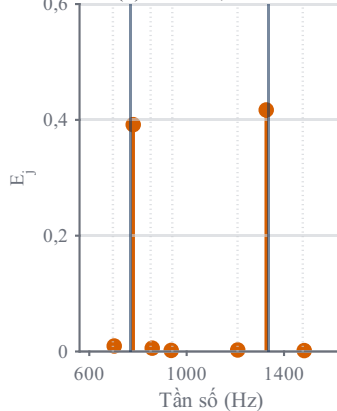
(d) Goertzel, N = 205
