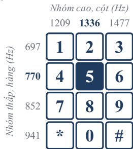
(b) Phím “5” = 770 Hz + 1336 Hz
