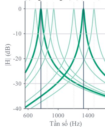
(e) Ngân hàng bộ lọc, r = 0,99
