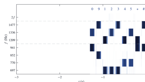
Hình 3: Năng lượng 8 bin theo khung, thang màu 0 – 0,5
