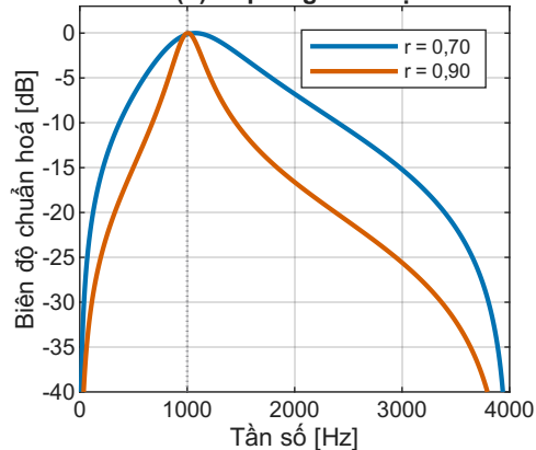
(b) Đáp ứng biên độ
