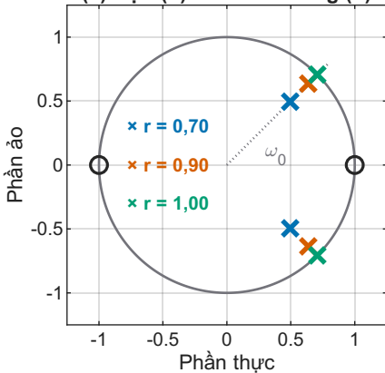
(a) Cực (x) và điểm không (o)
