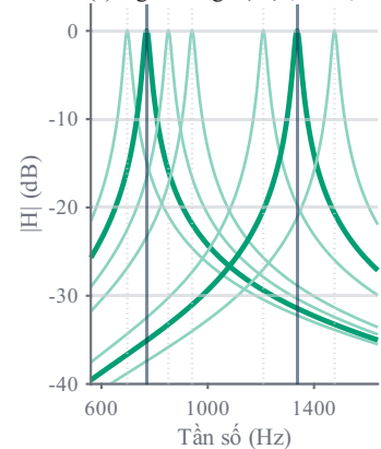
(e) Ngân hàng bộ lọc, r = 0,99
