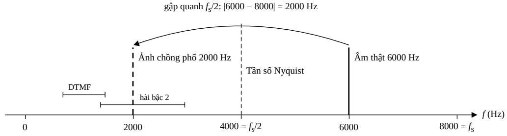
Hình 1.1. Minh hoạ chồng phổ với f_s = 8000 Hz: âm 6000 Hz nằm trên tần số Nyquist bị gập quanh f_s/2 và xuất hiện tại 2000 Hz. Hai đoạn ngang đánh dấu dải DTMF (697-1477 Hz) và dải hài bậc hai (1394-2954 Hz), đều nằm dưới f_s/2 .
