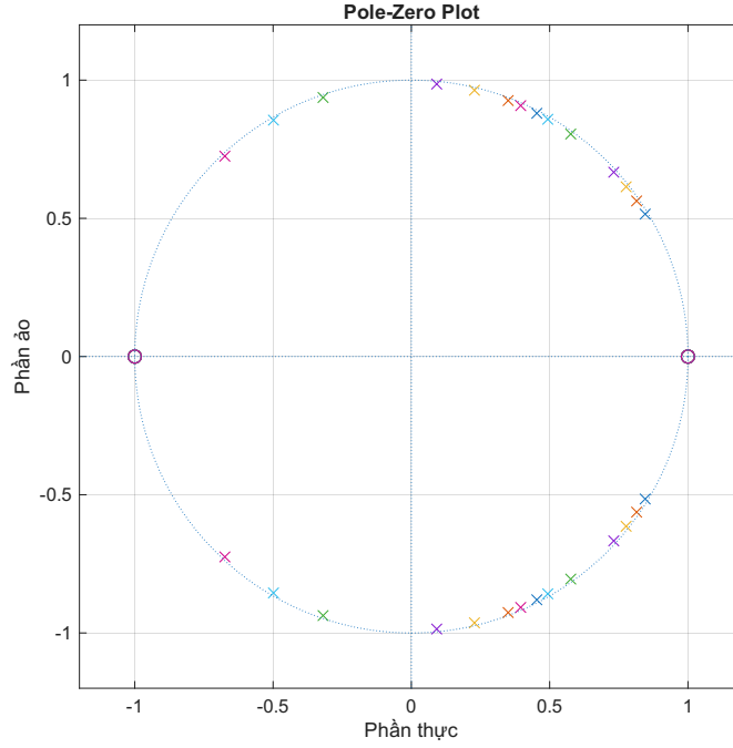
Hình 2.8. Vị trí cực (×) và điểm không (○) của 14 bộ cộng hưởng với r = 0,99 . Các cực nằm sát bên trong đường tròn đơn vị; cả 14 bộ dùng chung hai điểm không tại z = \pm 1 .
