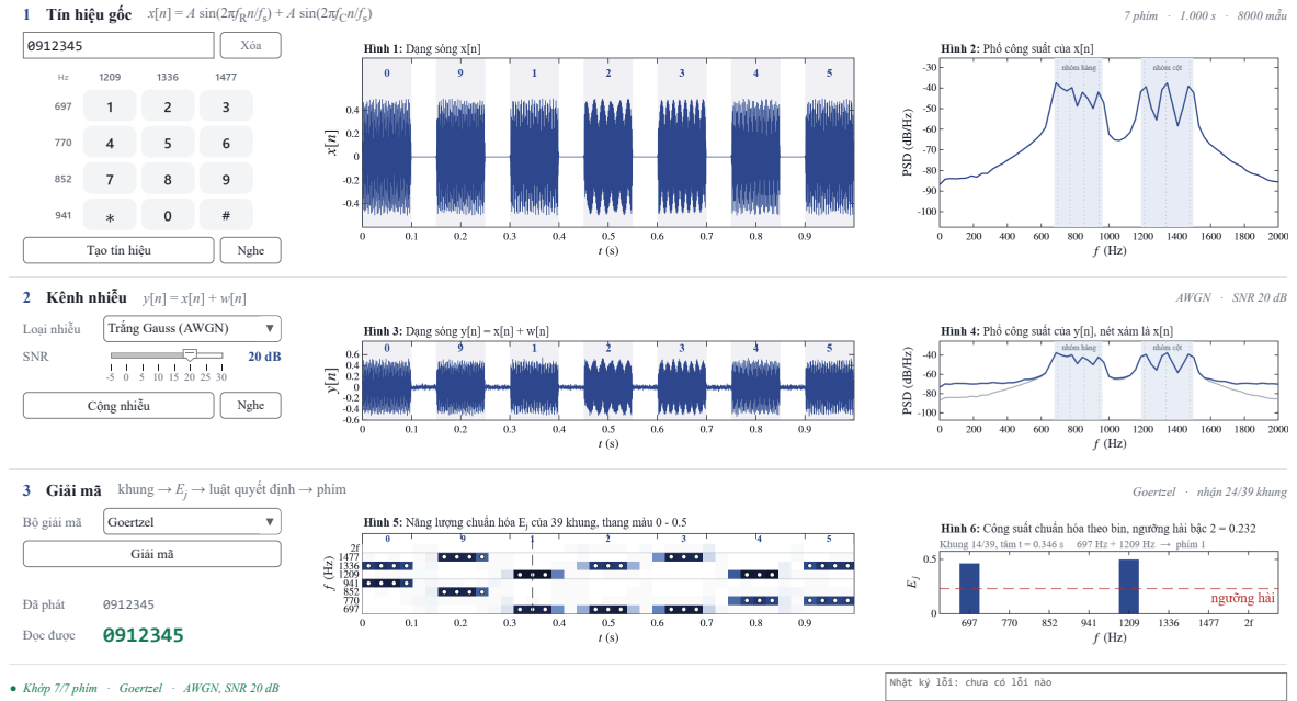
Hình 3.5. Giao diện DTMFApp với chuỗi “0912345”, nhiễu AWGN ở SNR 20dB và bộ giải mã Goertzel. Ba hàng từ trên xuống là tín hiệu gốc, tín hiệu có nhiễu và kết quả giải mã; chuỗi đọc được khớp 7/7 phím.
