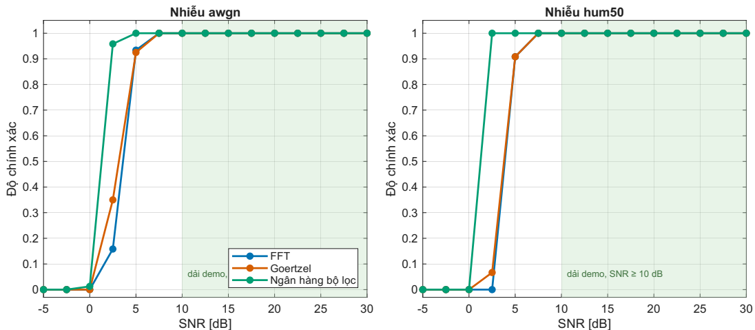
Hình 4.2. Độ chính xác theo SNR với nhiễu AWGN (trái) và nhiễu ù 50 Hz (phải), \rho \geq 0,70 . Vùng tô nền là dải làm việc SNR \geq 10 dB.
