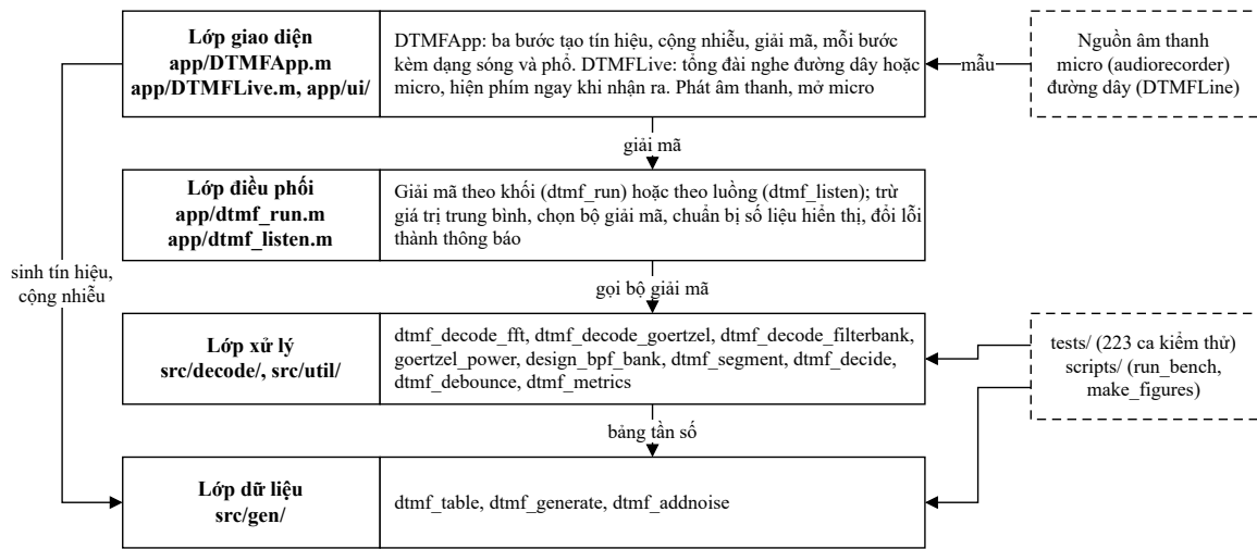
Hình 3.2. Kiến trúc phần mềm bốn lớp. Mũi tên chỉ chiều gọi hàm; khối nét đứt là nguồn âm thanh bên ngoài và mã kiểm thử.
