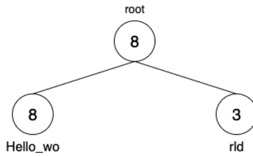
Hình 3: Minh họa sau khi thêm chuỗi "Hello_World" vào Rope rỗng
