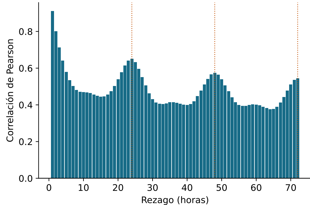
Autocorrelación hasta 72 horas
