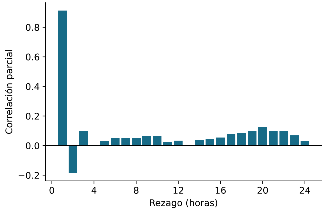
Correlación parcial, primeros 24 rezagos
