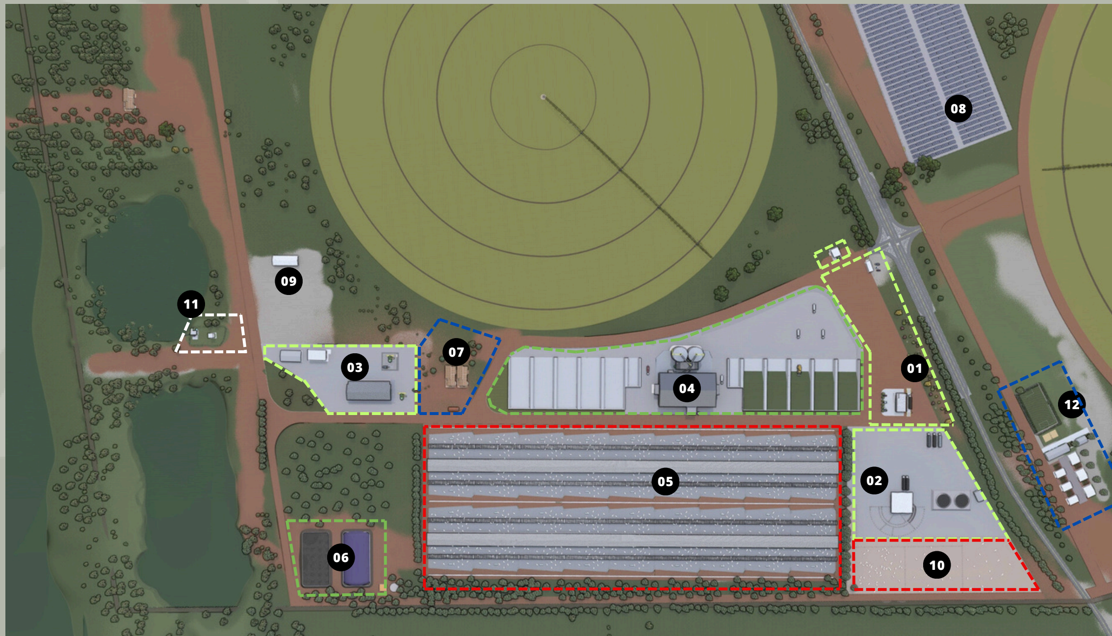
Masterplan Sede - Zoneamento
