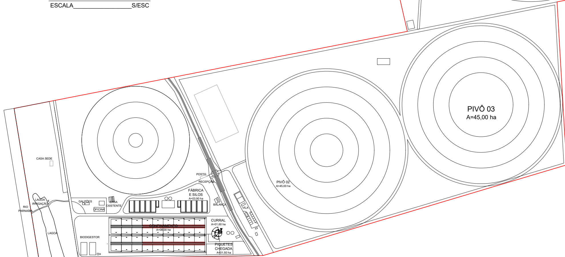
MASTERPLAN - PLANTA GERAL ESCALA _____ S/ESC
