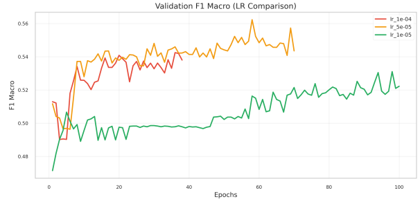
(b) Bi-RNN macro F1.
