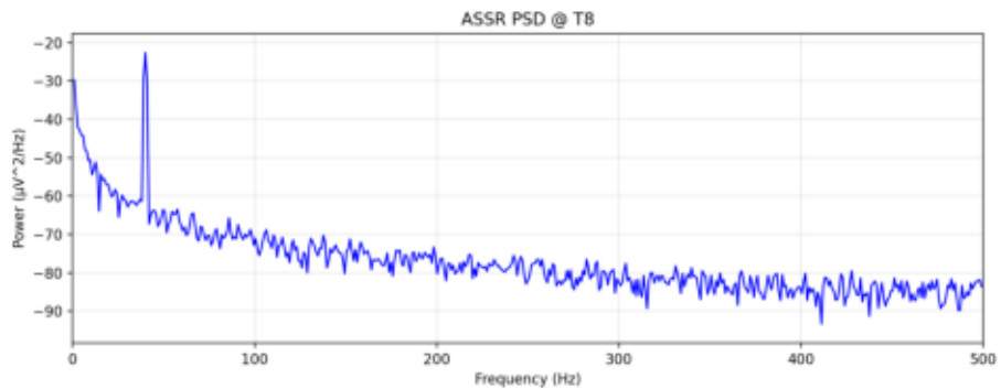
CortiPy ASSR psd
