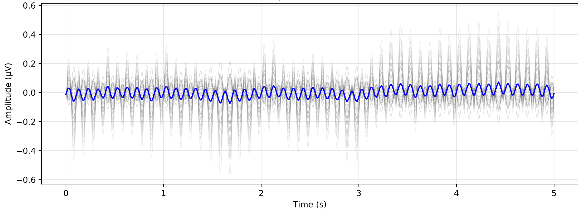
CortiPy SSVEP trace (Oz)
