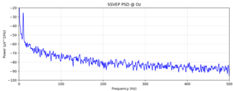
CortiPy SSVEP psd
