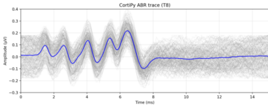
CortiPy ABR trace
