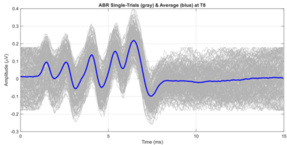
EEGLAB ABR trace
