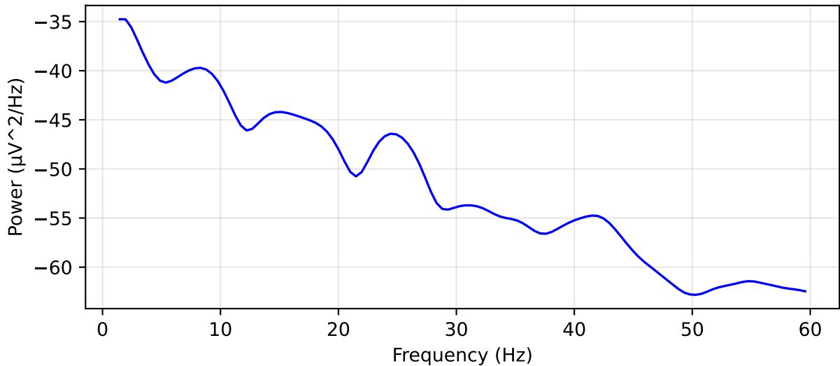
Oddball PSD (mean of EEG)
