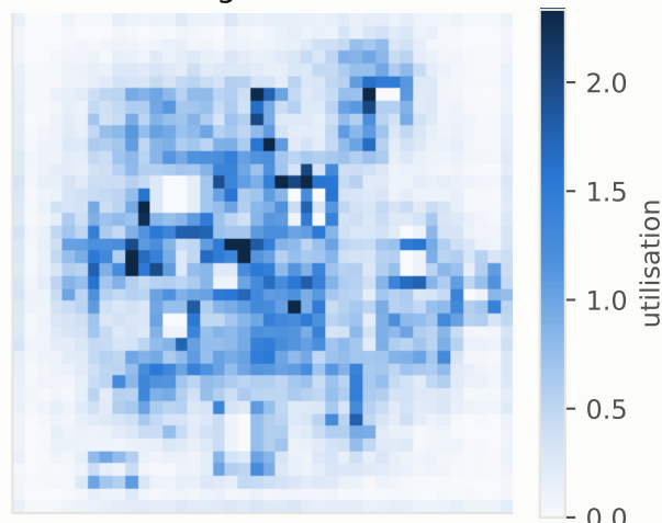
routing utilisation
