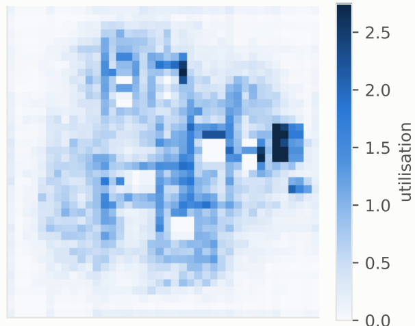
routing utilisation
