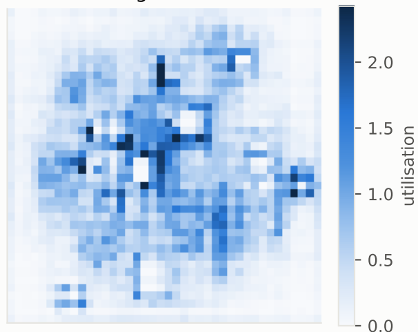
routing utilisation
