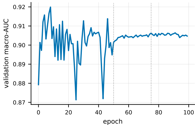
validation AUC
