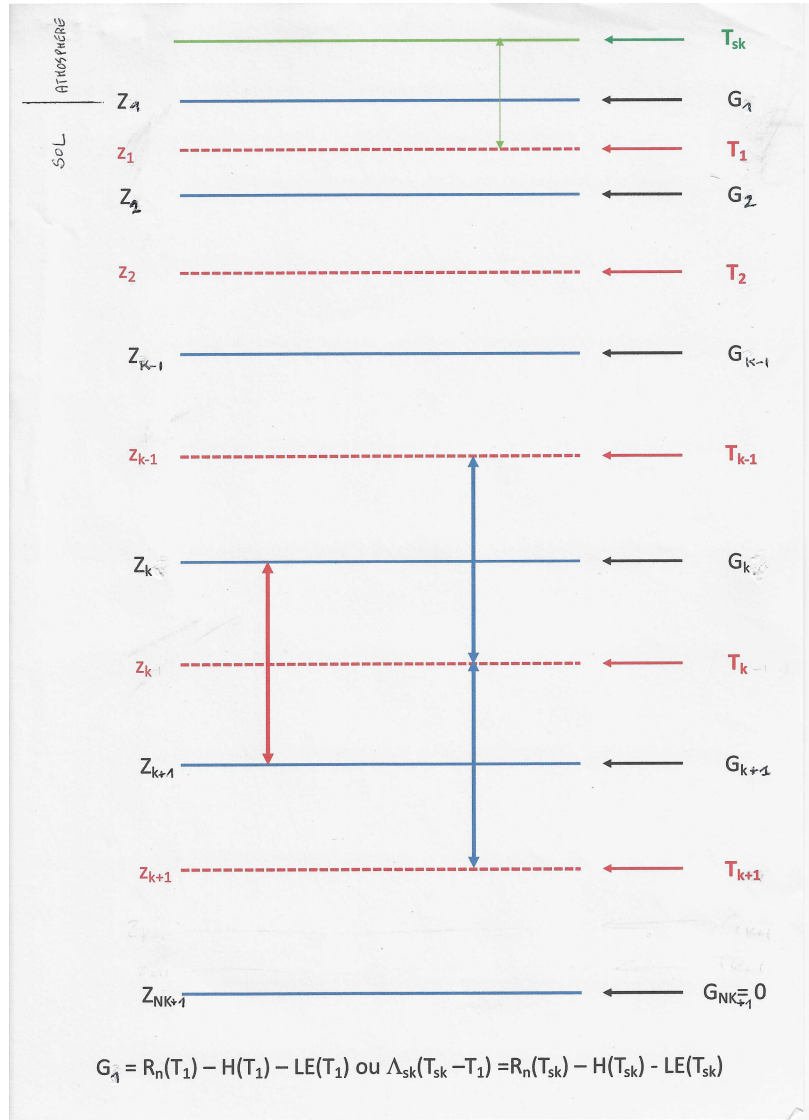
Figure 2: Discrétisation verticale dans le sol pour résoudre l'équation de diffusion de la température. Les niveaux entiers z_k où est définie la température T_k correspondent aux lignes en tiretés rouge. Les demi-niveaux Z_k où sont calculés les flux G_k correspondent aux lignes bleues en traits pleins. Un niveau supplémentaire pour le flux est créé au niveau NK + 1 (extrapolation) pour imposer une condition de flux nul à la limite inférieure du sol (définie par z_{NK} ). La ligne verte fléchée est associée au calcul de la température de peau T_{sk} avec un couplage sol-atmosphère par le flux G_1 = \Lambda_s(T_{sk} - T_1) . Les lignes fléchées bleues correspondent au calcul des flux de chaleur par conduction et la ligne fléchée rouge au calcul de la divergence de ces flux.
