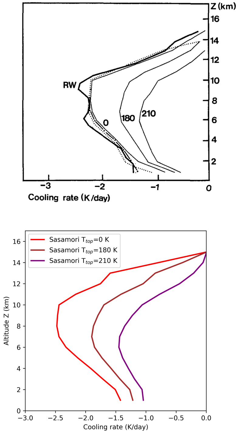
Figure 3: Taux de refroidissement infrarouge simulé à partir d'un profil atmosphérique de London 1952 proposé dans Savijärvi (1990) (Tableau 1). La figure du haut présente les résultats obtenus par Savijärvi (1990) avec l'approximation de Sasamori (1972) pour trois températures au sommet du modèle de transfert radiatif (en traits continus fins). La courbe en trait plein épais représente la simulation avec un modèle plus complet (plusieurs bandes spectrales) de Rodgers and Walshaw (1966) considéré ici comme la référence. La courbe en trait mixte a été obtenue avec l'approximation "cooling to space" et la courbe en pointillés avec le modèle à une bande complet (calcul des flux montant et descendant à chaque niveau). La figure du bas représente les simulations que j'ai effectuées avec la méthode de Sasamori (1972) pour les trois même températures (0, 180 et 210 K).
