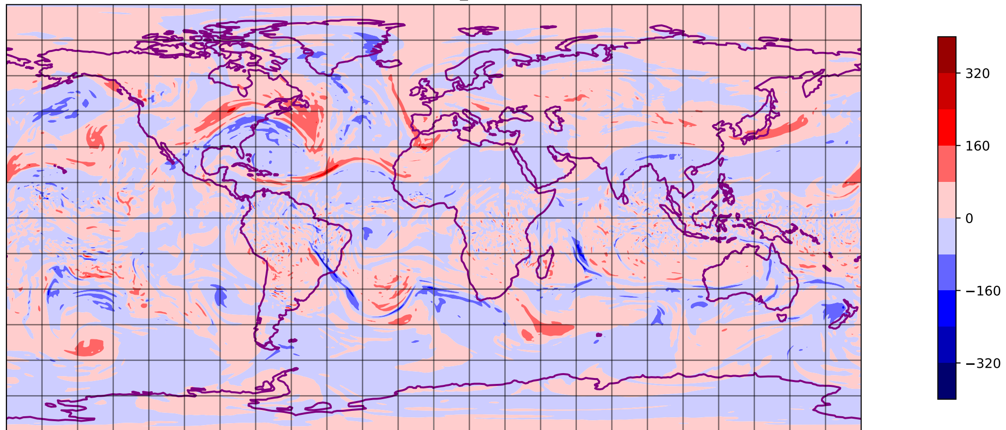
VOR 200 hPa 21121978_00 h - ERA5 025
