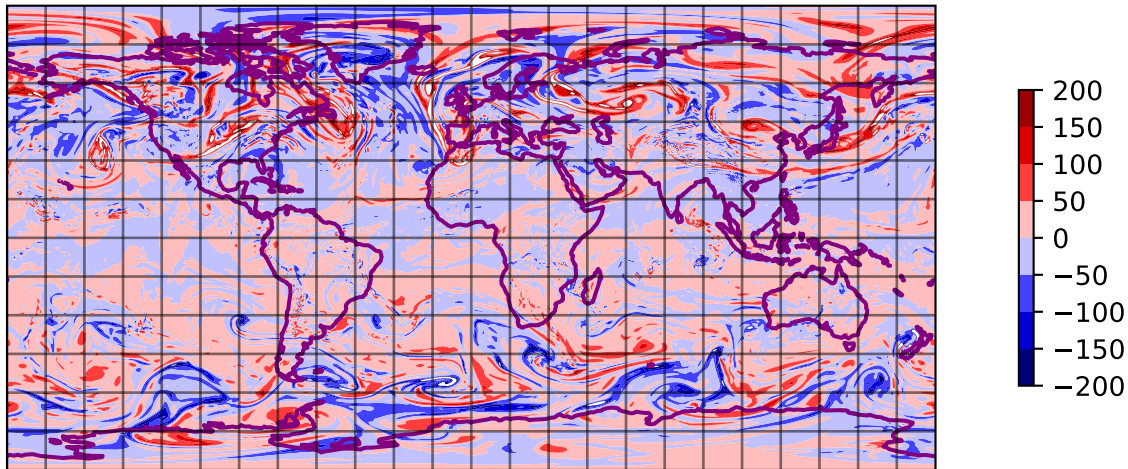
VOR 500 hPa 21121978_00 h - ERA5 025
