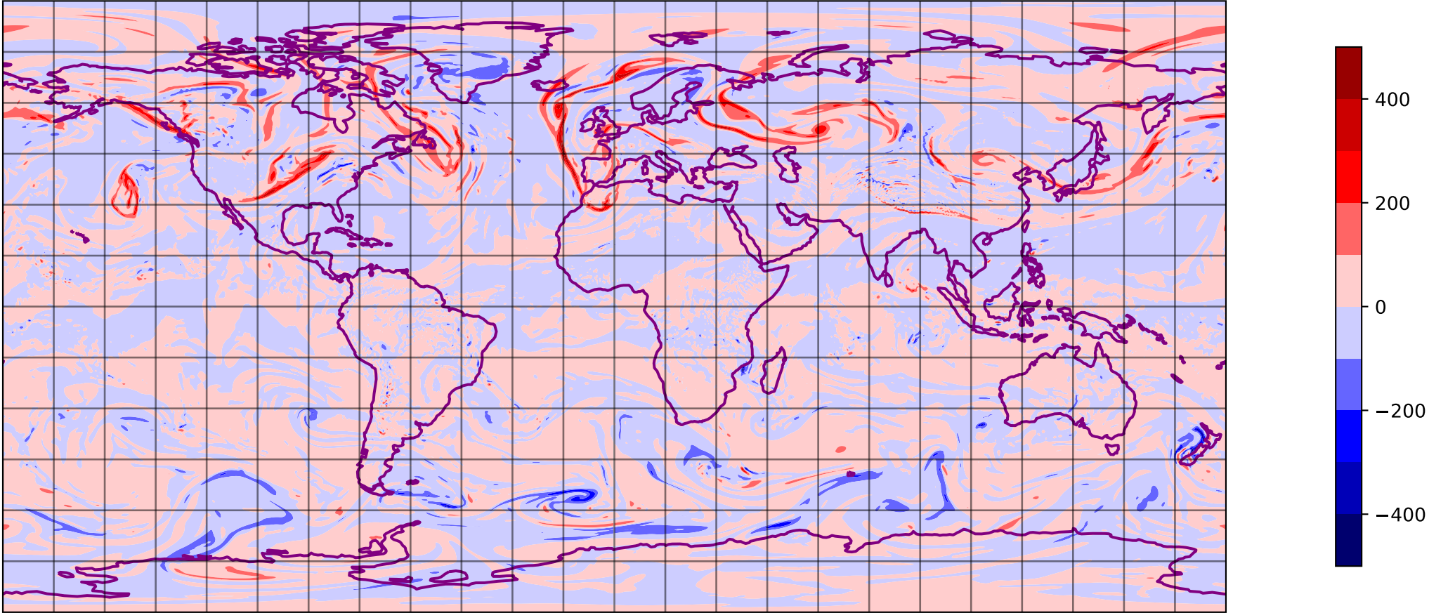
VOR 500 hPa 21121978_00 h - ERA5 025
