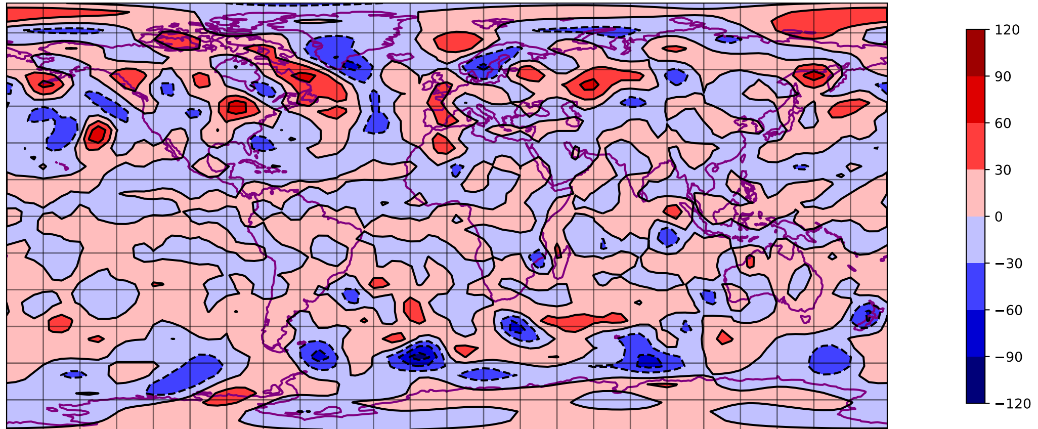
SQG vor 800 hpa 0000h - T031 expid=101
