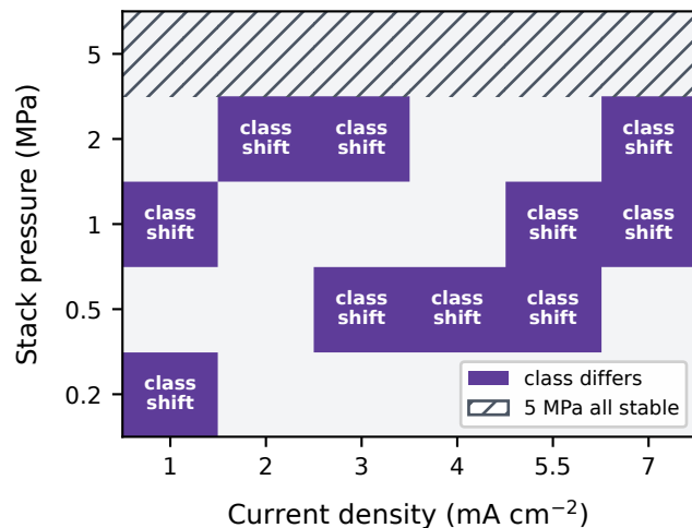
(d) Classification leverage
