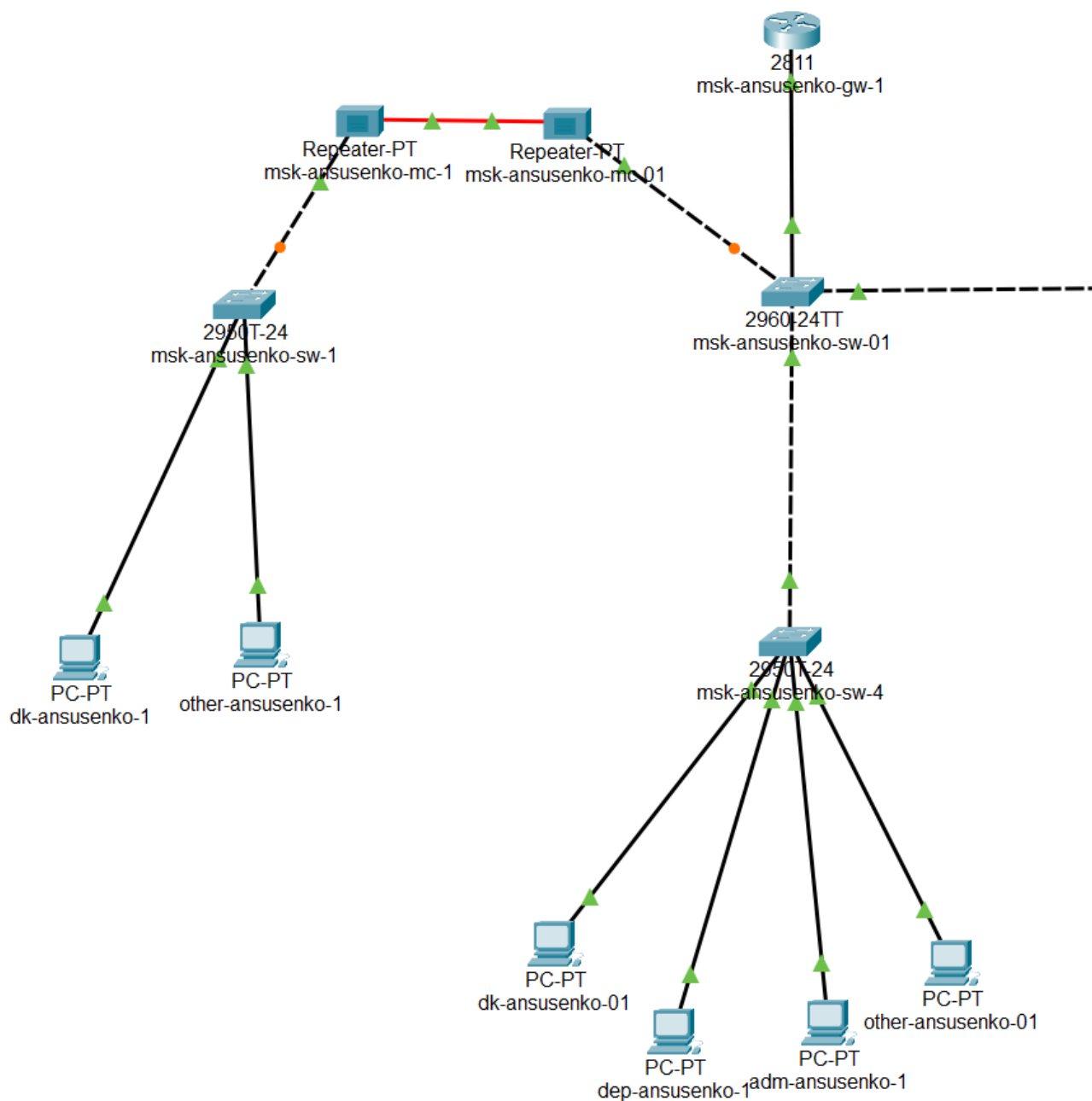
Рис. 10: Новый вид схемы (отрезок с повторителями)
