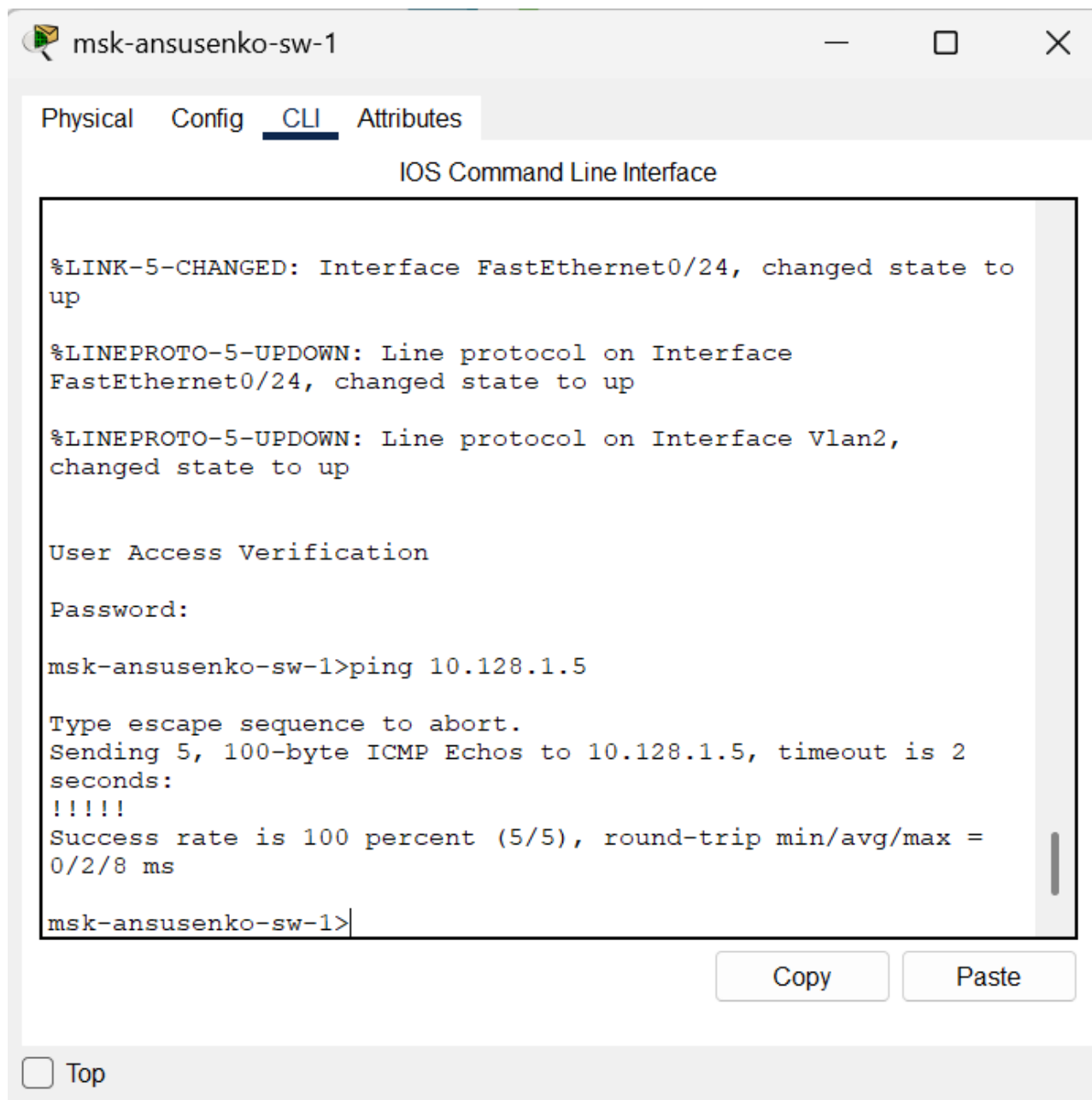
Рис. 13: Ping от ansusenko-p к ansusenko.
