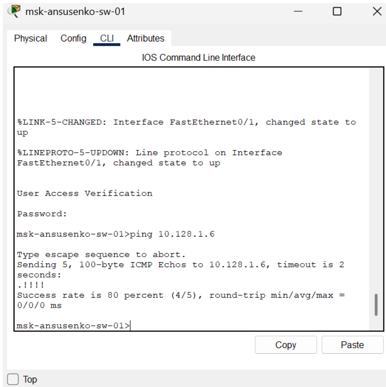
Рис. 12: Ping от ansusenko к ansusenko-p.
